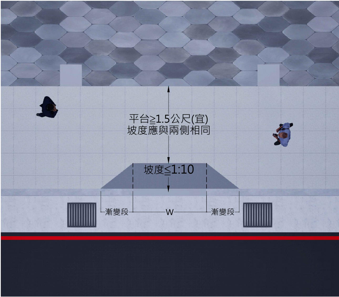
車行穿越道平面圖 註:車道寬度W依照核定尺寸施作 單位:cm
