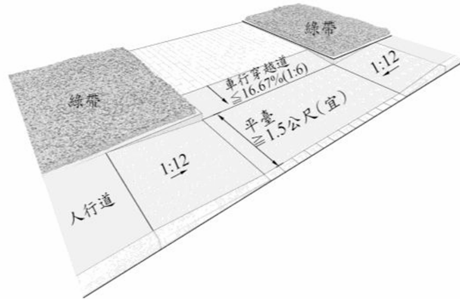
斜視圖
