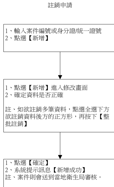
圖27 報備支援註銷操作流程
