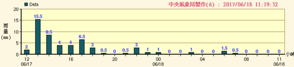
彌陀 過去24小時時雨量 2017-06-17 12:00 ~ 2017-06-18 11:00
