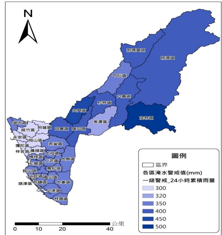
淹水警戒雨量-24小時
