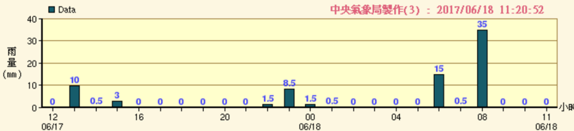
鳳山 過去24小時時雨量 2017-06-17 12:00 ~ 2017-06-18 11:00
