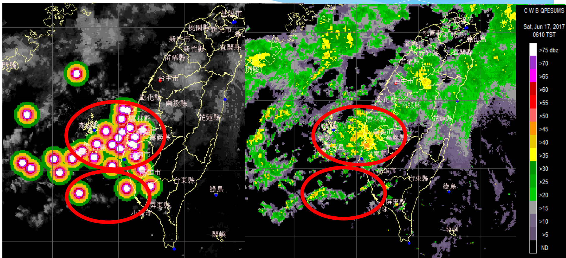
6月18日11:10對流胞分布圖
