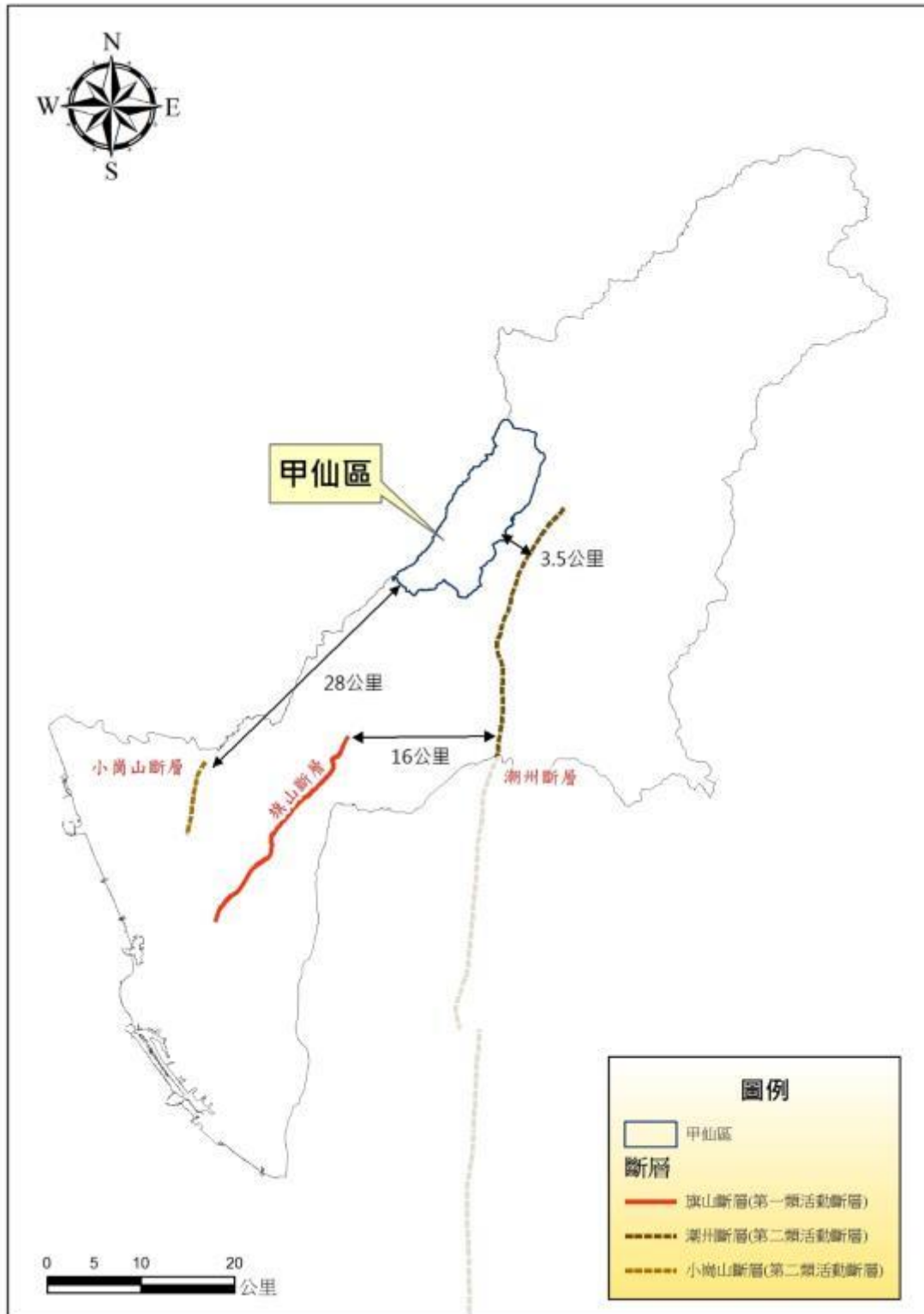
圖 13 甲仙區與高雄市斷層分布相對位置圖
