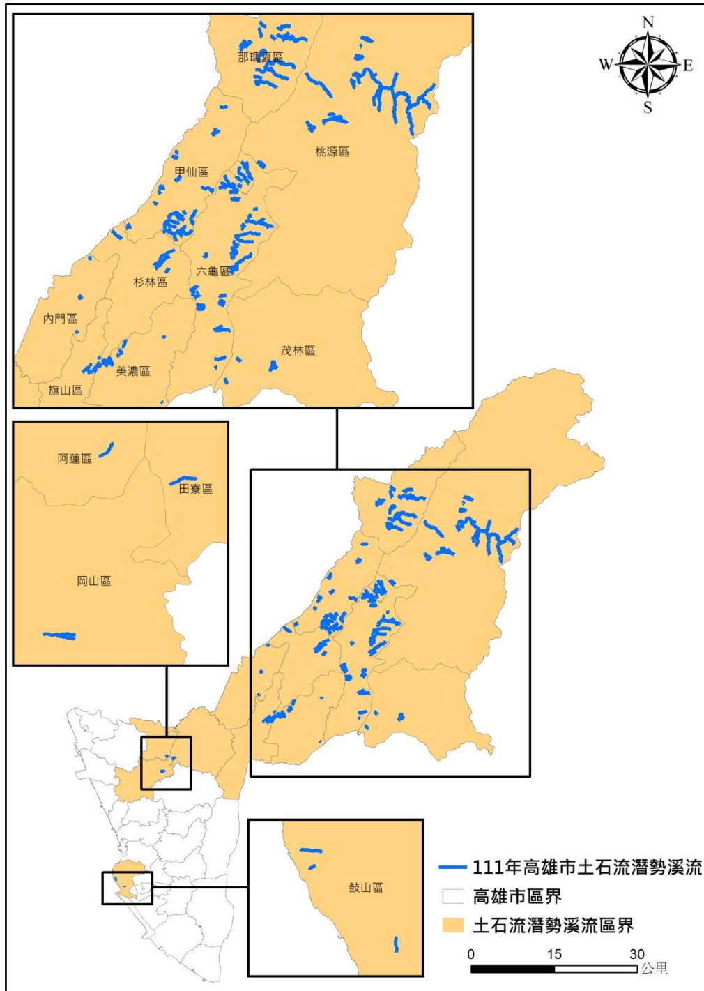
圖 8 高雄市土石流潛勢溪流分布圖
