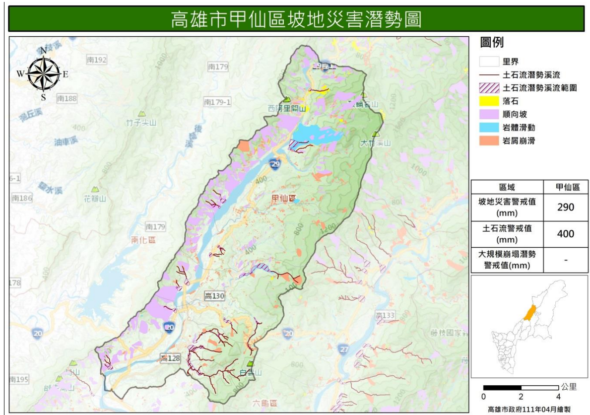
圖 9 甲仙區坡地災害潛勢分布圖
