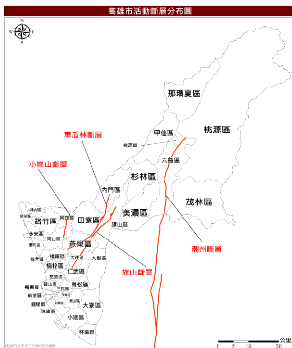
圖 10 高雄市境內與鄰近地區斷層分布圖
