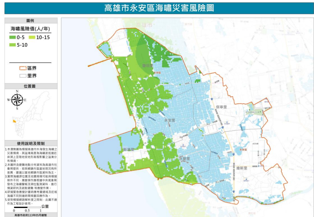
圖 27 永安區海嘯災害風險圖
