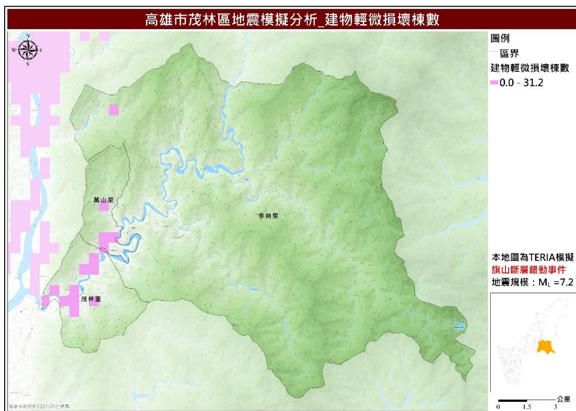
圖 13 茂林區旗山斷層錯動事件建物輕微損壞數推估圖
