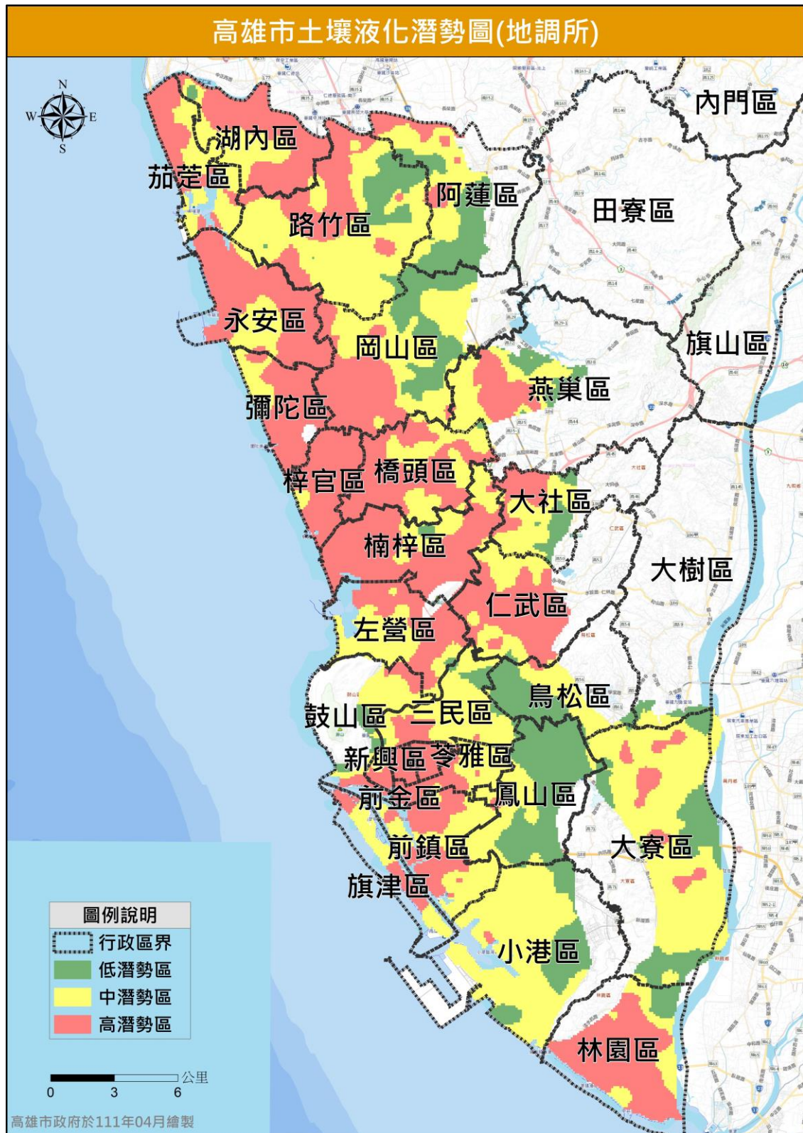
圖 20 高雄市土壤液化潛勢圖 (資料來源：經濟部中央地質調查所)
