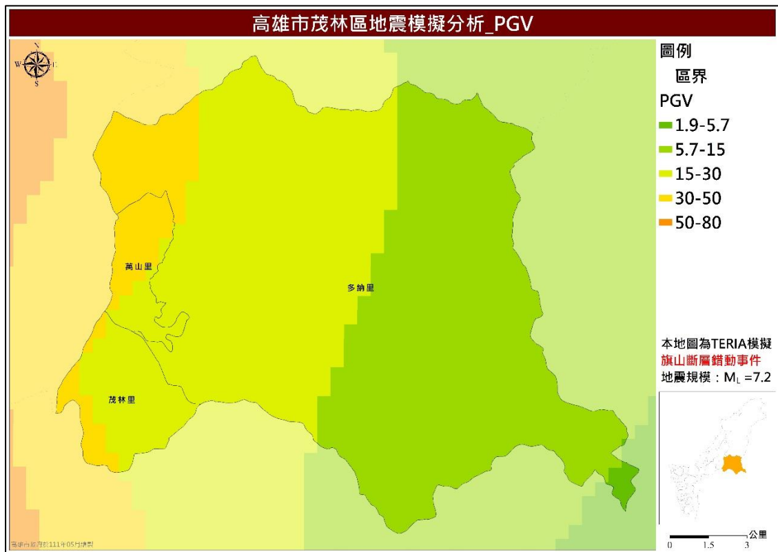
圖 8 茂林區旗山斷層錯動事件最大地表速度值(PGV)分布圖
