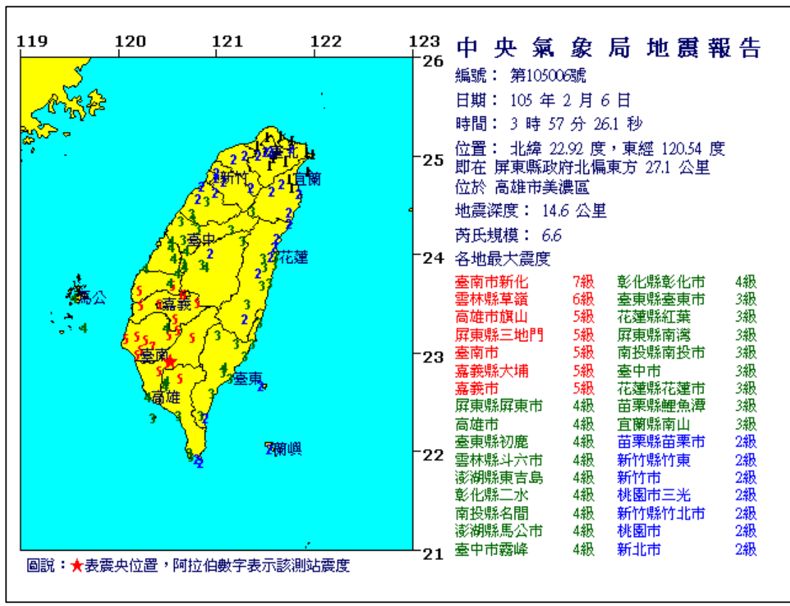
圖 19 第 105006 號高雄市美濃地震參數及各地震度分布
