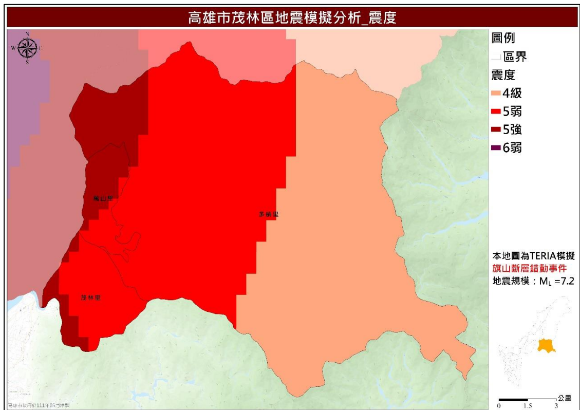
圖 9 茂林區旗山斷層錯動事件震度分布圖
