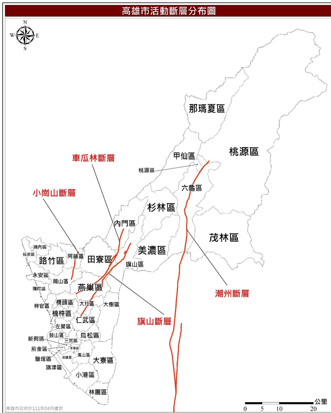
圖 6 高雄市境內與鄰近地區斷層分布圖
