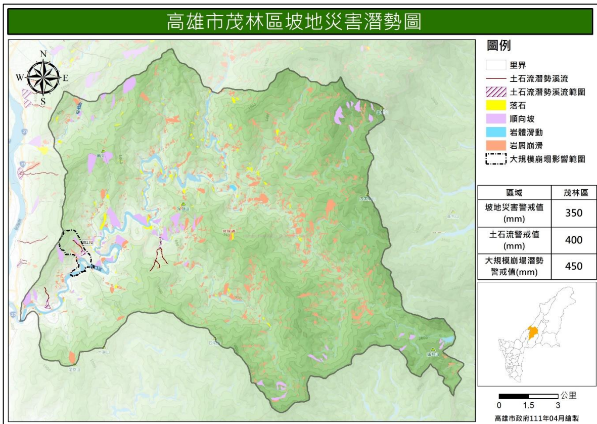
圖 5 茂林區坡地潛勢分布圖
