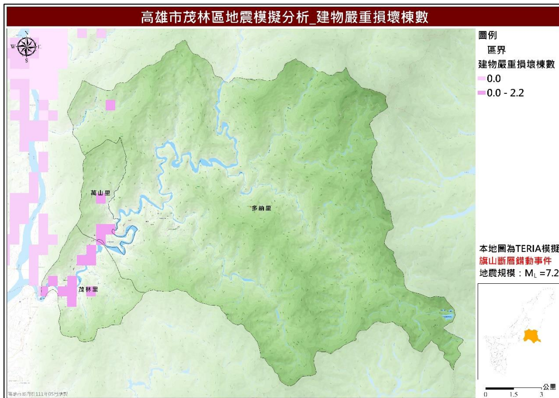
圖 11 茂林區旗山斷層錯動事件建物嚴重損壞棟數推估圖
