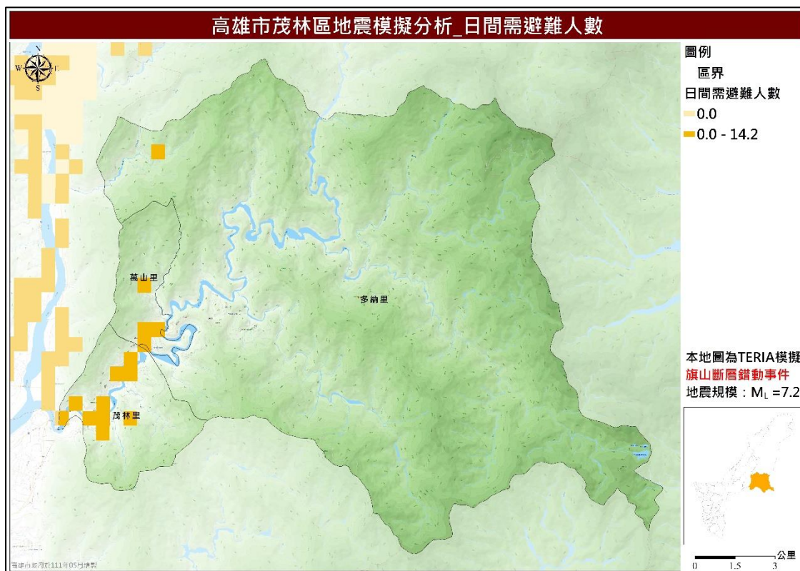
圖 17 茂林區旗山斷層錯動事件日間需避難人數推估圖
