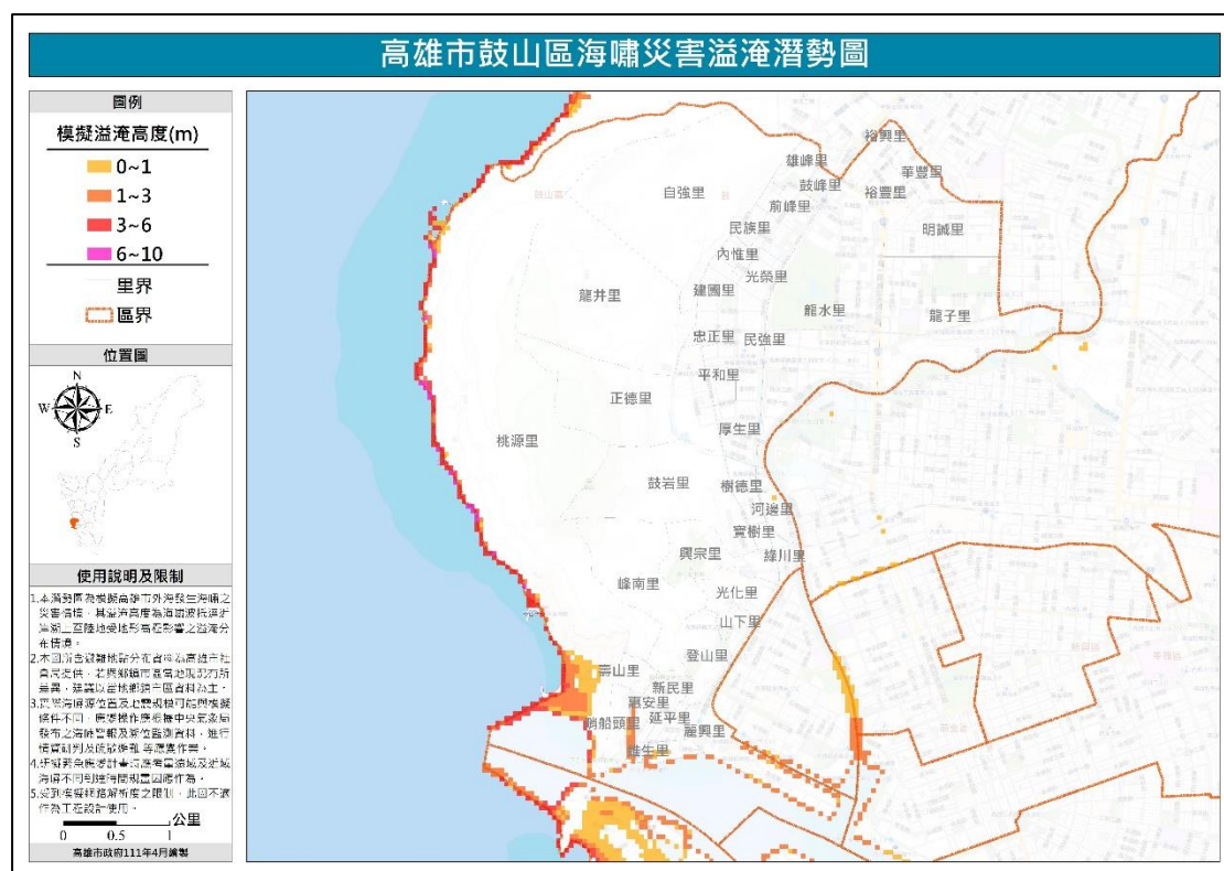
圖 28 鼓山區海嘯災害溢淹潛勢圖
