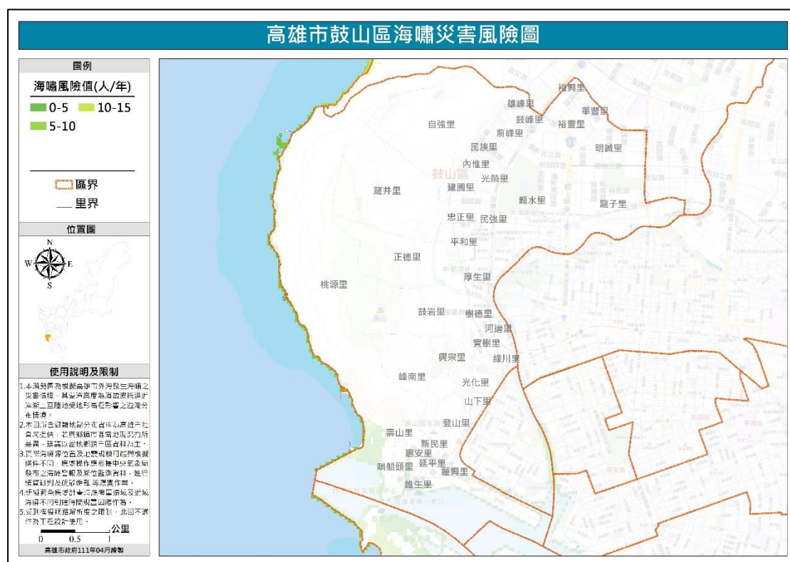
圖 29 鼓山區海嘯災害風險圖
