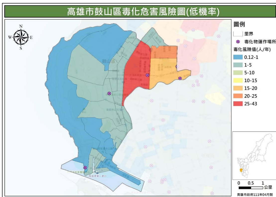
圖 31 鼓山區毒性化學物質災害危害風險潛勢圖（低機率）
