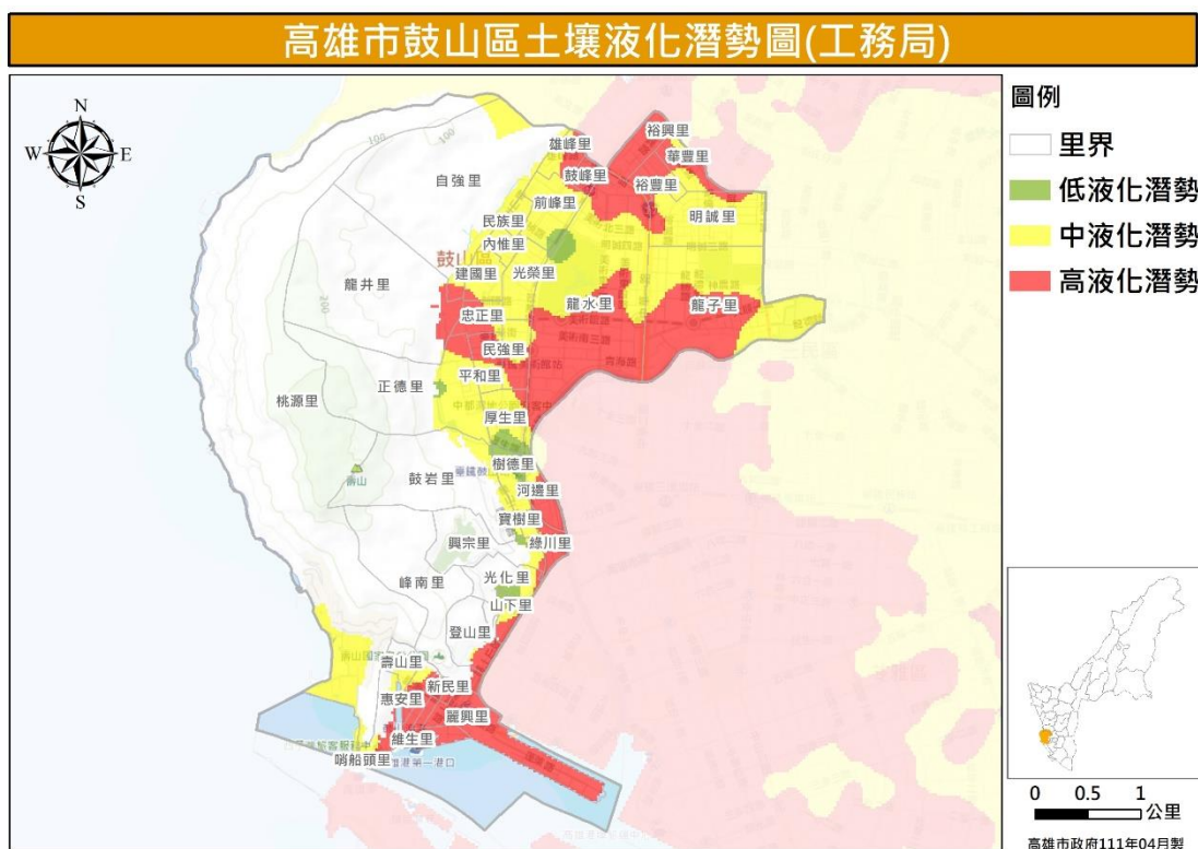
圖 27 鼓山區土壤液化潛勢圖（資料來源：高雄市政府工務局）
