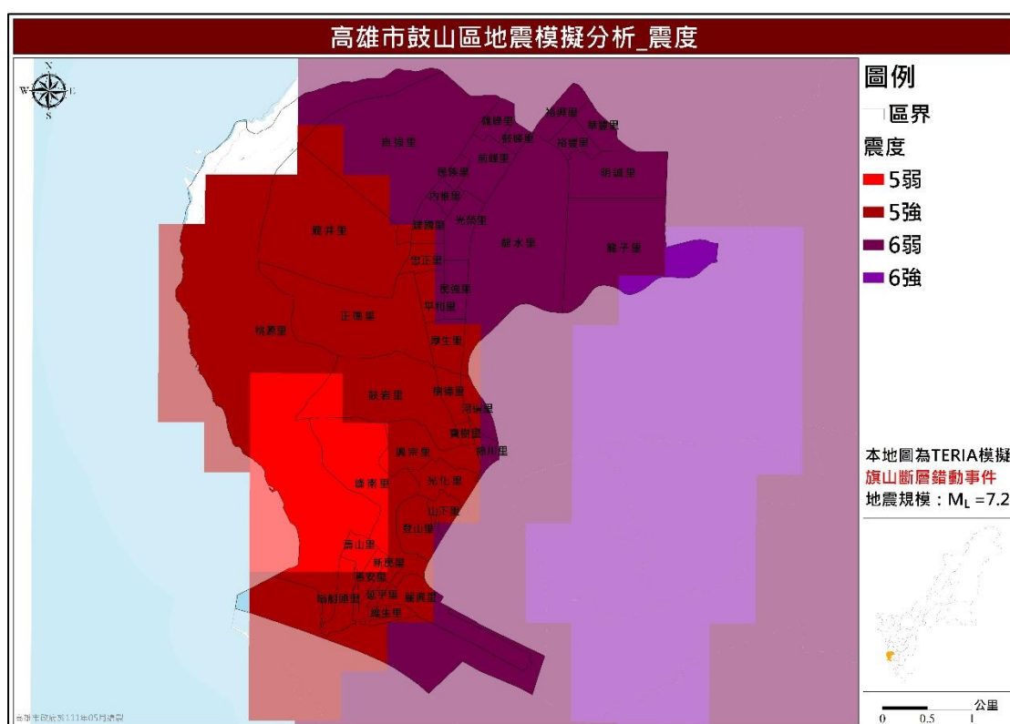
圖 15 旗山斷層錯動事件震度分布圖
