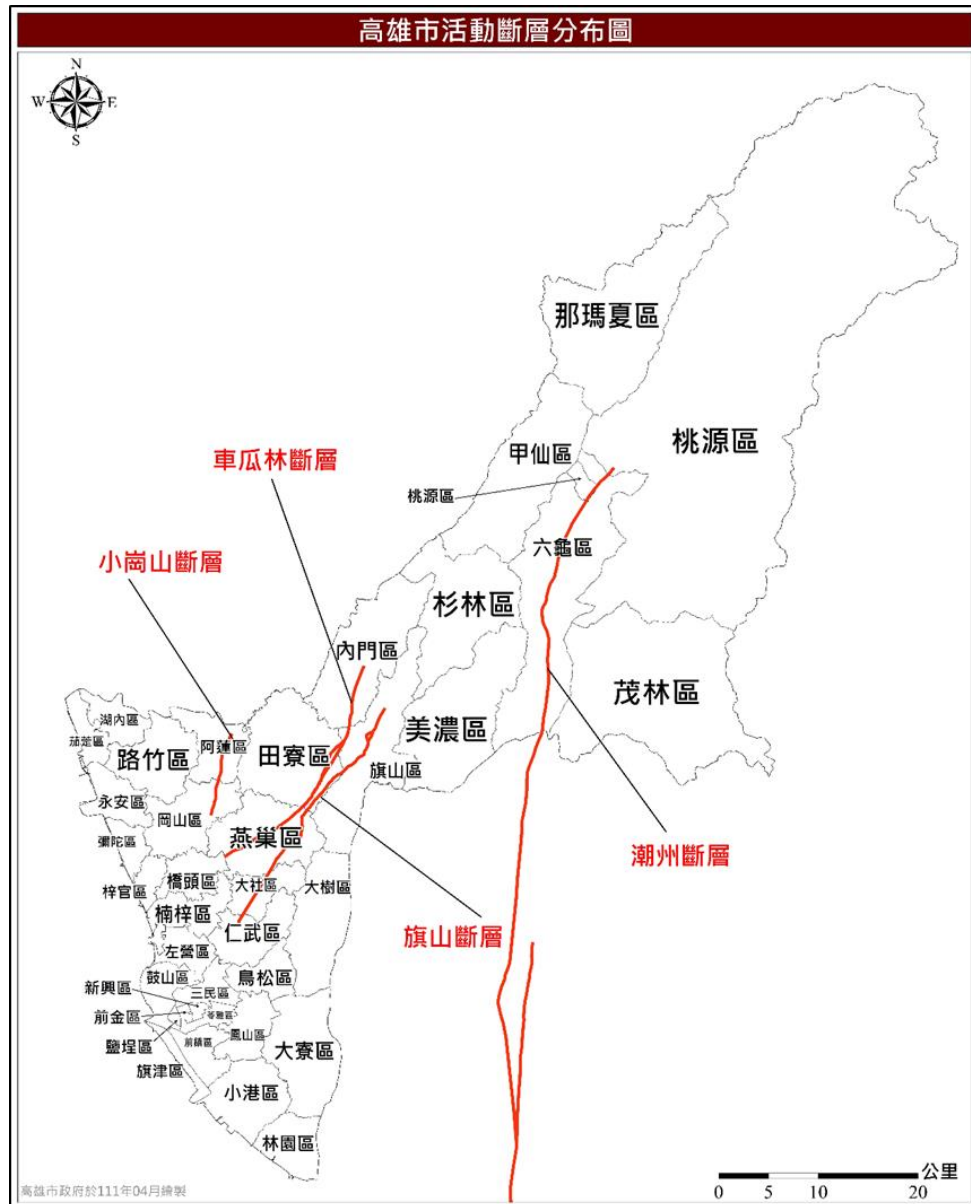
圖 12 高雄市境內與鄰近地區斷層分布圖
