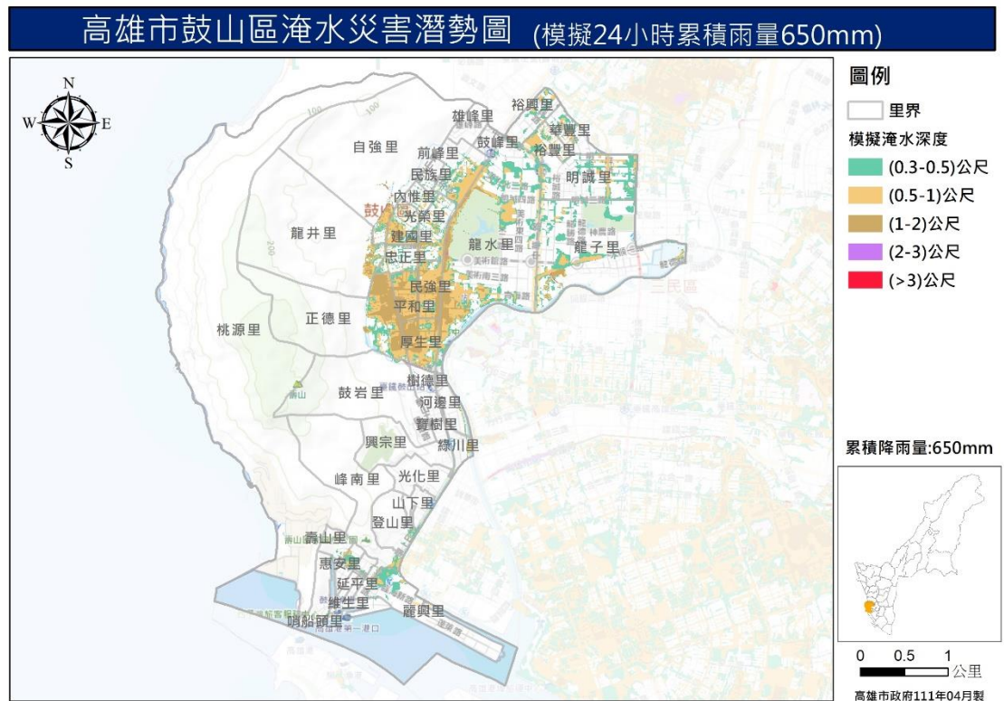
圖 7 鼓山區淹水災害潛勢圖（模擬 24 小時累積降雨量 650mm）
