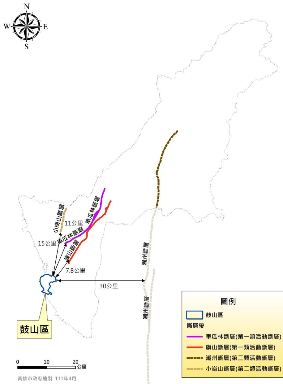
圖 13 鼓山區與高雄市斷層分布相對位置圖
