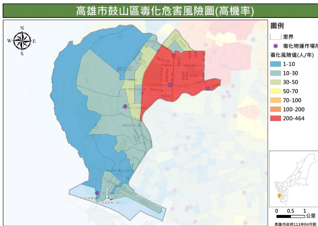
圖 32 鼓山區毒性化學物質災害危害風險潛勢圖（高機率）
