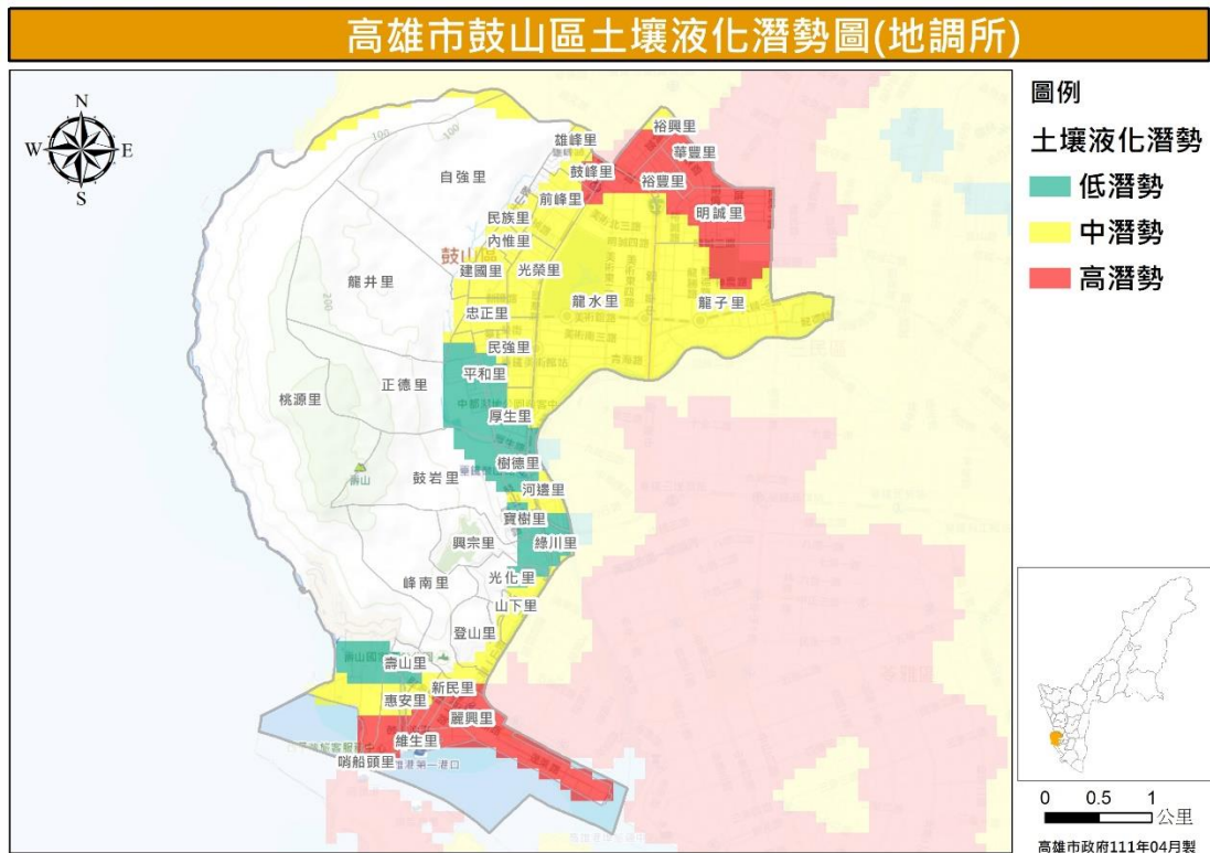
圖 26 鼓山區土壤液化潛勢圖（資料來源：經濟部中央地質調查所）
