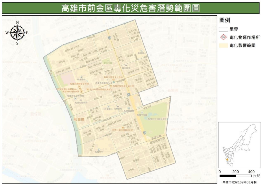
圖 30 前金區毒性化學物質災害危害潛勢範圍圖
