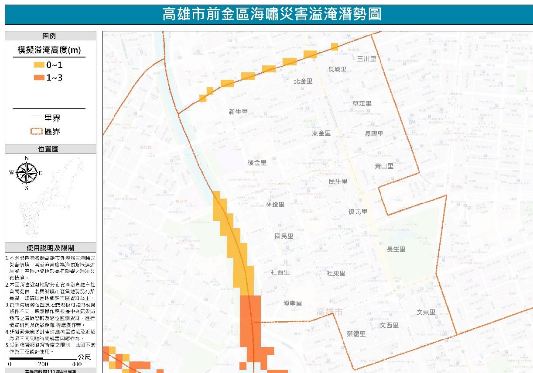
圖 28 前金區海嘯災害潛勢圖
