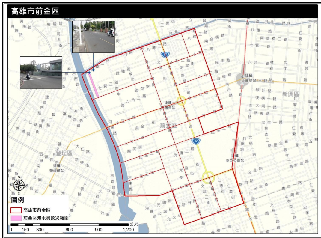
圖 9 前金區淹水易致災區域分布圖
