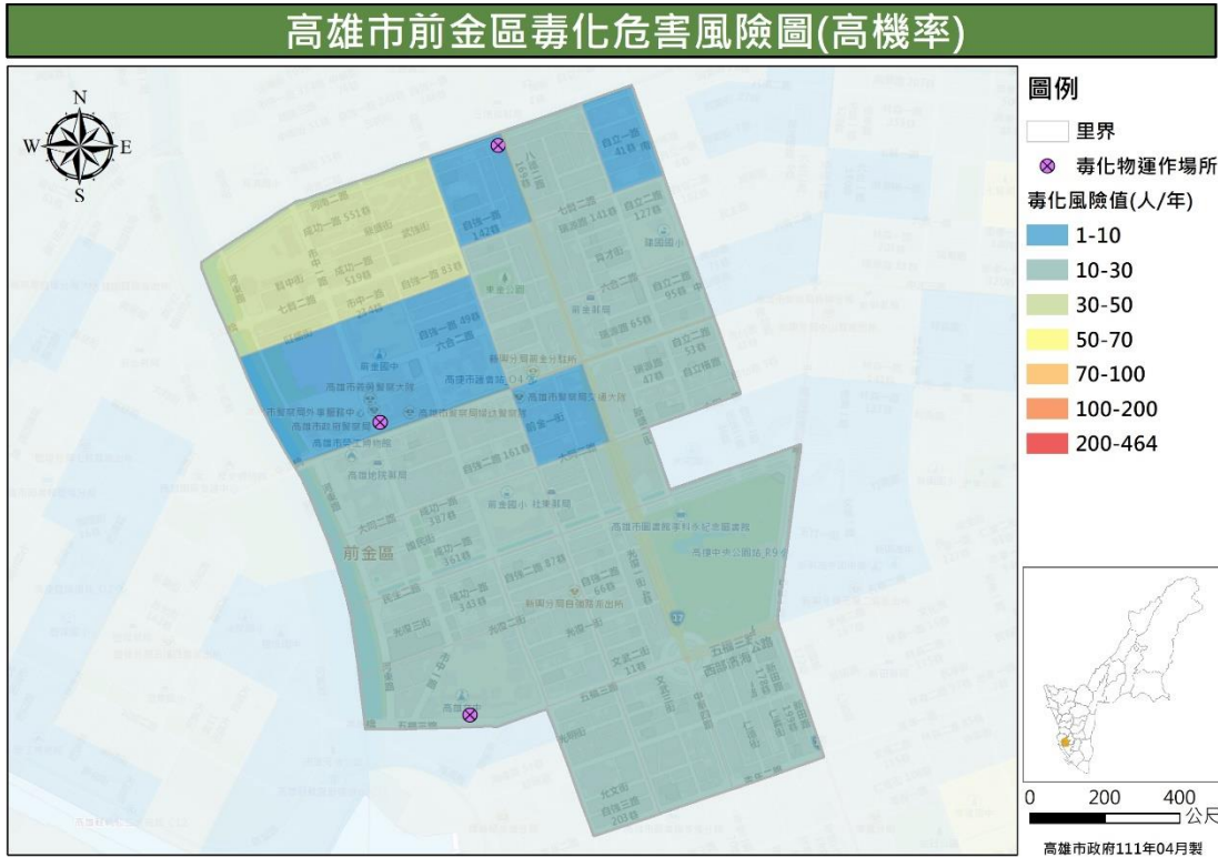
圖 31 前金區毒性化學物質災害危害風險潛勢圖（高機率）
