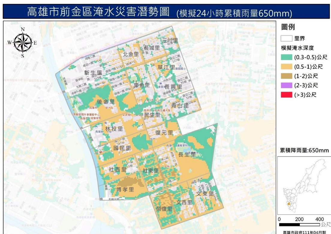
圖 6 前金區淹水災害潛勢圖 (模擬 24 小時累積降雨量 650mm)
