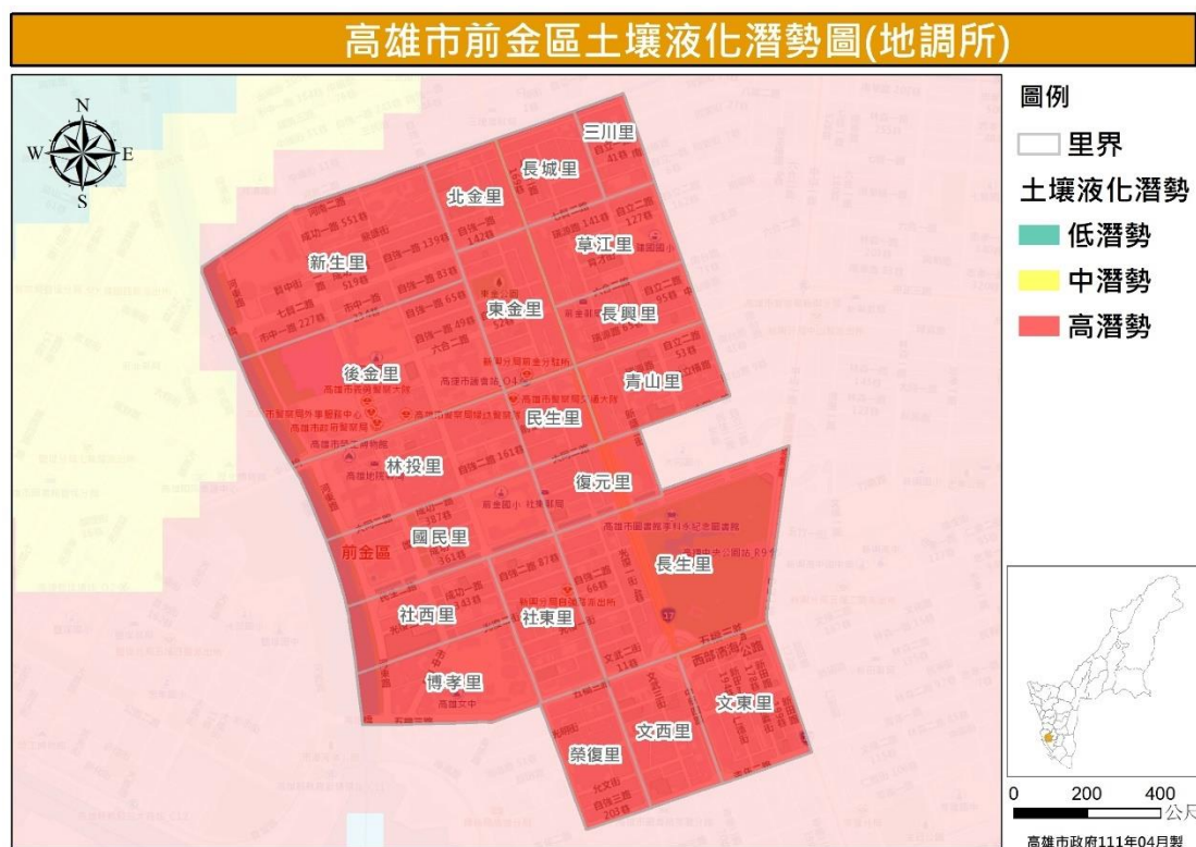
圖 26 前金區土壤液化潛勢圖（資料來源：經濟部中央地質調查所）
