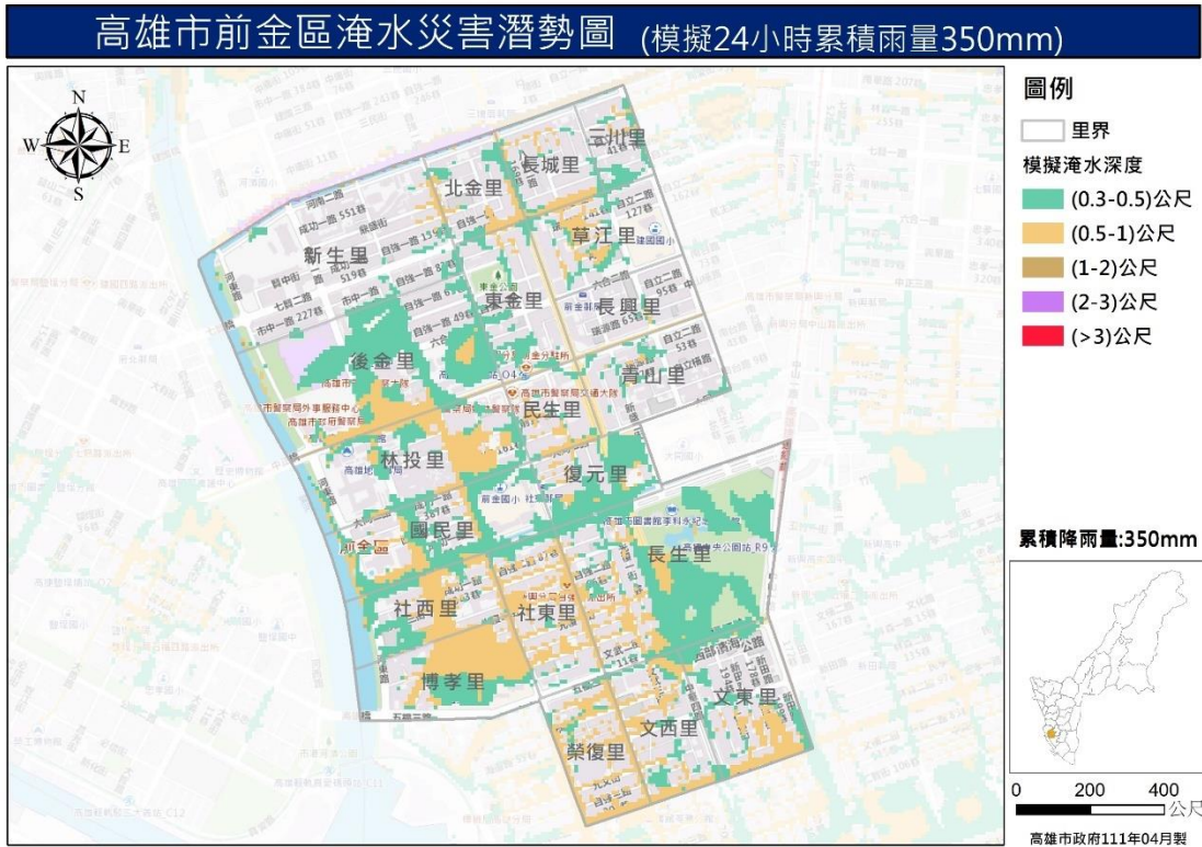
圖 8 前金區淹水災害潛勢圖 (模擬 24 小時累積降雨量 350mm)
