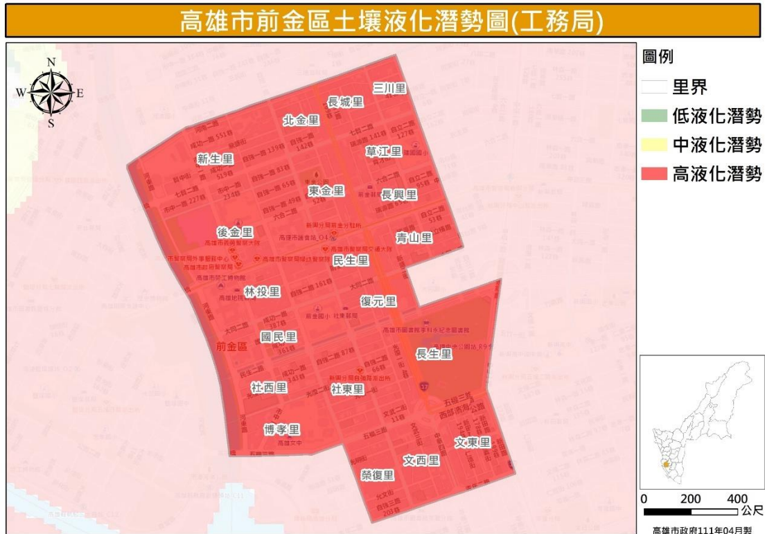
圖 27 前金區土壤液化潛勢圖（資料來源：高雄市政府工務局）
