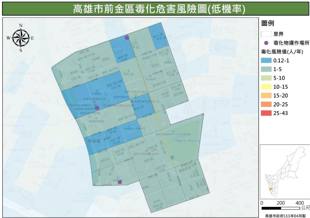
圖 32 前金區毒性化學物質災害危害風險潛勢圖（低機率）
