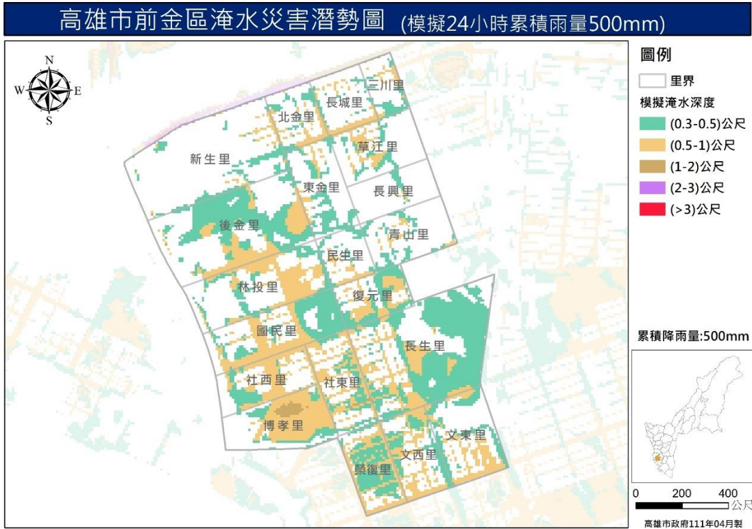
圖 7 前金區淹水災害潛勢圖 (模擬 24 小時累積降雨量 500mm)
