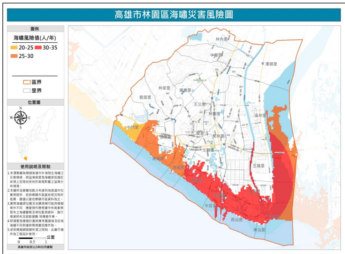
圖 27 林園區海嘯災害風險圖
