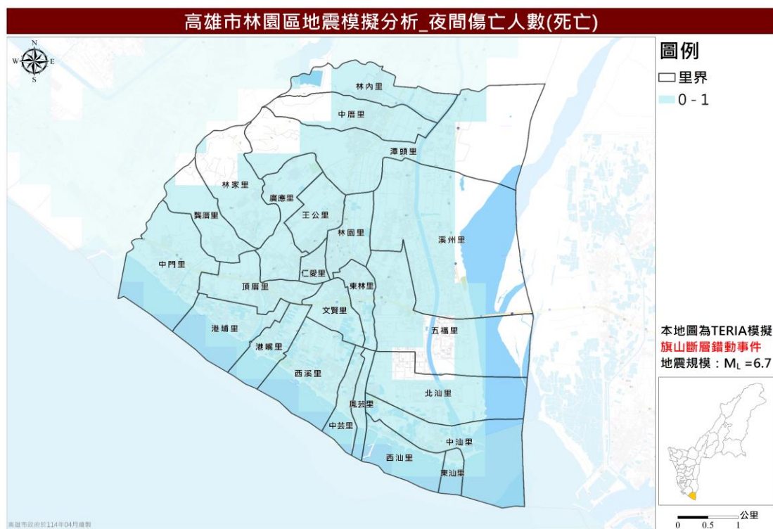
圖 19 旗山斷層錯動事件夜間死亡人數推估圖
