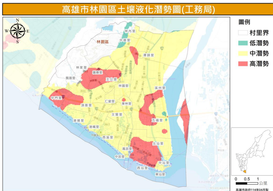
圖 25 林園區土壤液化潛勢圖（資料來源：高雄市政府工務局）
