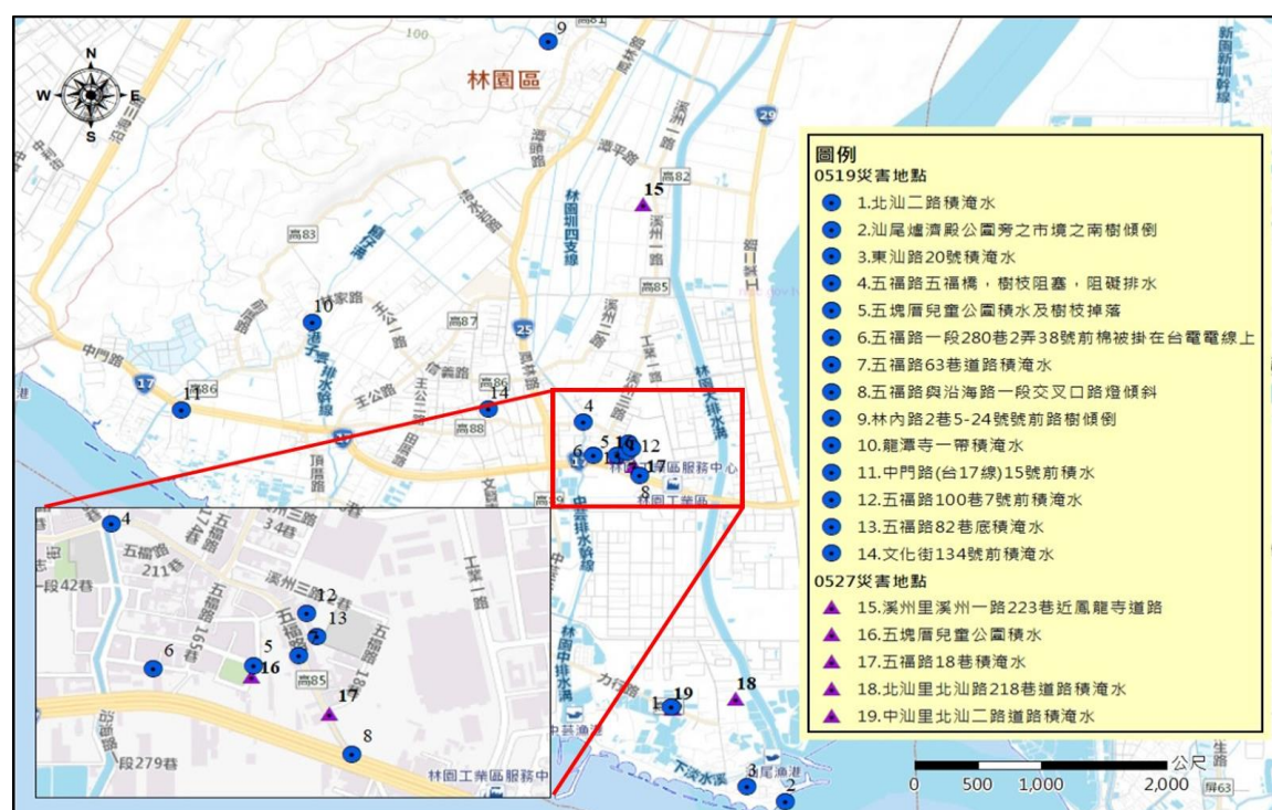
圖 8 林園區淹水易致災區域分布圖
