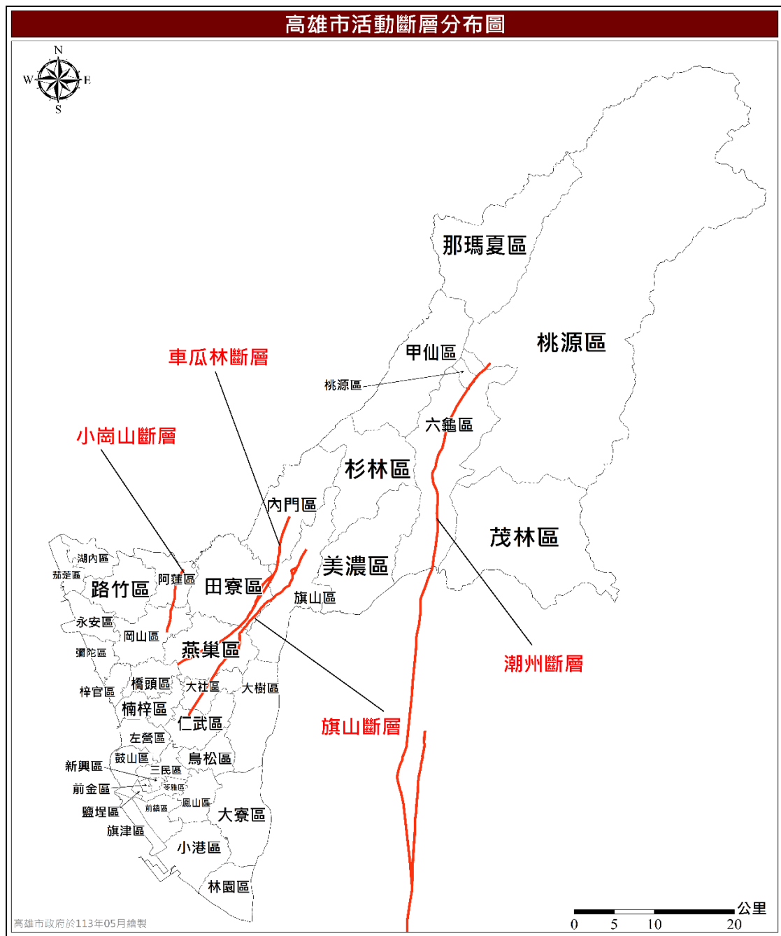
圖 10 高雄市境內與鄰近地區斷層分布圖
