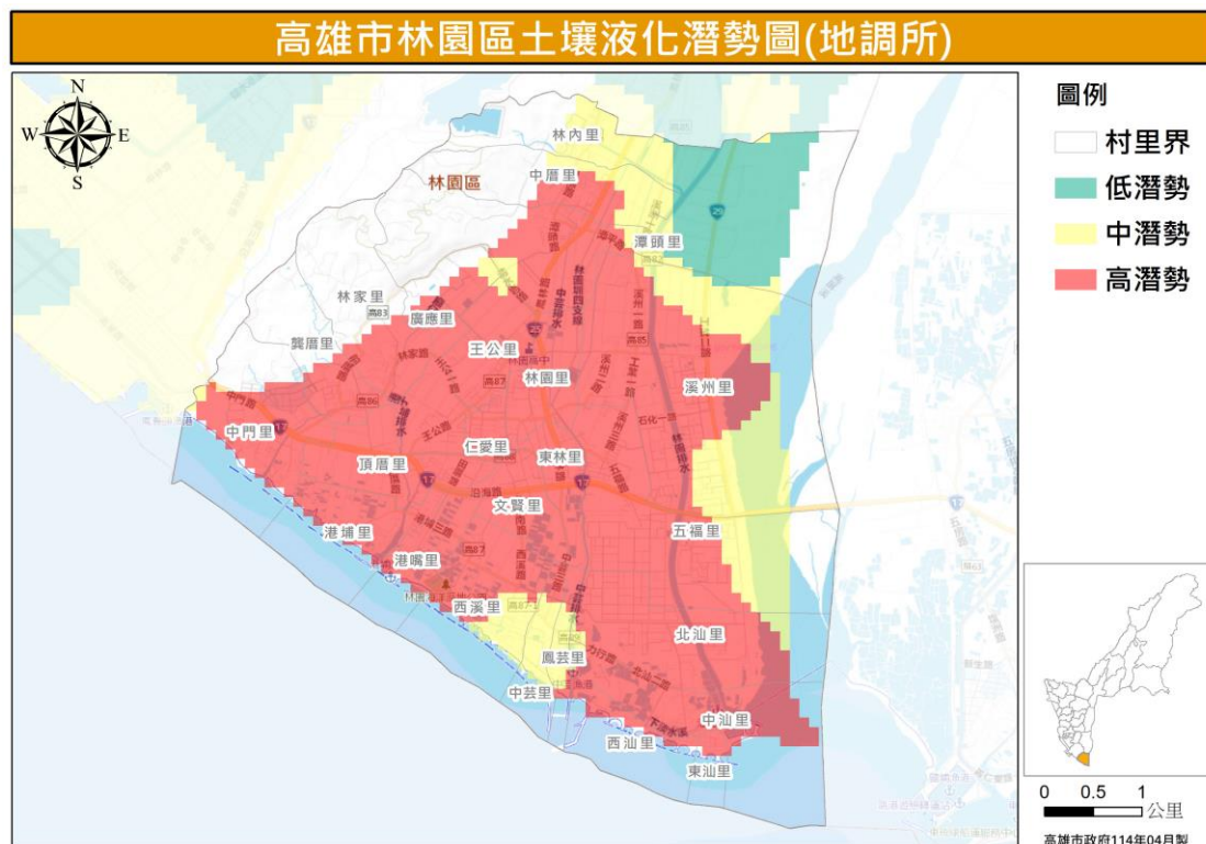
圖 24 林園區土壤液化潛勢圖（資料來源：地質調查及礦業管理中心）
