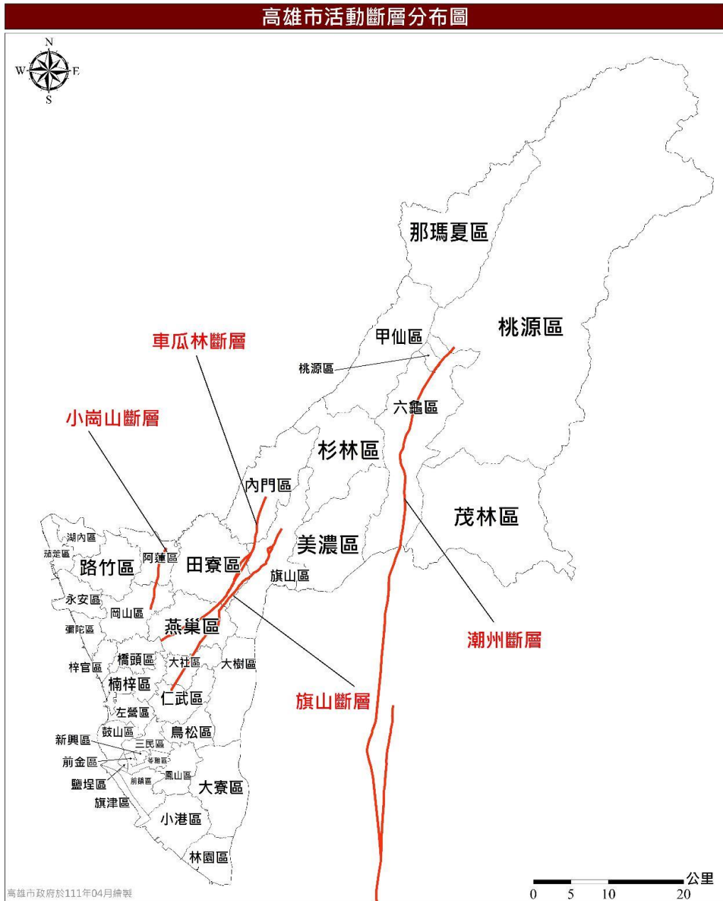
圖 11 高雄市境內與鄰近地區斷層分布圖
