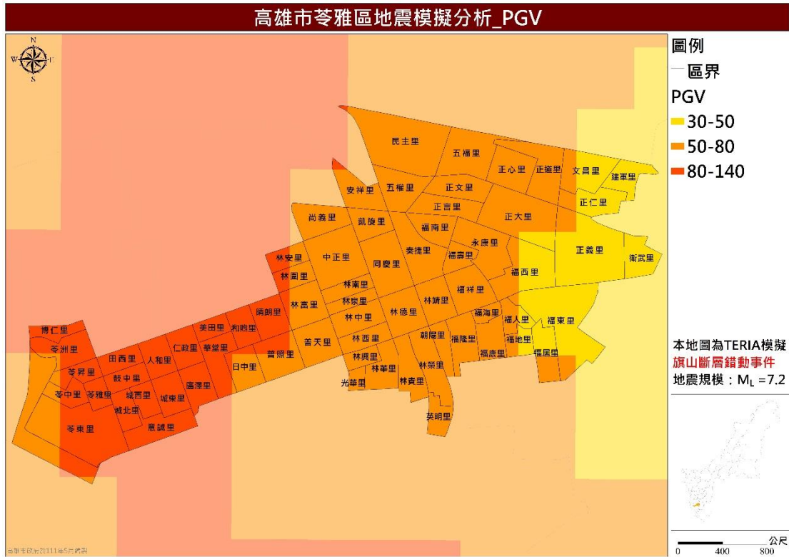
圖 12 旗山斷層錯動事件最大地表速度值 (PGA) 分布圖
