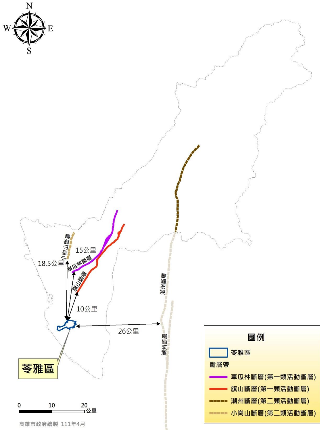
圖 11 苓雅區與高雄市斷層分布相對位置圖
