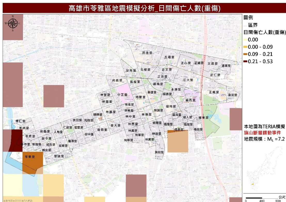
圖 23 旗山斷層錯動事件日間重傷人數推估圖
