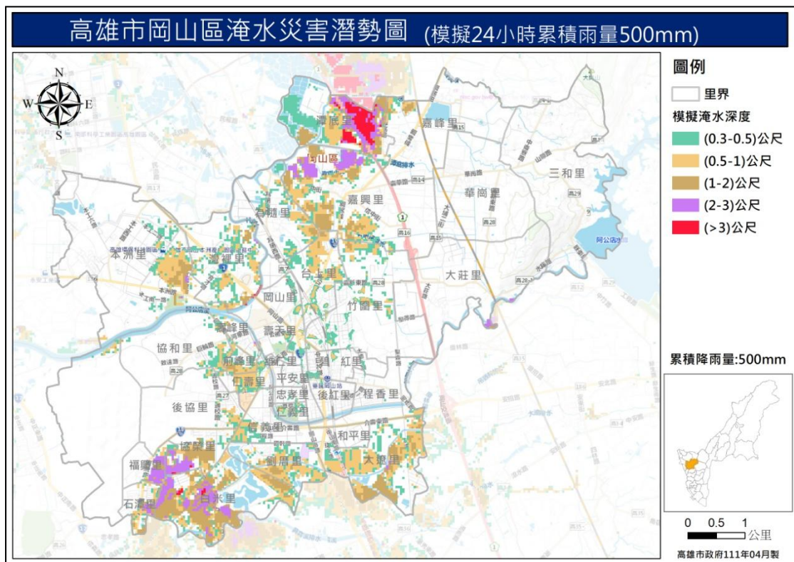
圖 7 岡山區淹水災害潛勢圖 (模擬 24 小時累積降雨量 500mm)
