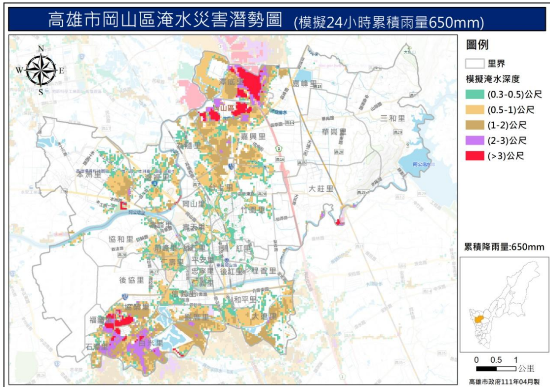
圖 6 岡山區淹水災害潛勢圖 (模擬 24 小時累積降雨量 650mm)
