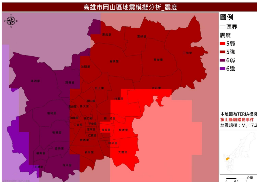
圖 14 旗山斷層錯動事件震度分佈圖
