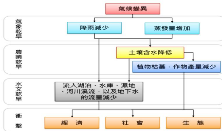
圖 23 不同乾旱類型之相互關係及衝擊
