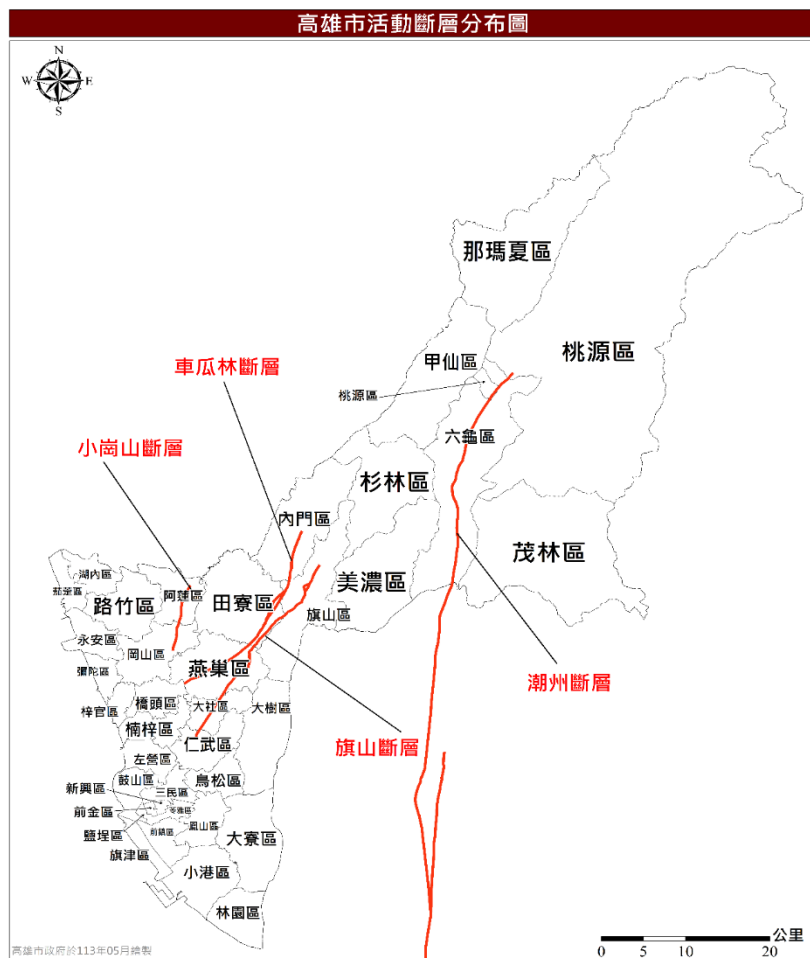
圖 6 高雄市境內與鄰近地區斷層分布圖
