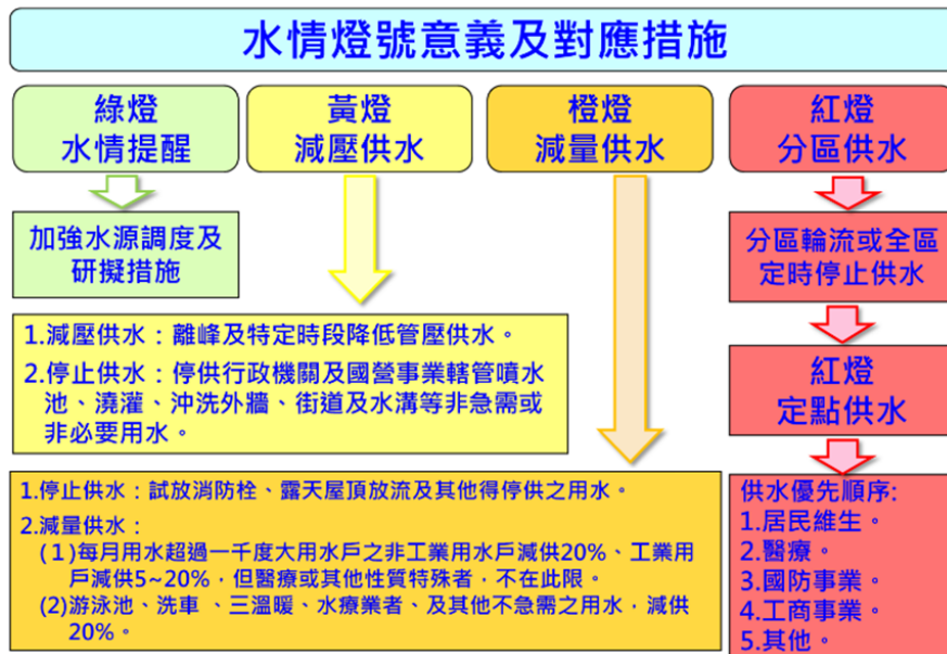
圖 22 水情燈號及各階段限水措施說明
