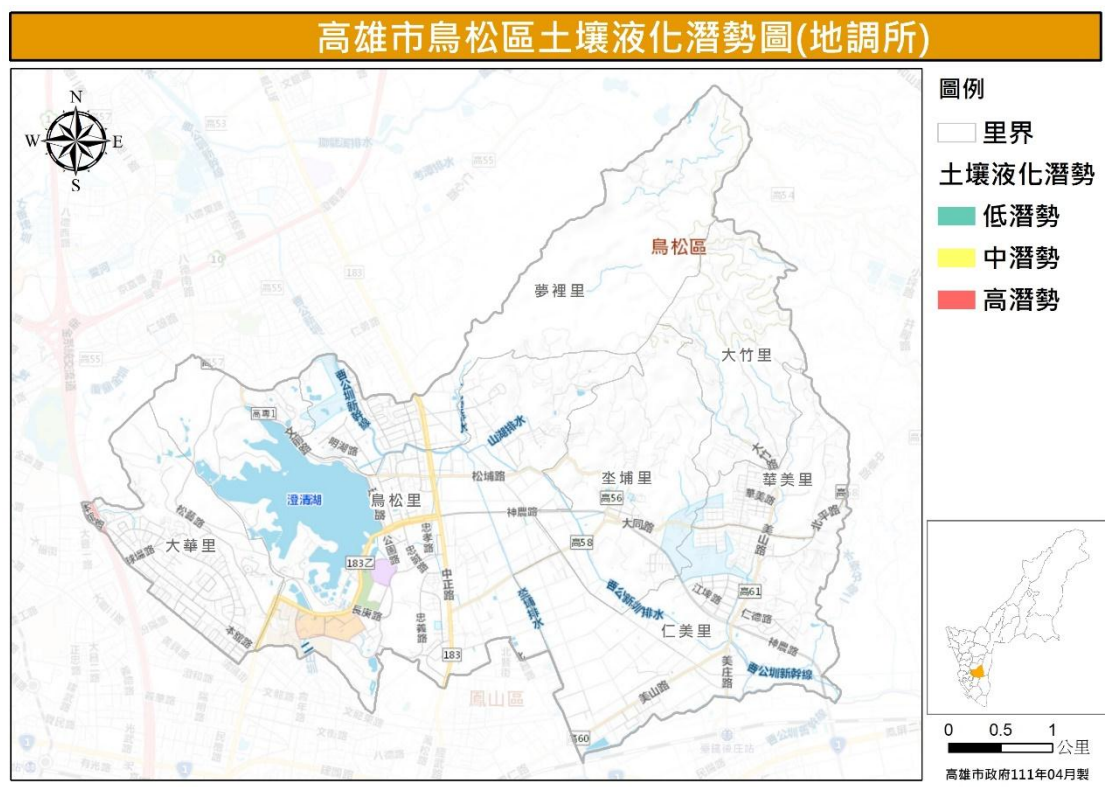
圖 25 鳥松區土壤液化潛勢圖 (資料來源：經濟部中央地質調查所)
