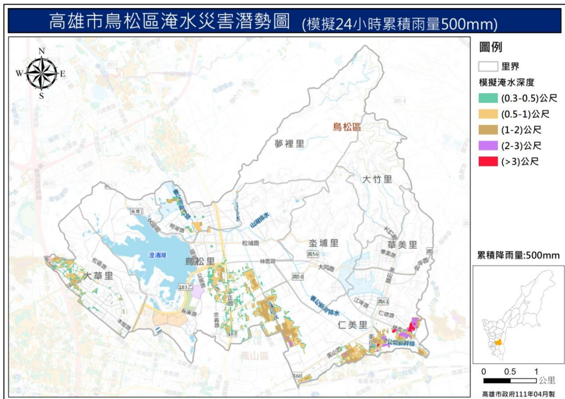
圖 6 鳥松區淹水救災潛勢圖 (模擬 24 小時累積降雨量 500mm)
