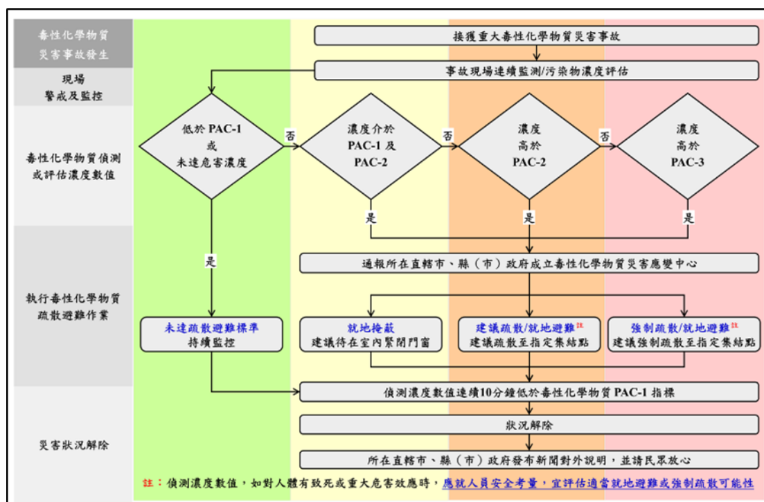
圖 30 毒性及關注化學物質災害疏散避難計畫作業流程圖
