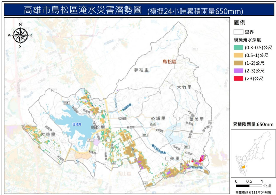
圖 5 鳥松區淹水救災潛勢圖 (模擬 24 小時累積降雨量 650mm)
