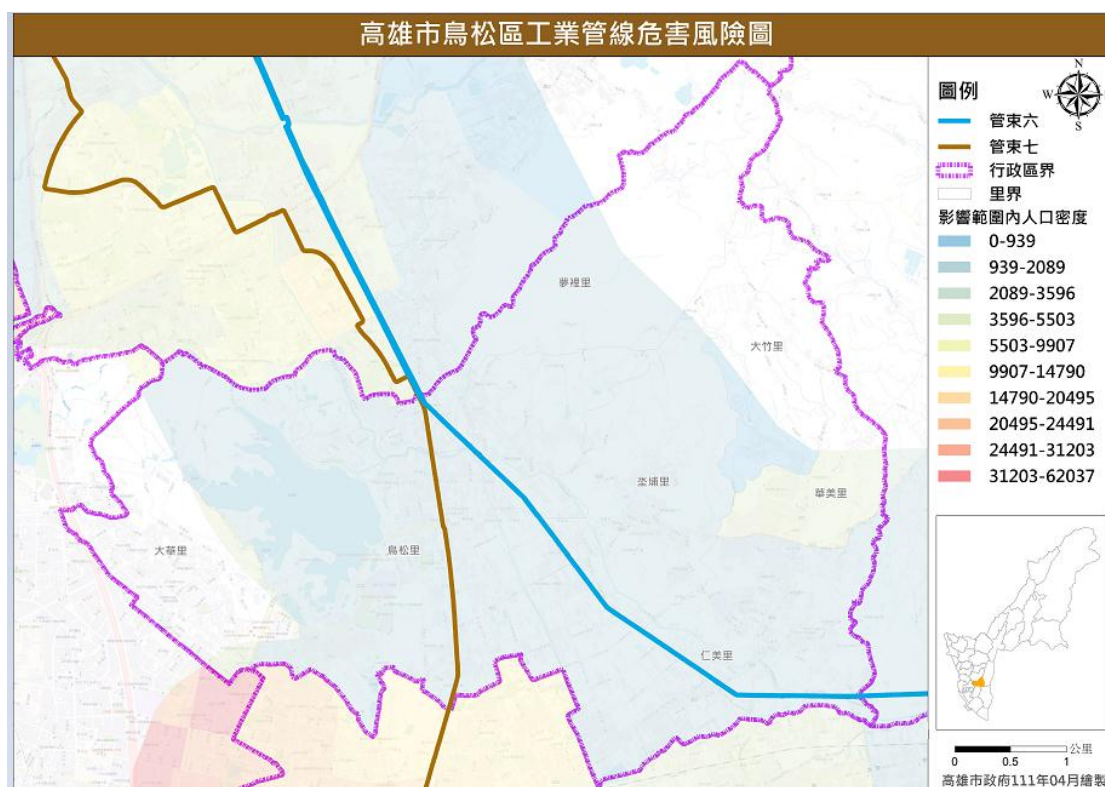
圖 31 烏松區工業管線分布圖
