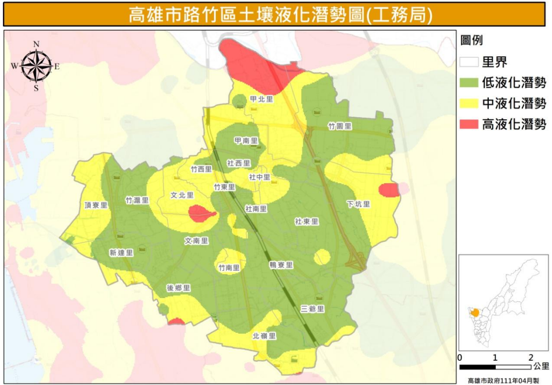
圖 24 路竹區土壤液化潛勢圖 (資料來源：高雄市政府工務局)
