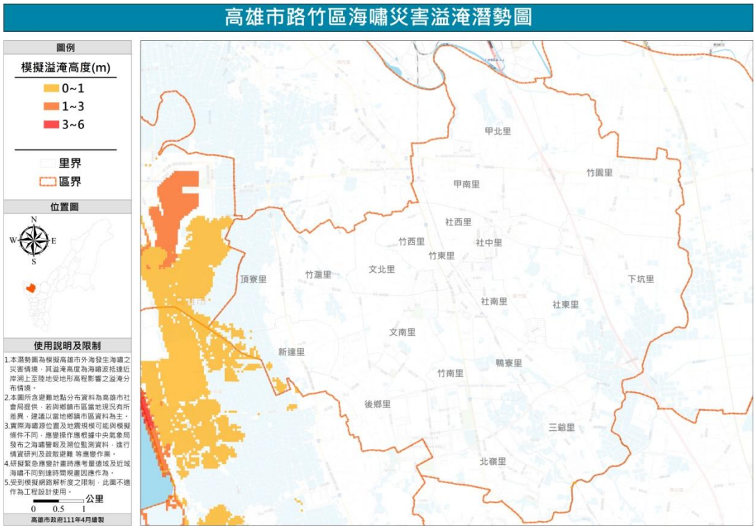
圖 25 路竹區海嘯災害溢淹潛勢圖
