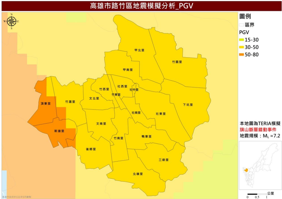
圖 11 旗山斷層錯動事件最大地表加速度 (PGA) 分布圖
