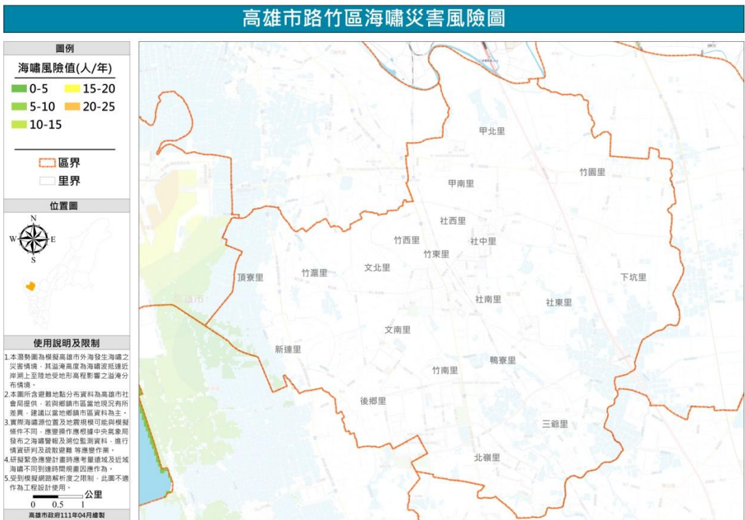
圖 26 路竹區海嘯災害風險圖
