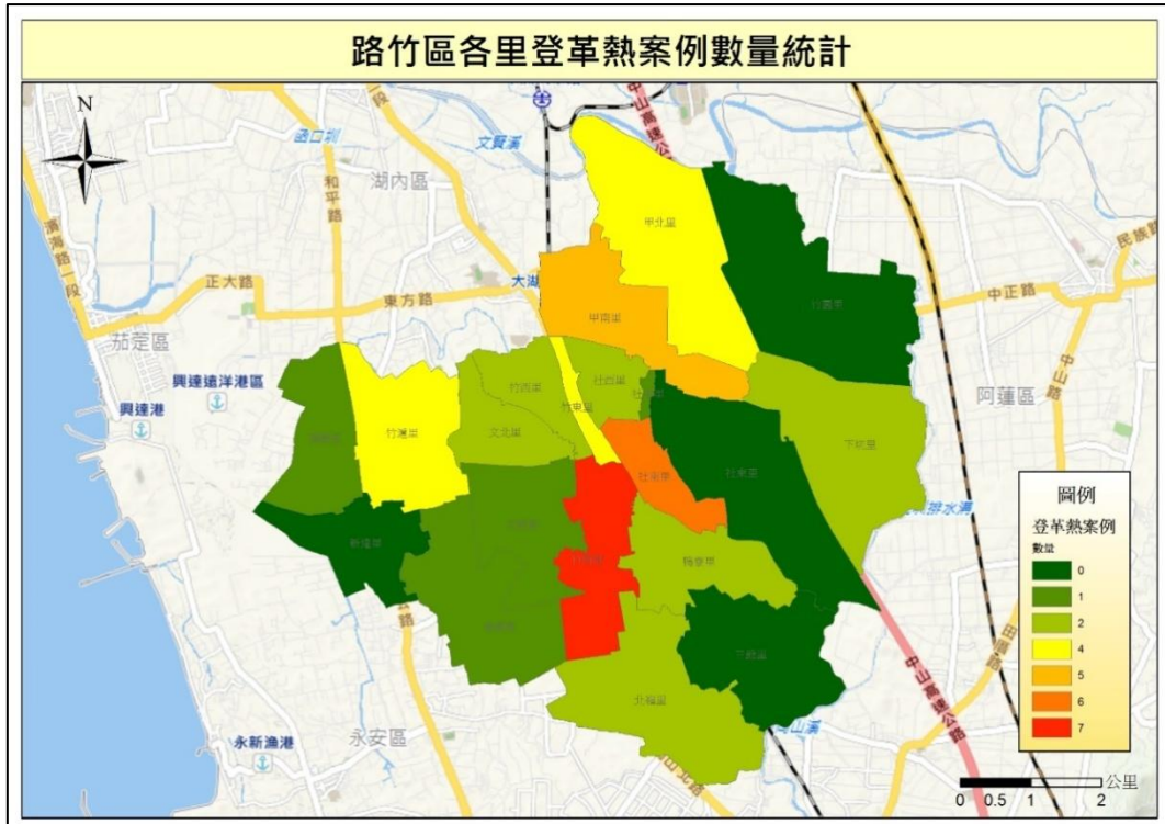
圖 32 路竹區登革熱確診病例分布圖(104 年)
