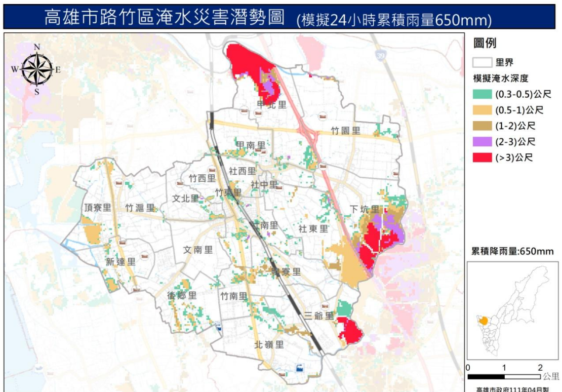
圖 5 路竹區淹水災害潛勢圖（模擬 24 小時累積降雨量 650mm）
