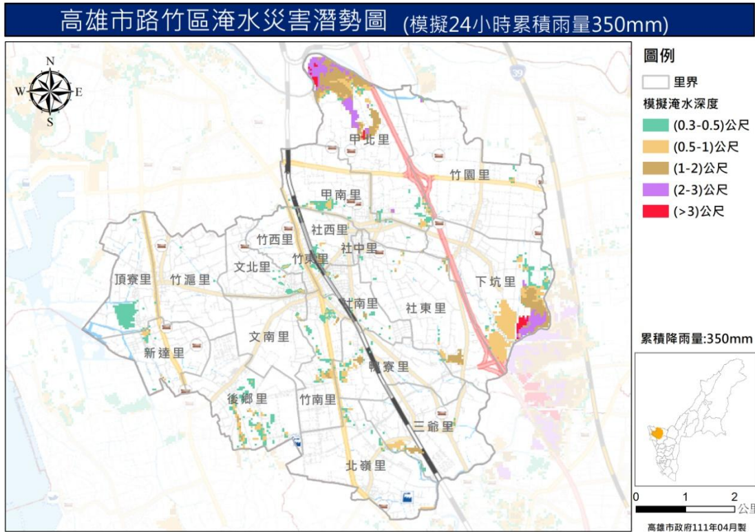
圖 7 路竹區淹水災害潛勢圖 (模擬 24 小時累積降雨量 350mm)
