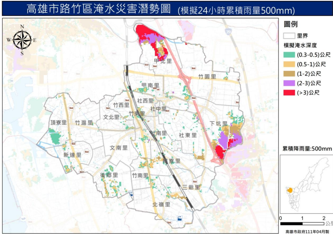
圖 6 路竹區淹水災害潛勢圖 (模擬 24 小時累積降雨量 500mm)
