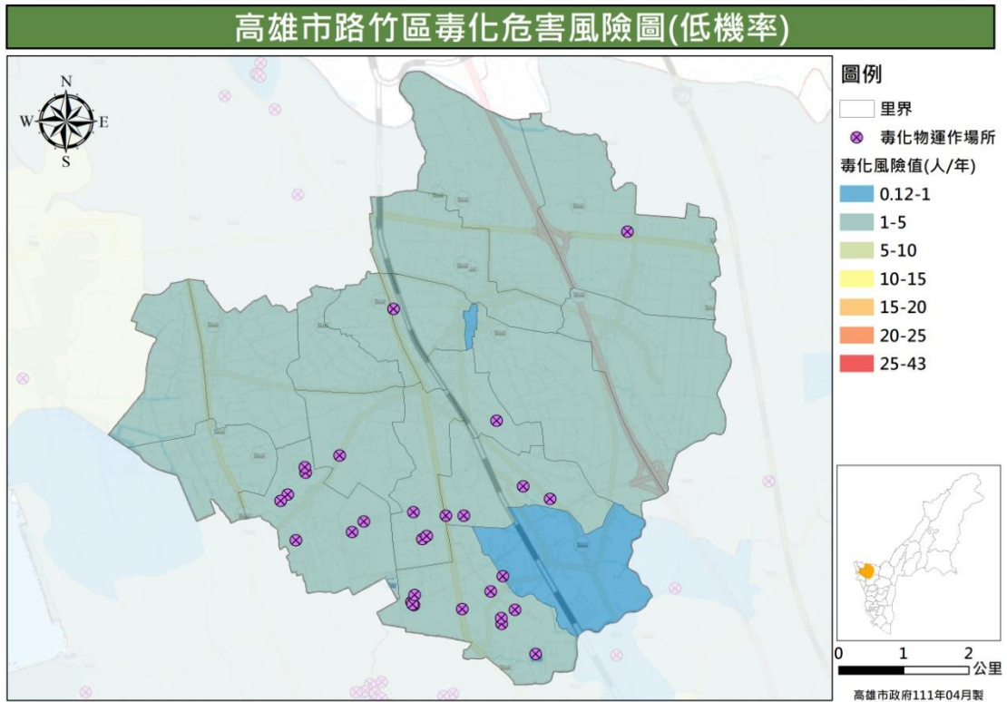
圖 28 路竹區毒性化學物質災害危害風險潛勢圖（低機率）
