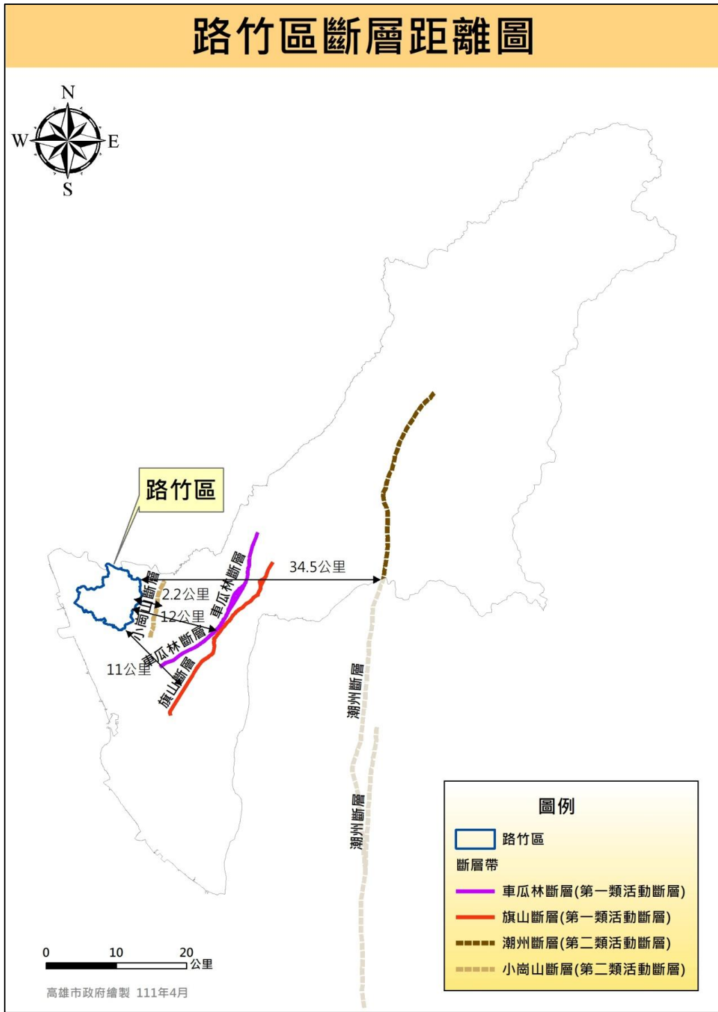
圖 10 路竹區與高雄市斷層分布相對位置圖
