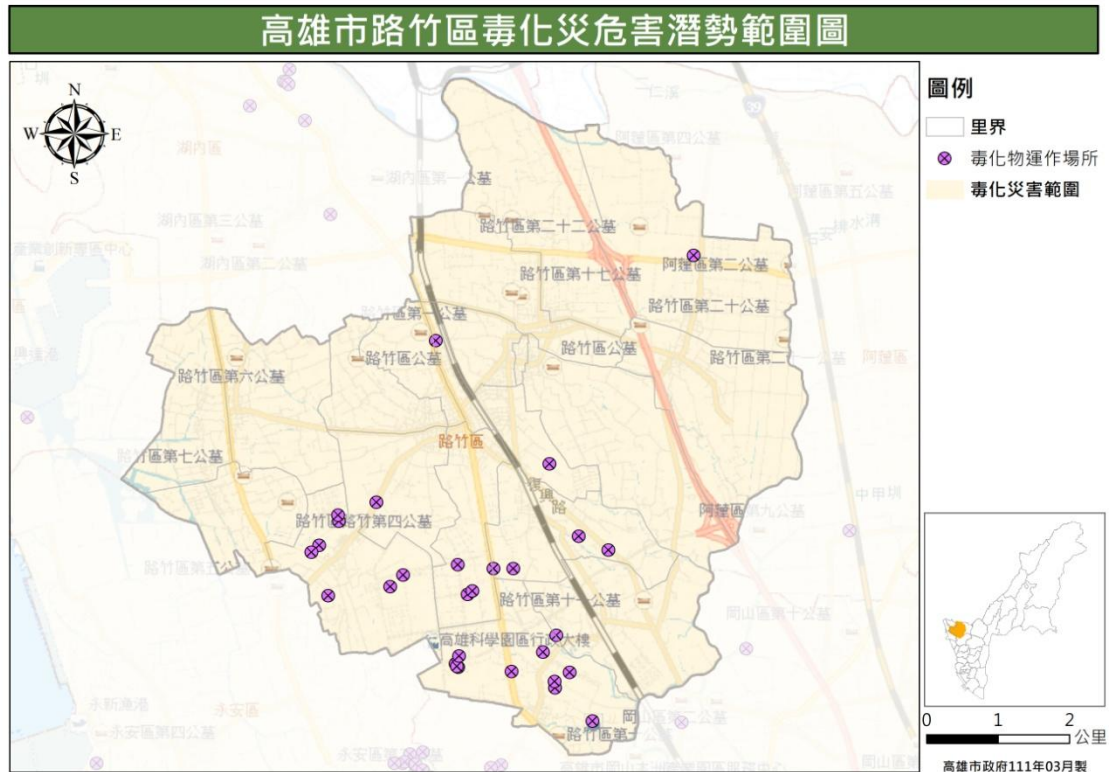
圖 27 路竹區毒性化學物質災害危害潛勢範圍圖
