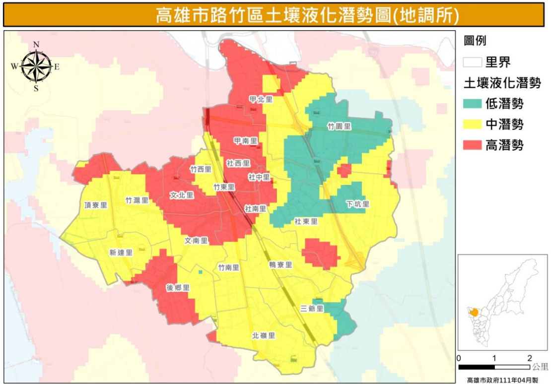
圖 23 路竹區土壤液化潛勢圖 (資料來源：經濟部中央地質調查所)
