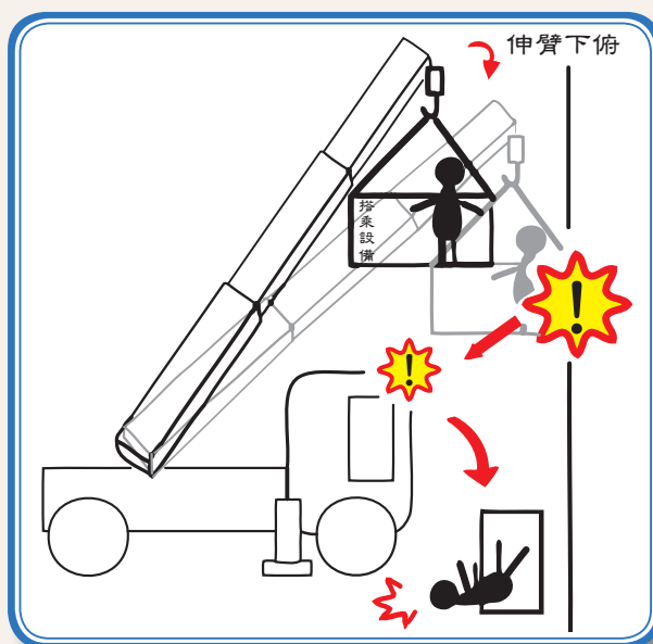
圖1 職災案例1之示意圖
