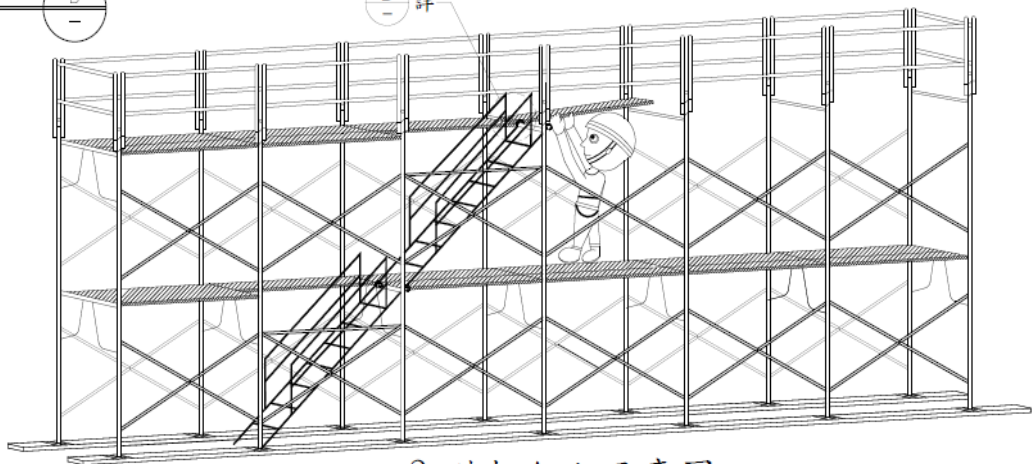
2. 踏板組立示意圖
