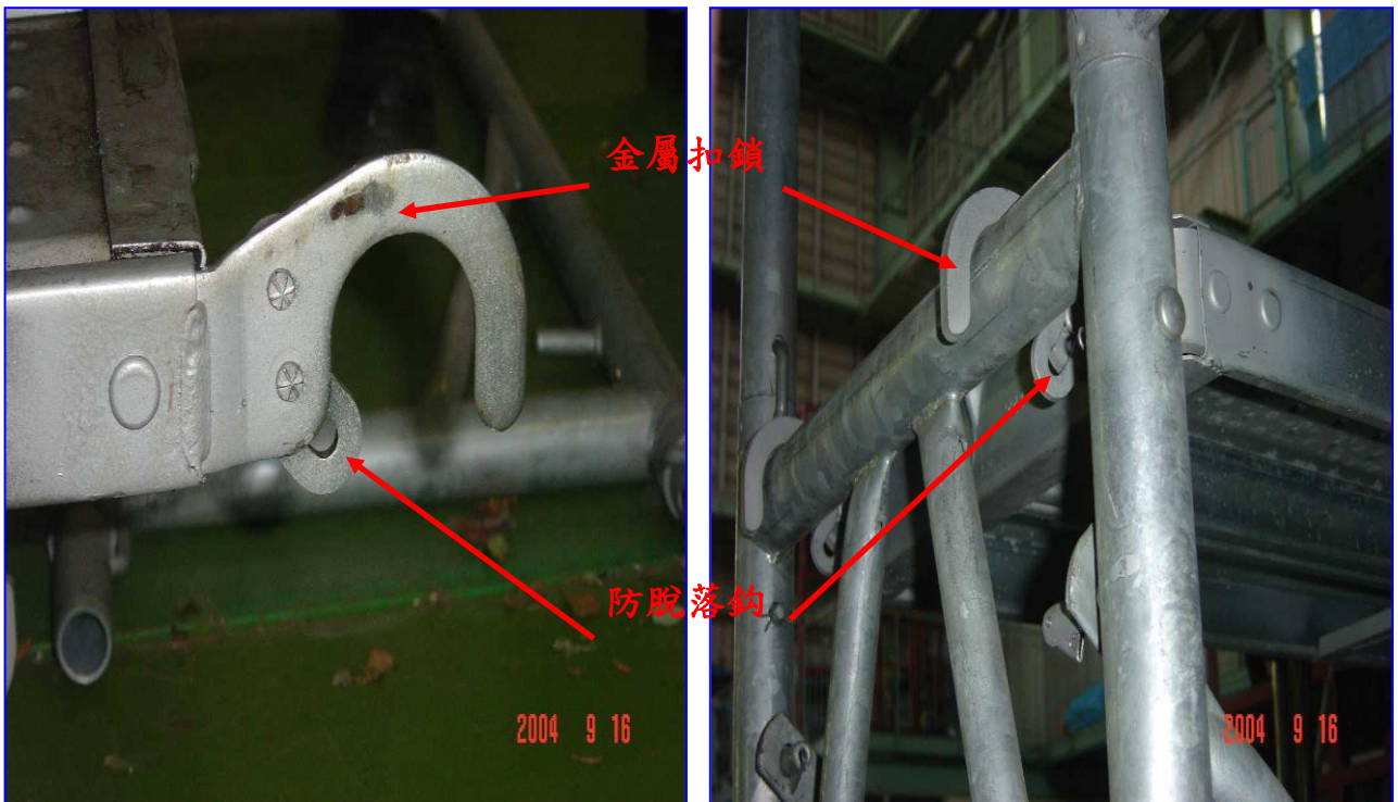
照片 6：踏板應設金屬扣鎖及防脫落鉤，以固定避免翻覆。
