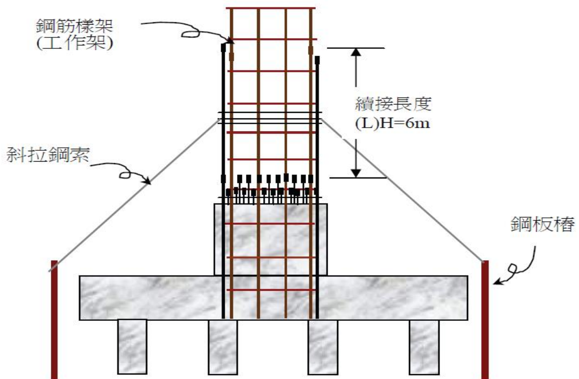
圖1：橋梁墩柱鋼筋續接及鋼筋樣架示意圖
