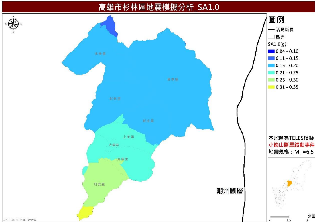
圖 9 小崗山斷層錯動事件長周期譜加速度 (SA1.0) 分布圖
