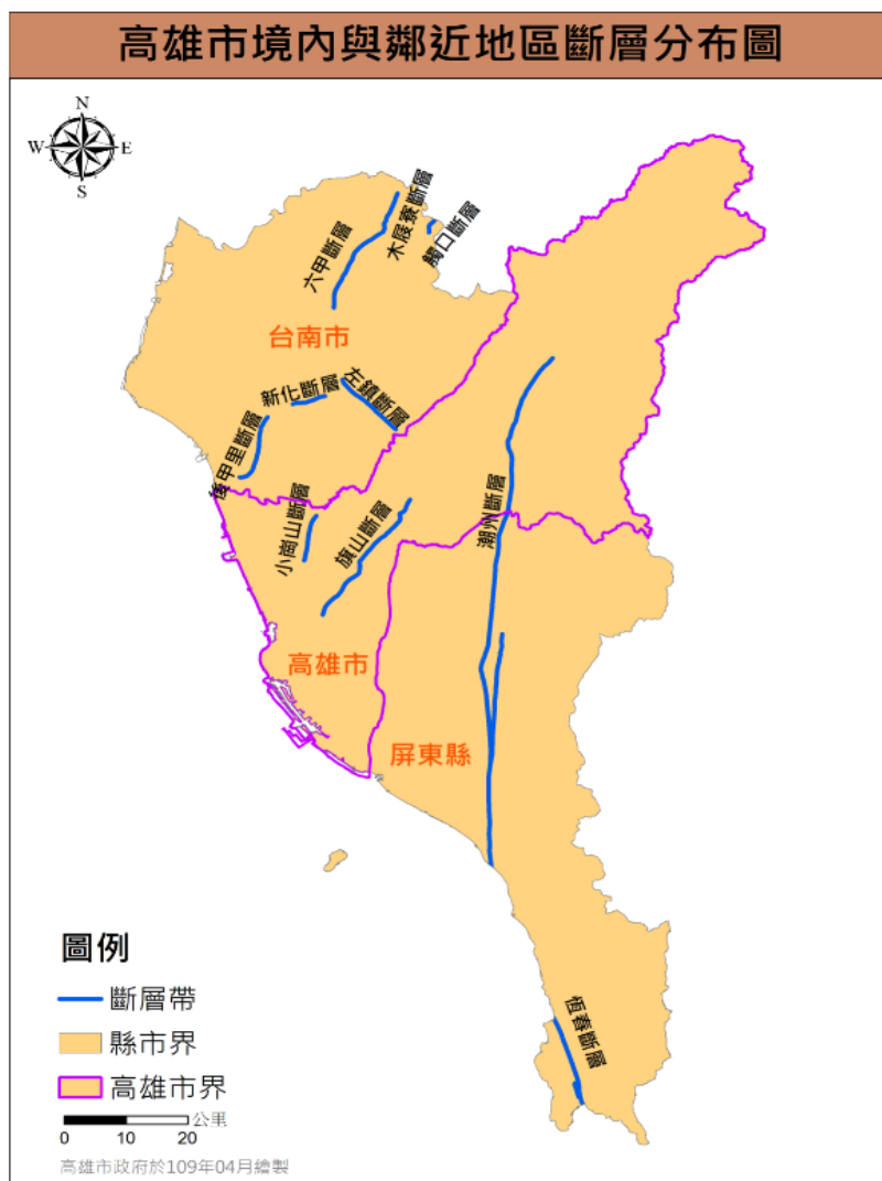
圖 5 高雄市境內與鄰近地區斷層分布圖
