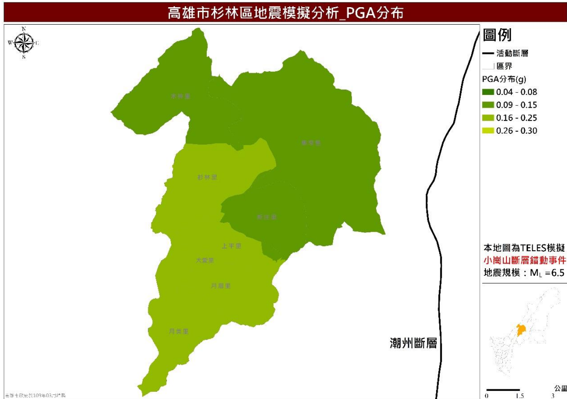
圖 7 小崗山斷層錯動事件最大地表加速度 (PGA) 分布圖
