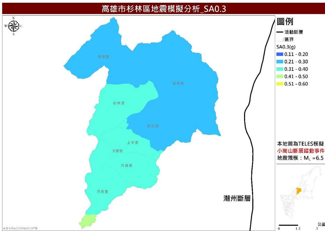
圖 8 小崗山斷層錯動事件短周期譜加速度 (SA0.3) 分布圖
