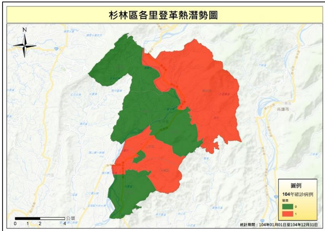
圖 22 杉林區登革熱潛勢分布圖(104 年)
