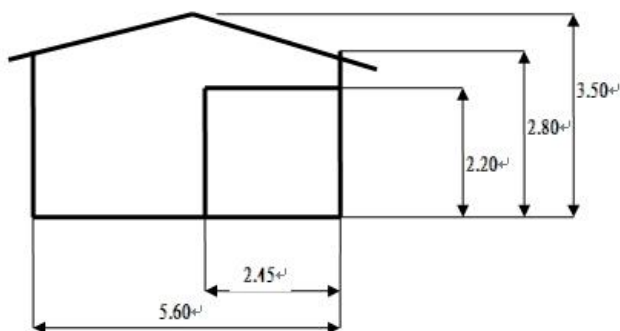
正立面圖
