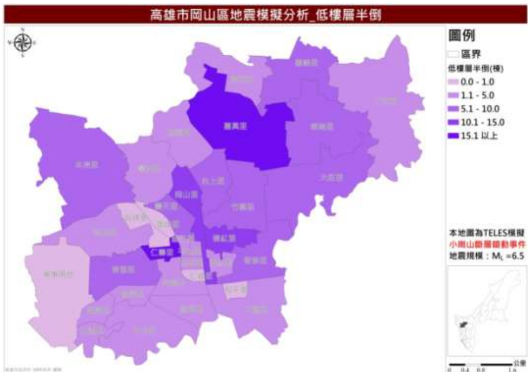
圖 25 小崗山斷層錯動事件低樓層半倒棟數推估圖
