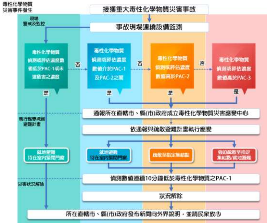
圖 40 毒性化學物質災害疏散避難計畫作業流程圖
