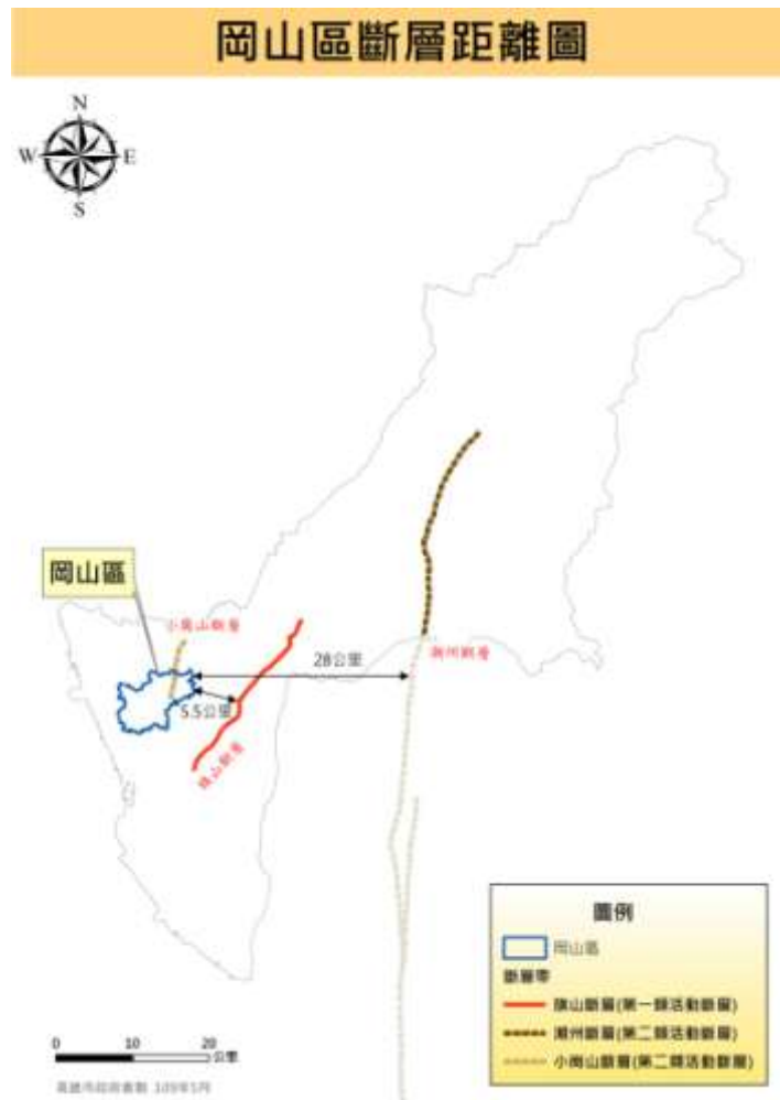
圖 17 岡山區與高雄市斷層分布相對位置圖
