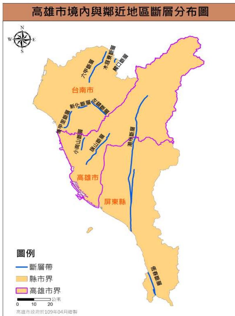
圖 16 高雄市境內與鄰近地區斷層分布圖
