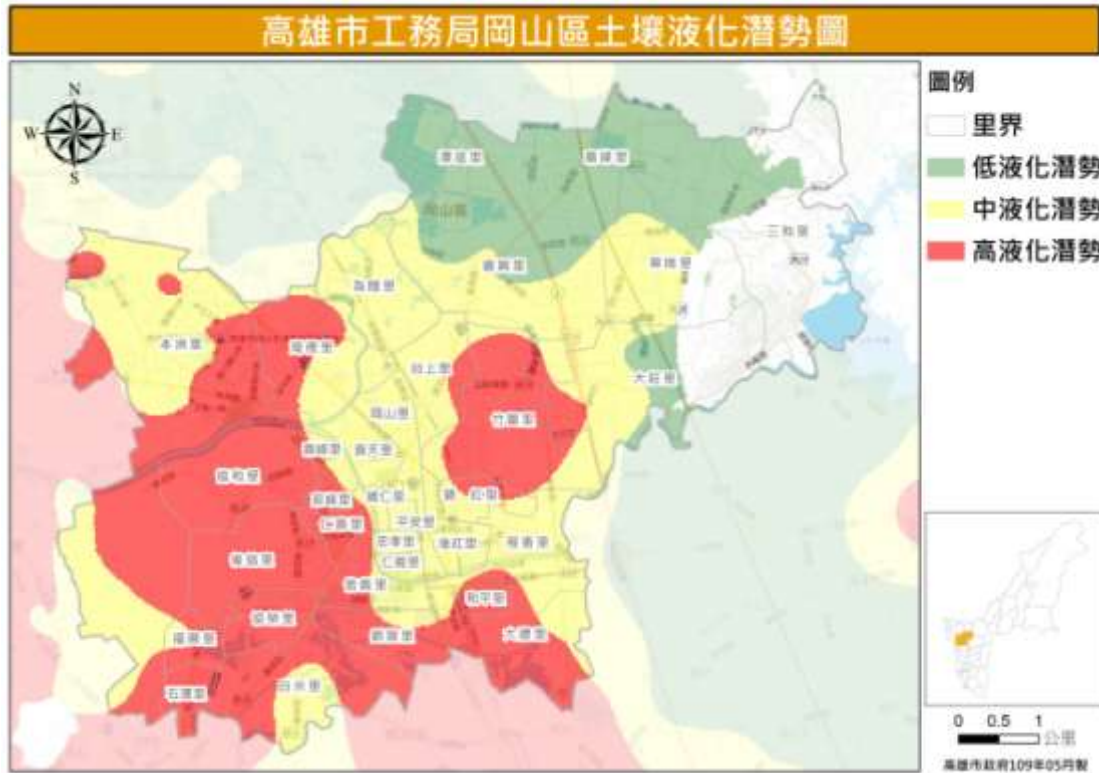
圖 32 岡山區土壤液化潛勢圖（資料來源：高雄市政府工務局）
