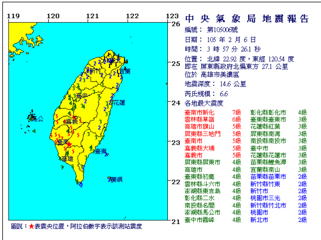
圖 30 第 105006 號高雄市美濃地震參數及各地震度分布
