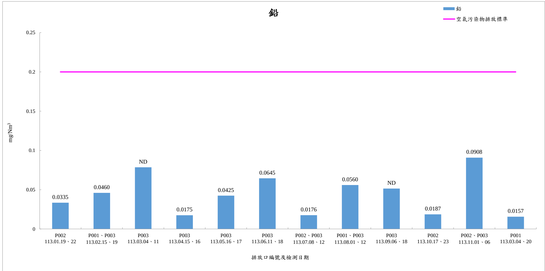
113 年 1 月-113 年 12 月煙道廢氣檢測結果-鉛
