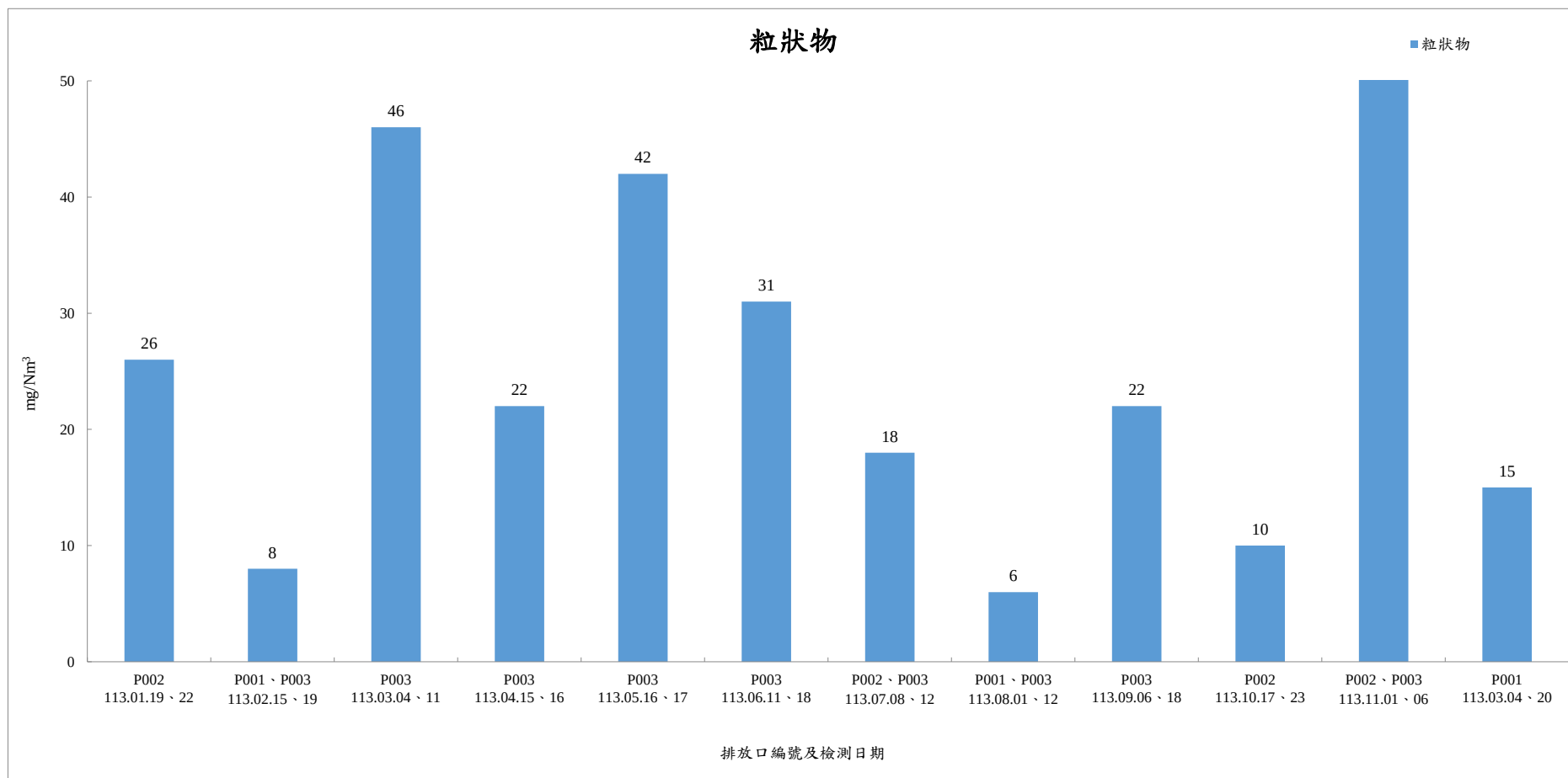
113 年 1 月-113 年 12 月煙道廢氣檢測結果-粒狀物
