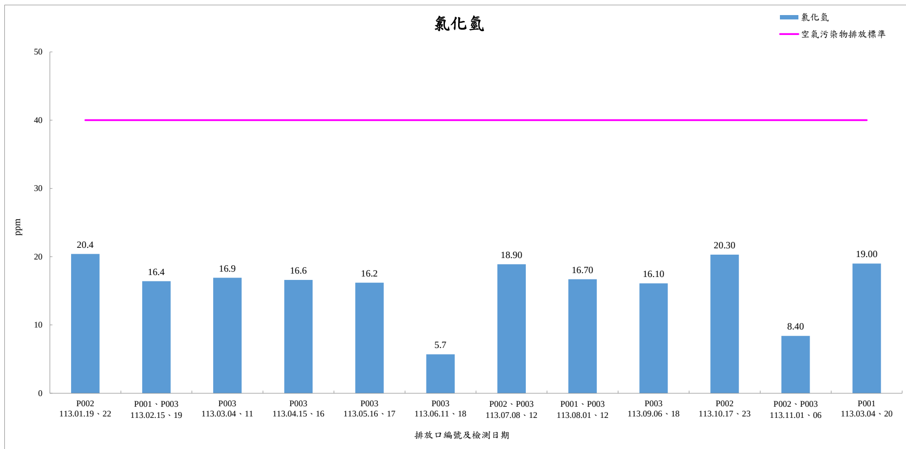
113 年 1 月-113 年 12 月煙道廢氣檢測結果-氯化氫
