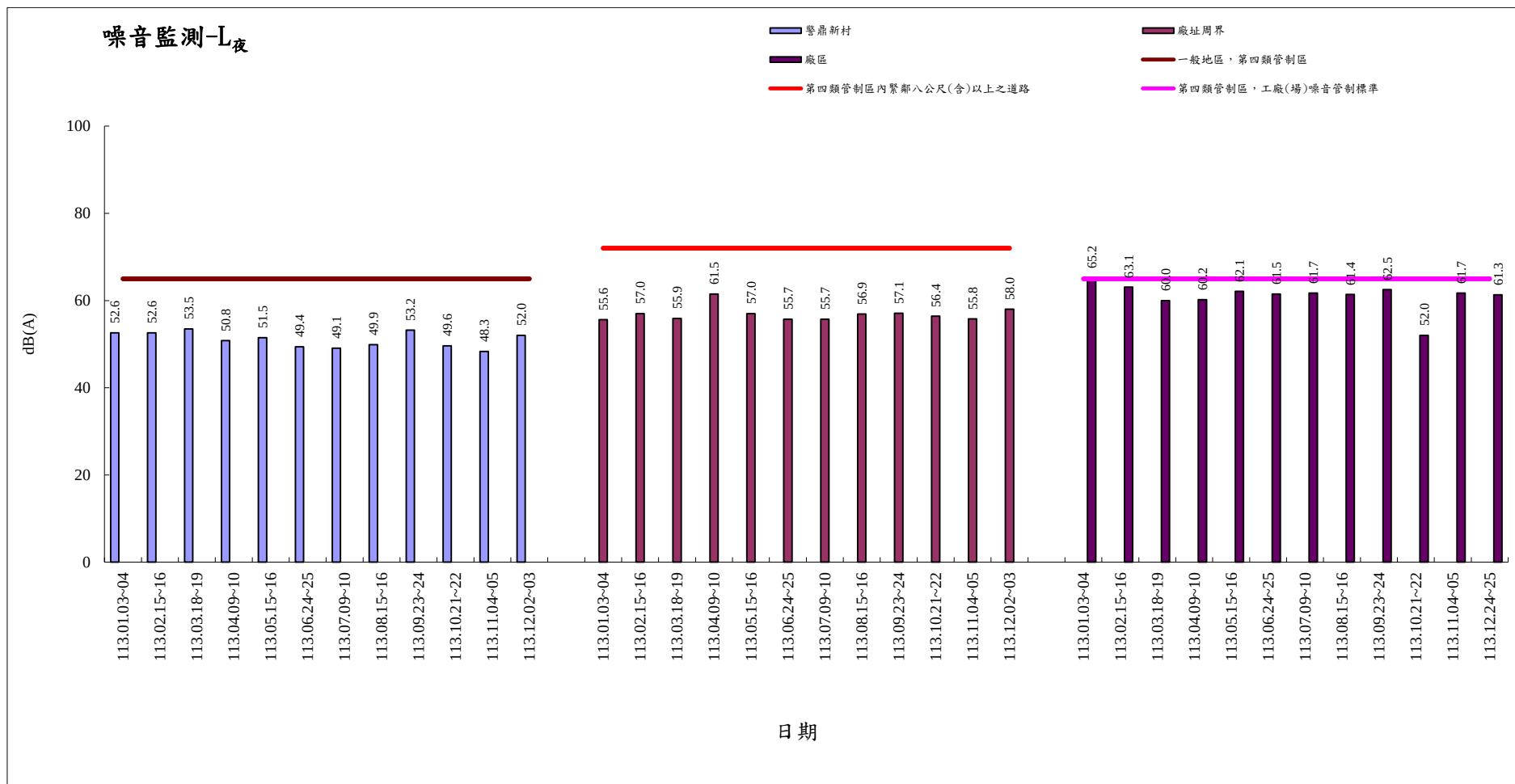
113 年 1 月-113 年 12 月噪音監測(L 夜 )
