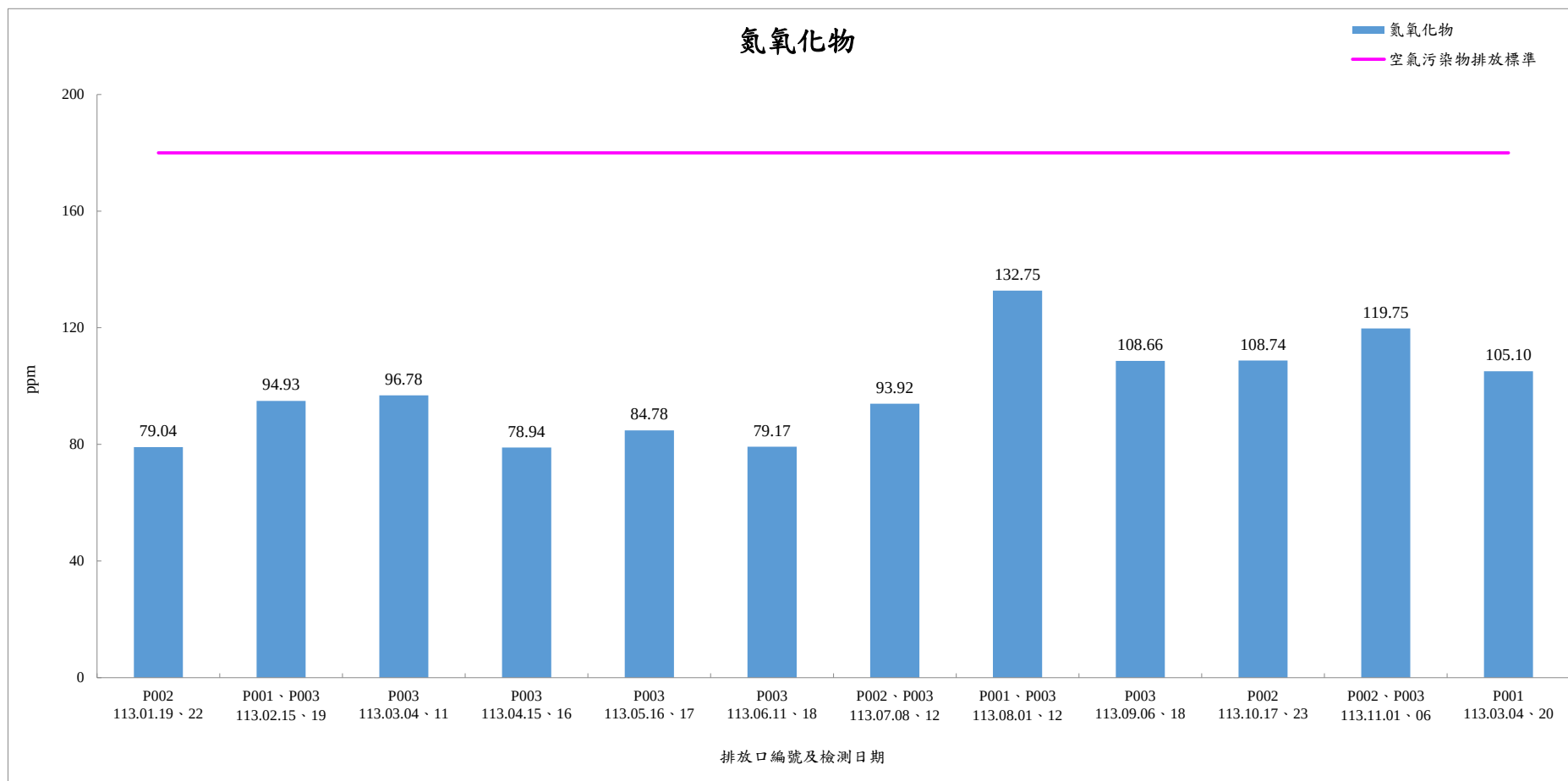
113 年 1 月-113 年 12 月煙道廢氣檢測結果-氮氧化物
