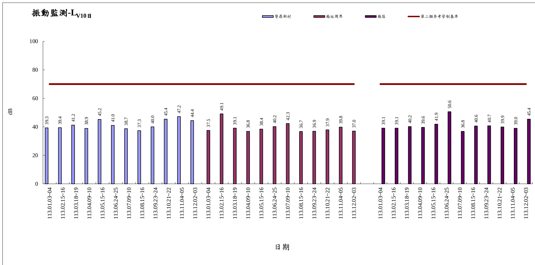
113 年 1 月-113 年 12 月振動監測(L V10 日)
