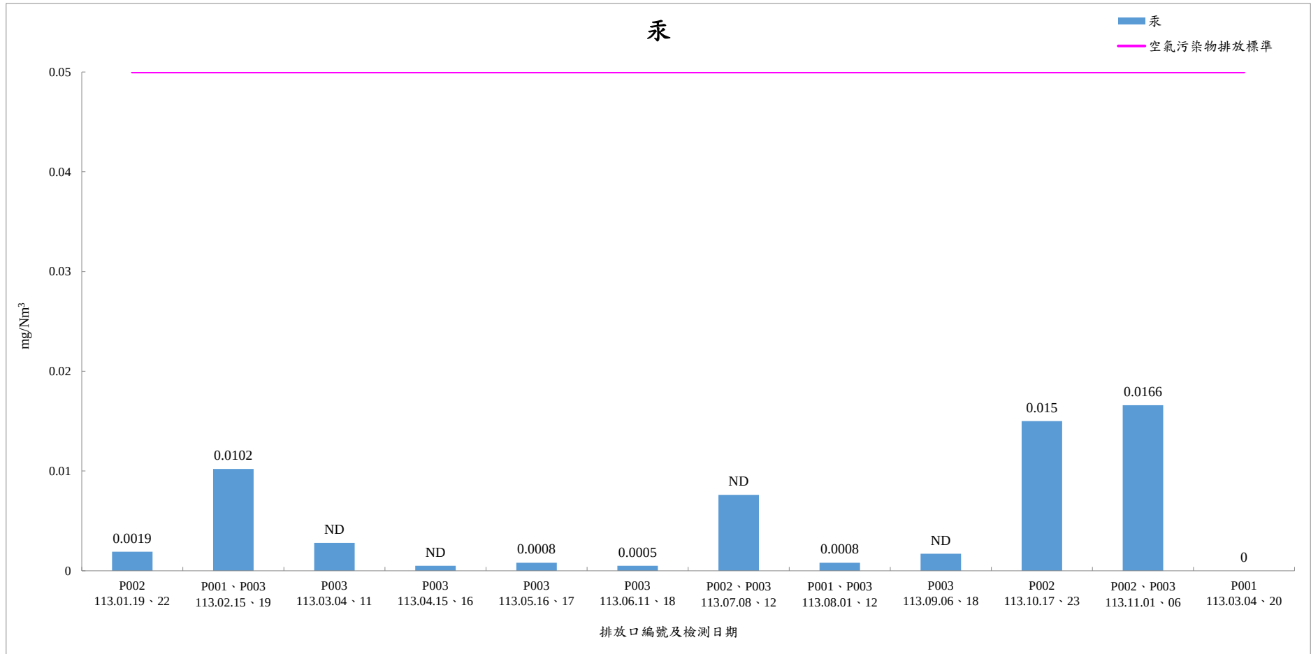
113 年 1 月-113 年 12 月煙道廢氣檢測結果-汞
