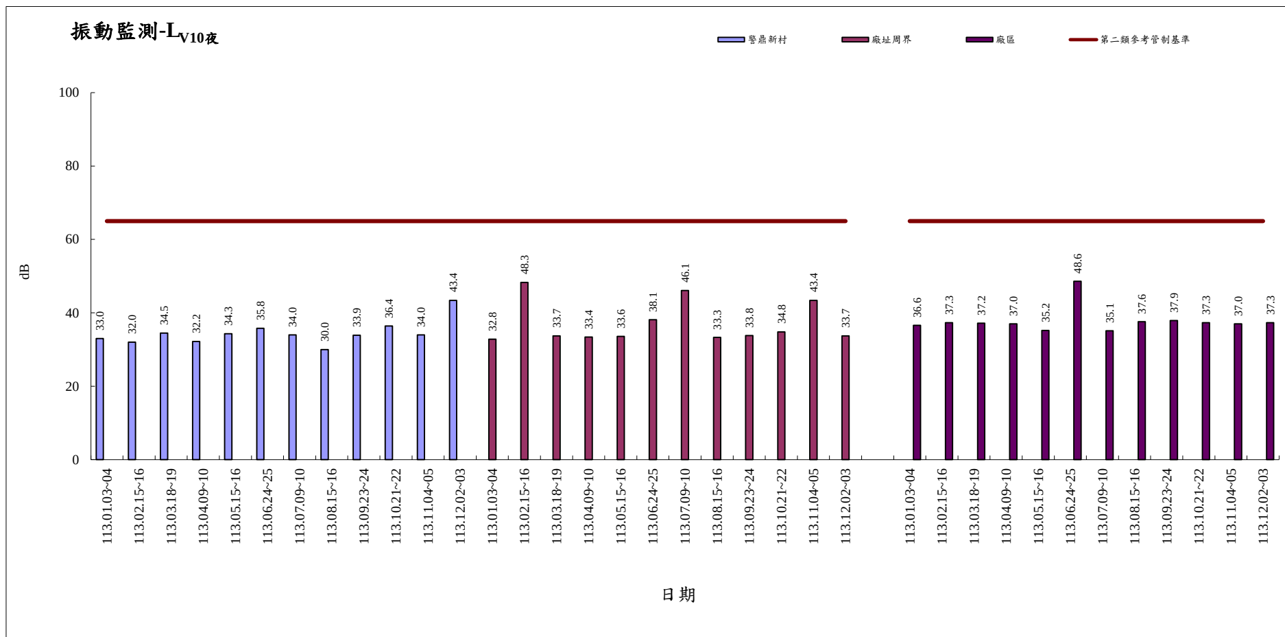
113 年 1 月-113 年 12 月振動監測(L V10 夜)
