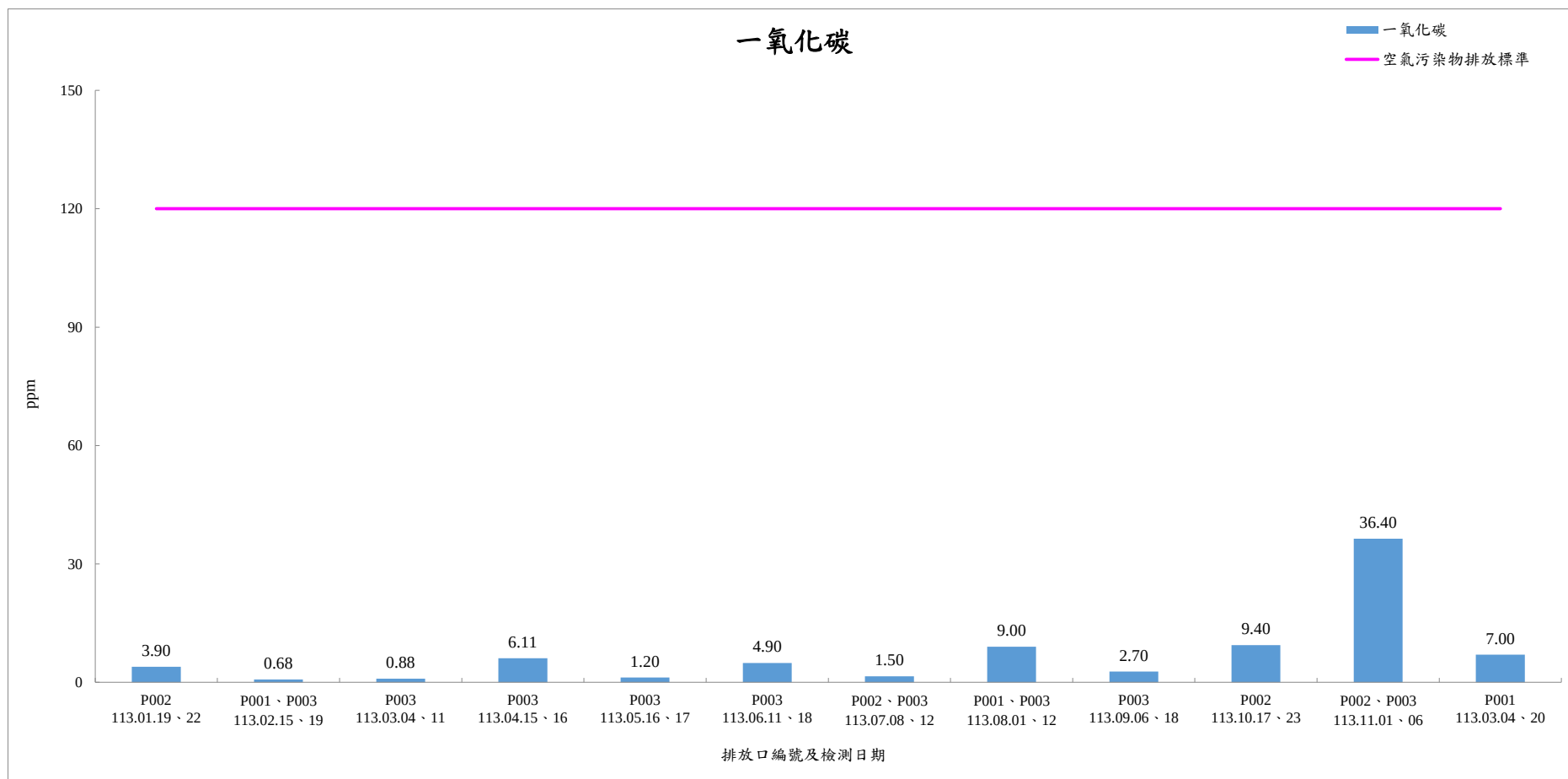
113 年 1 月-113 年 12 月煙道廢氣檢測結果-一氧化碳
