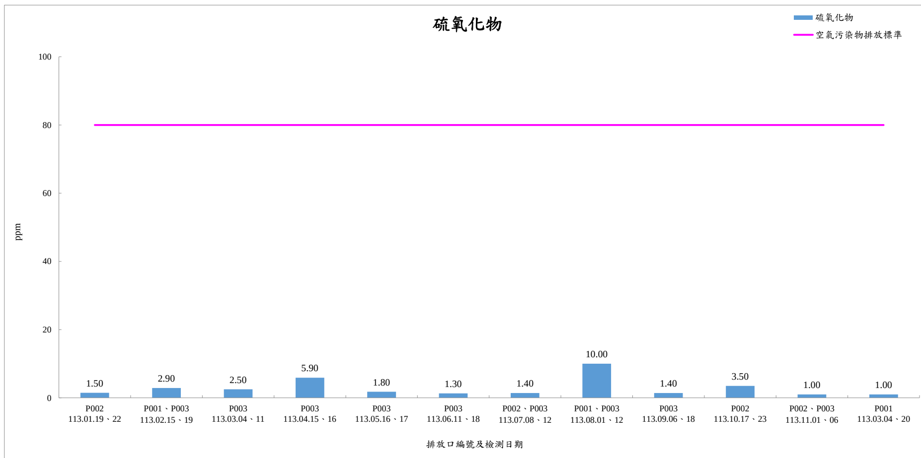
113 年 1 月-113 年 12 月煙道廢氣檢測結果-硫氧化物
