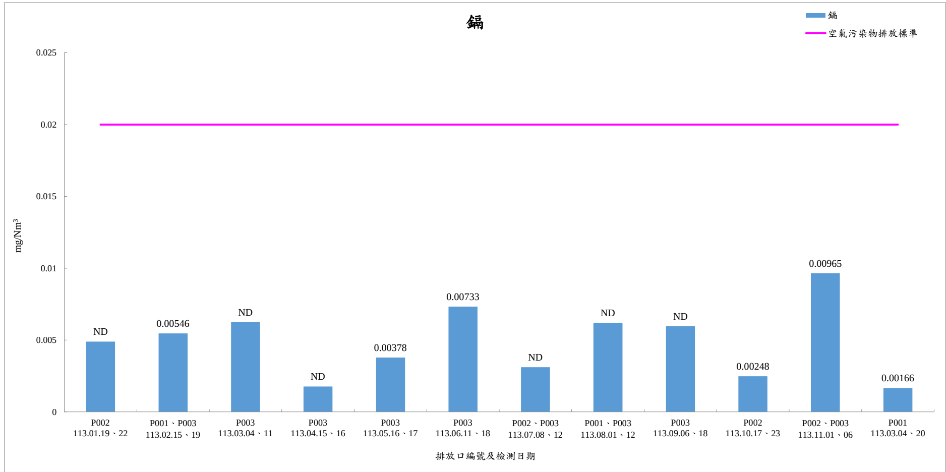
113 年 1 月-113 年 12 月煙道廢氣檢測結果-鎘
