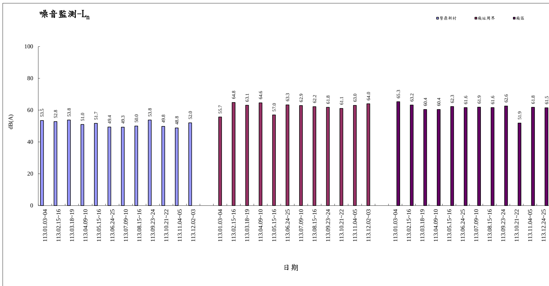
113 年 1 月-113 年 12 月噪音監測( L_n )
