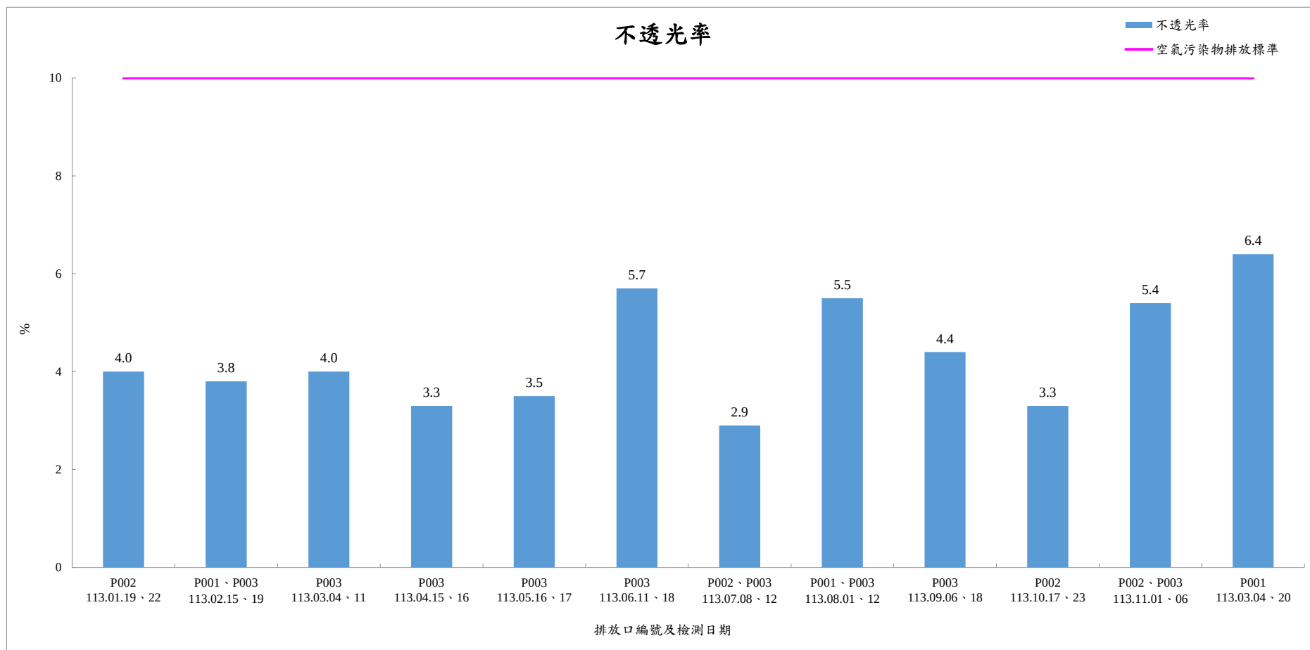
113 年 1 月-113 年 12 月煙道廢氣檢測結果-不透光率
