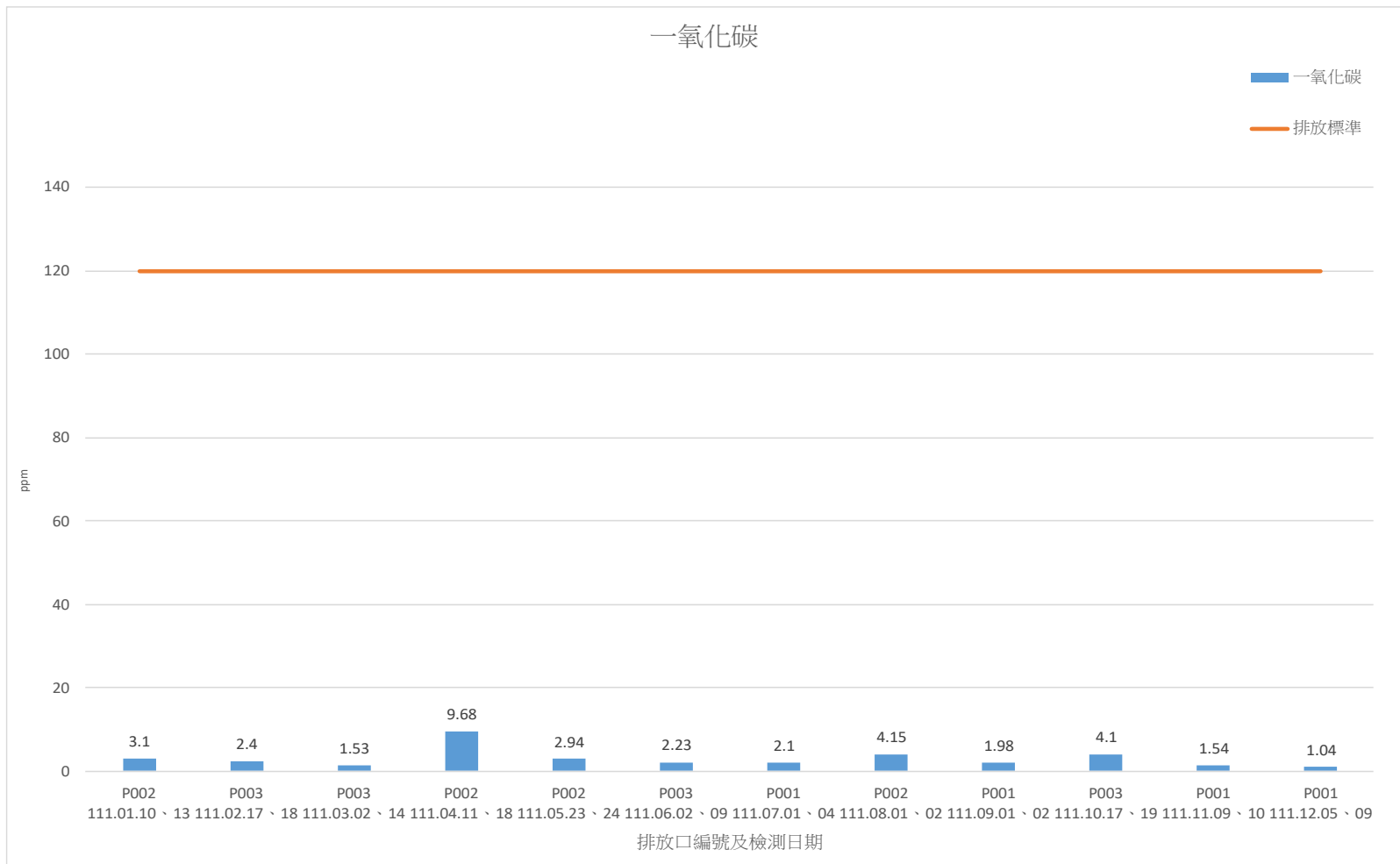
111 年 1 月-111 年 12 月煙道廢氣檢測結果-一氧化碳
