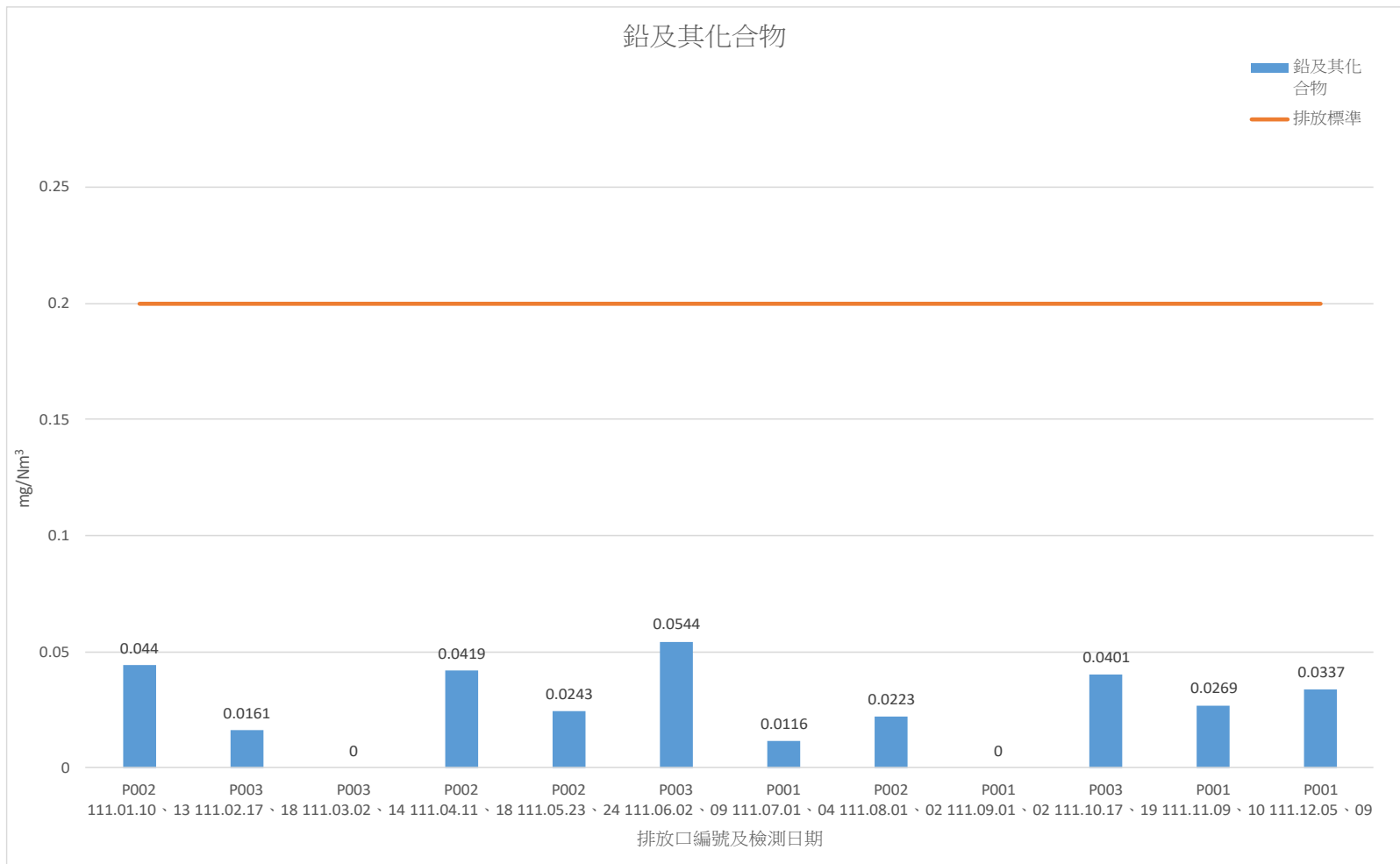
111 年 1 月-111 年 12 月煙道廢氣檢測結果-鉛
