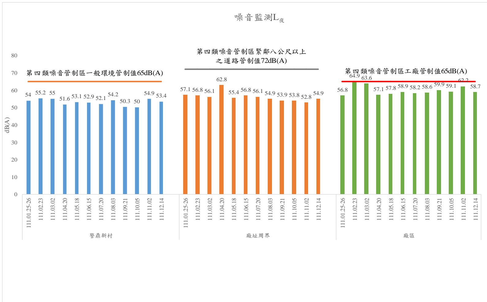
111 年 1 月-111 年 12 月噪音監測(L 夜 )
