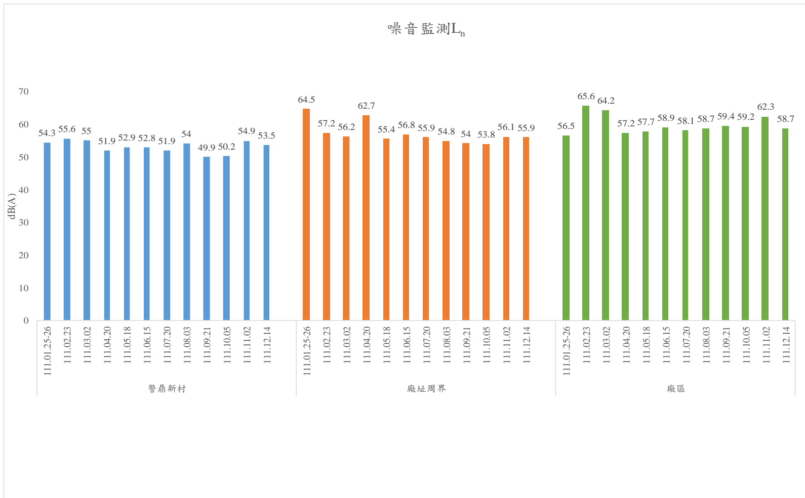
111 年 1 月-111 年 12 月噪音監測( L_n )
