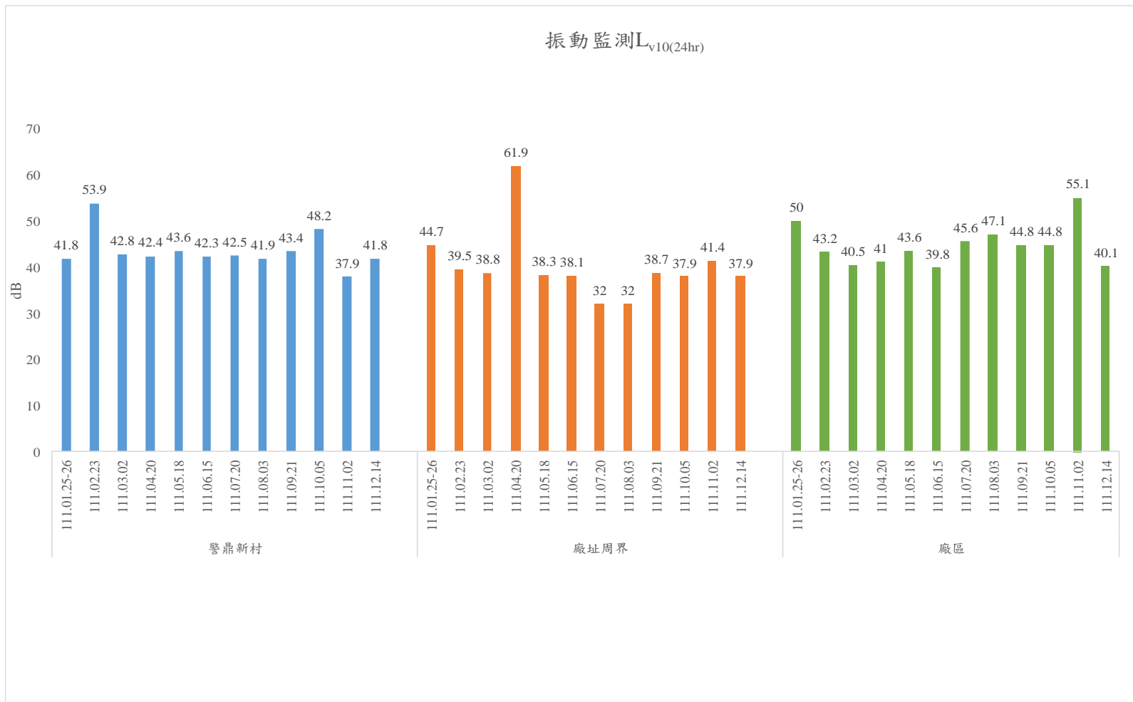
111 年 1 月-111 年 12 月振動監測( L_{v10(24hr)} )
