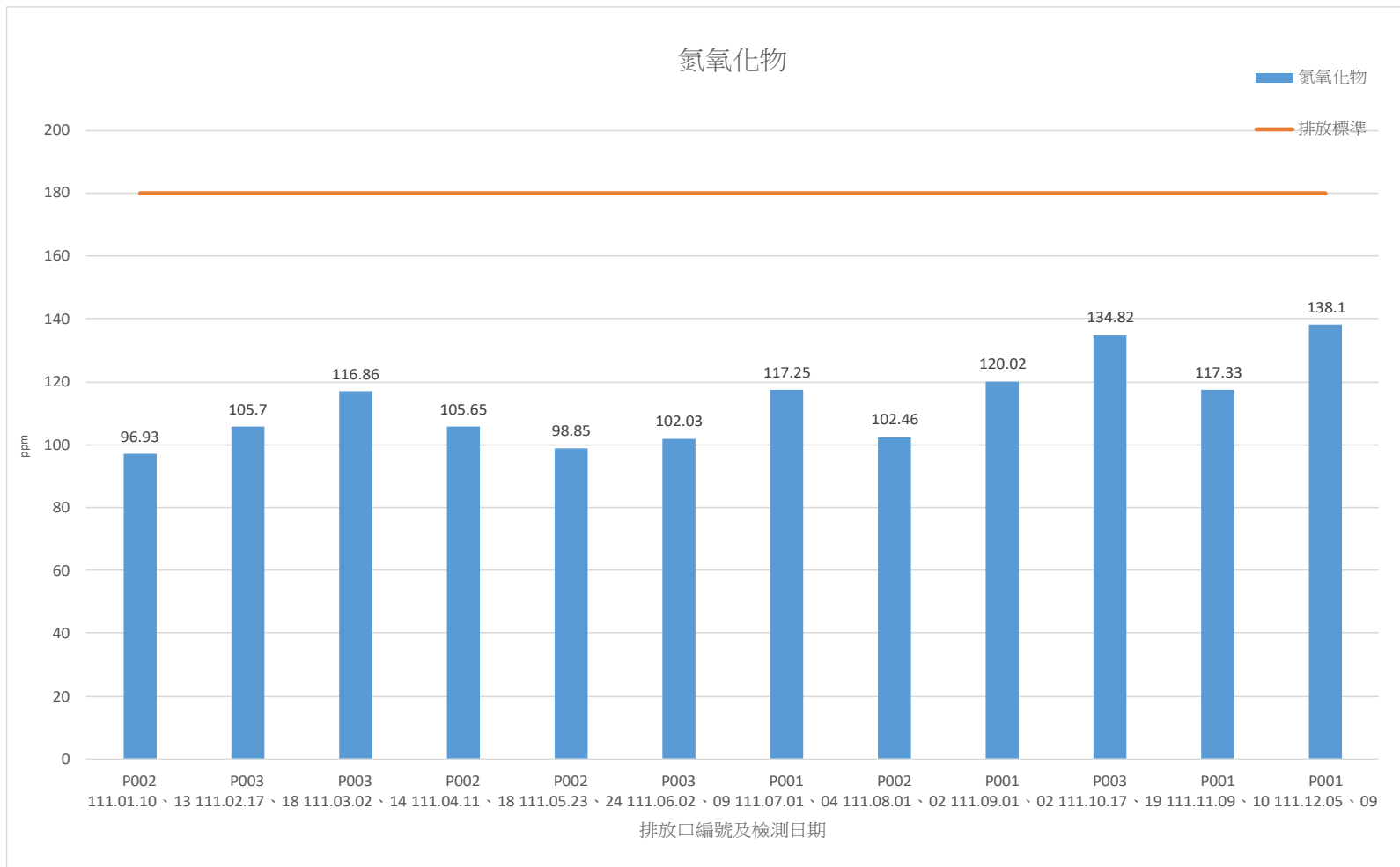
111 年 1 月-111 年 12 月煙道廢氣檢測結果-氮氧化物
