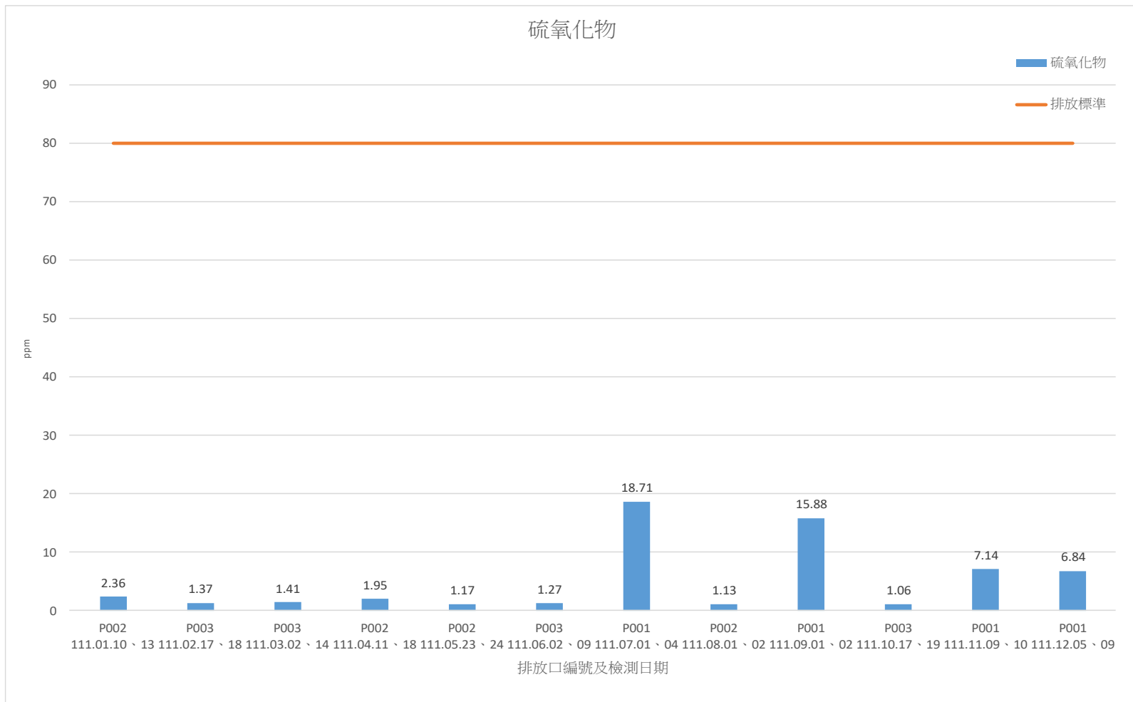
111 年 1 月-111 年 12 月煙道廢氣檢測結果-硫氧化物
