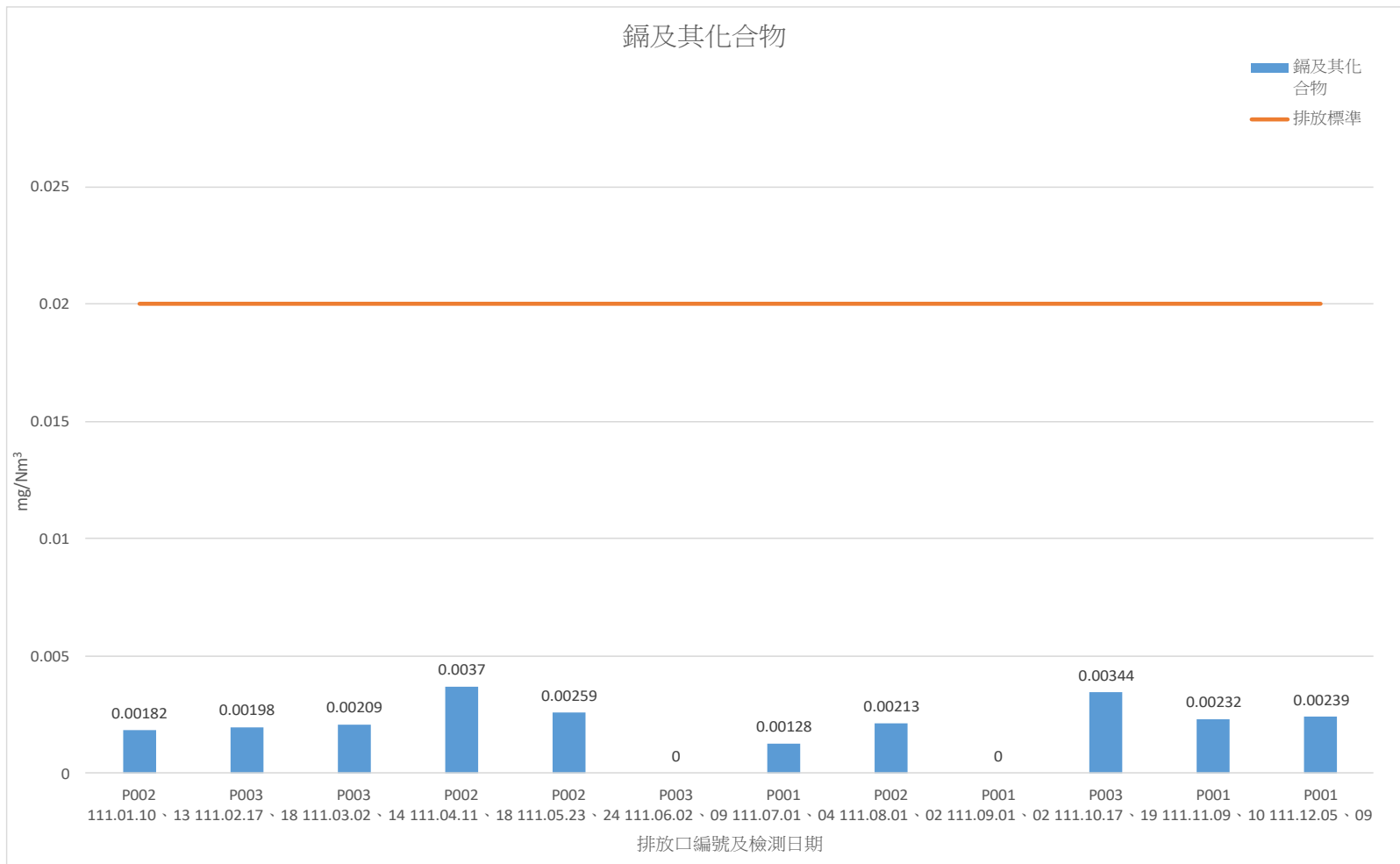
111 年 1 月-111 年 12 月煙道廢氣檢測結果-鎘
