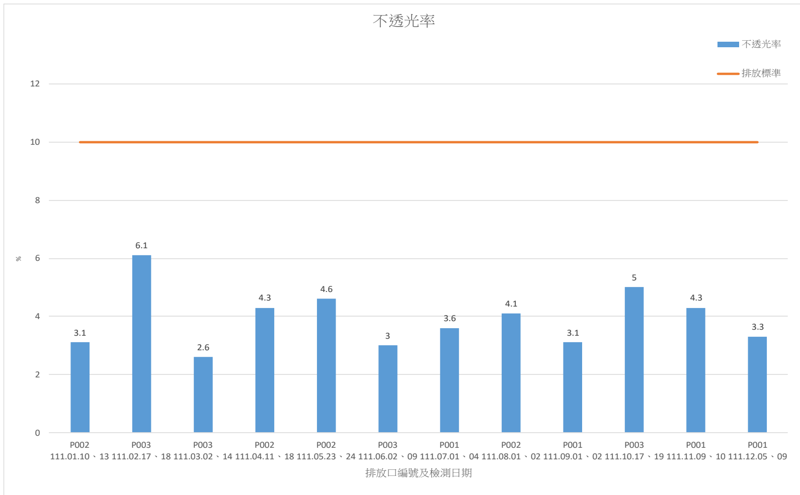
111 年 1 月-111 年 12 月煙道廢氣檢測結果-不透光率
