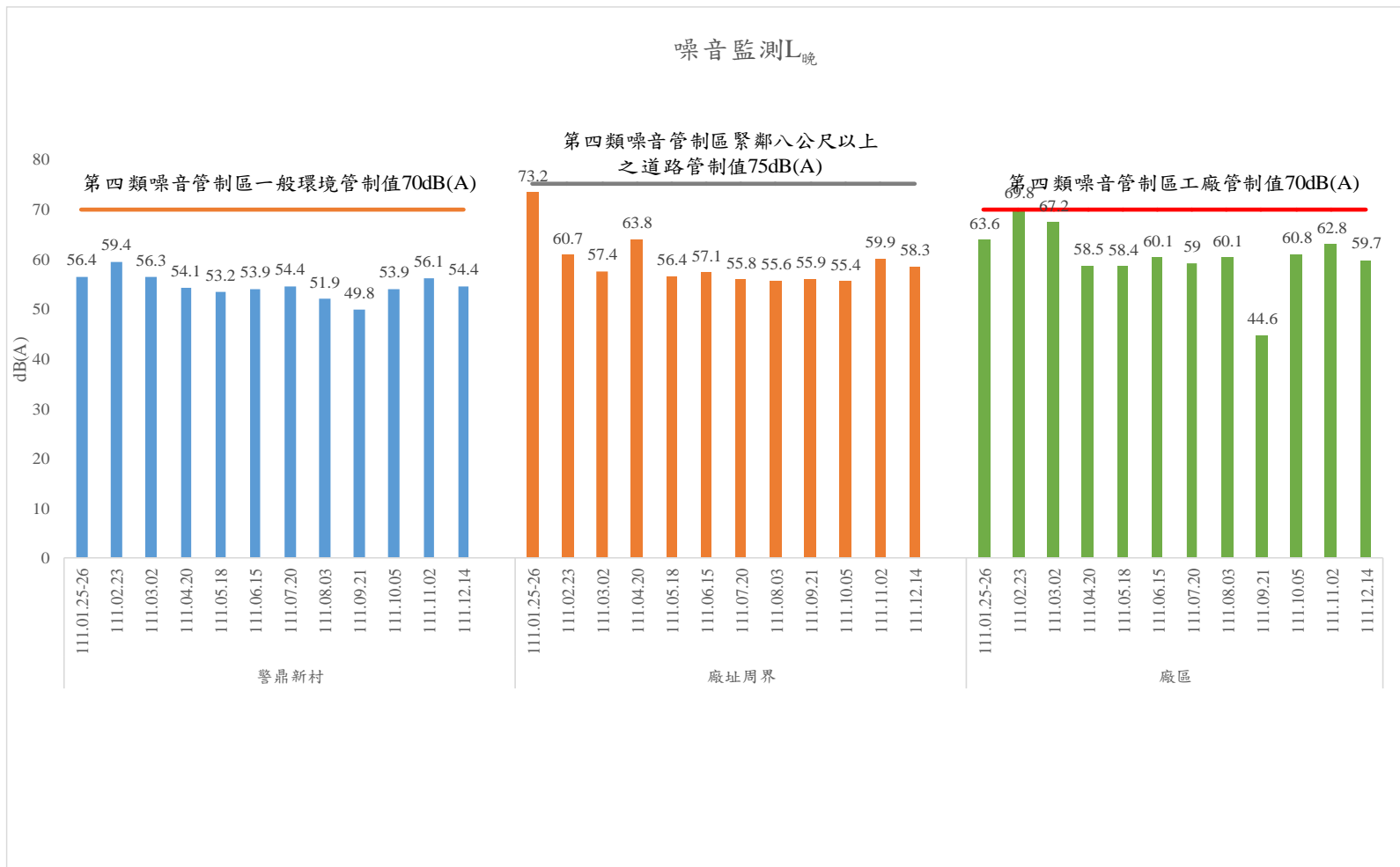
111 年 1 月-111 年 12 月噪音監測(L 晚 )
