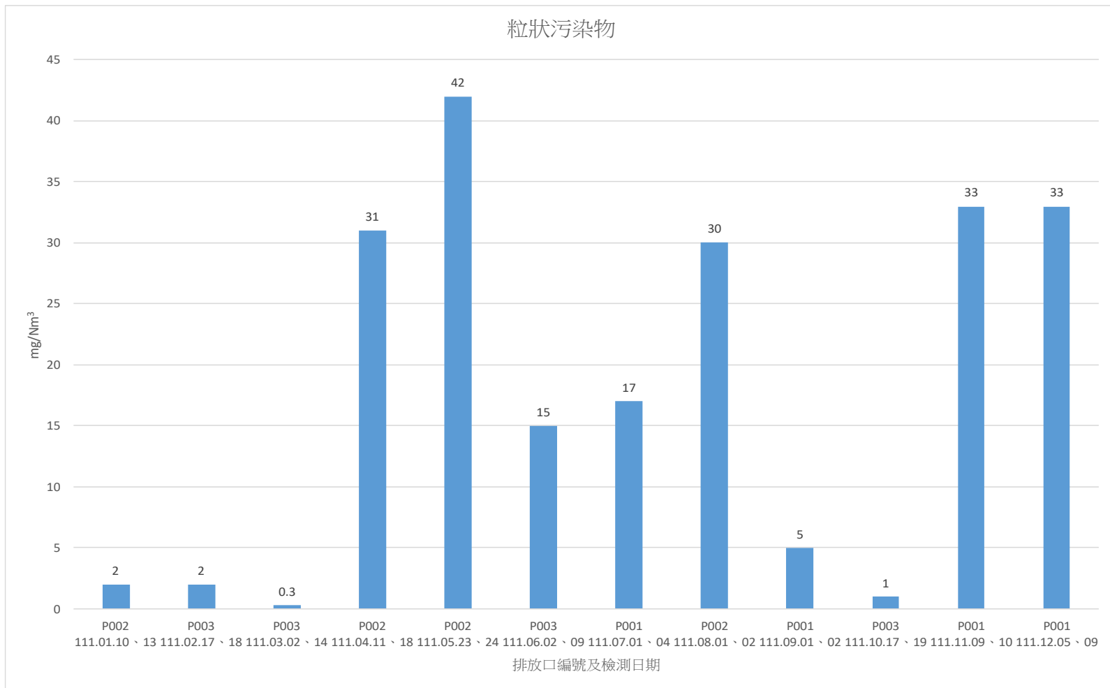
111 年 1 月-111 年 12 月煙道廢氣檢測結果-粒狀物
