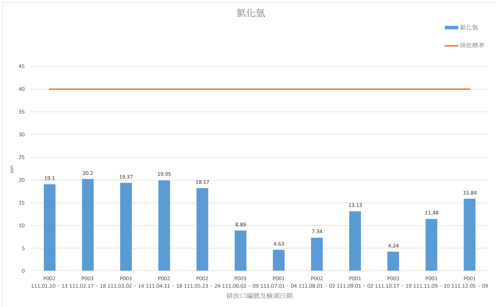
111 年 1 月-111 年 12 月煙道廢氣檢測結果-氯化氫
