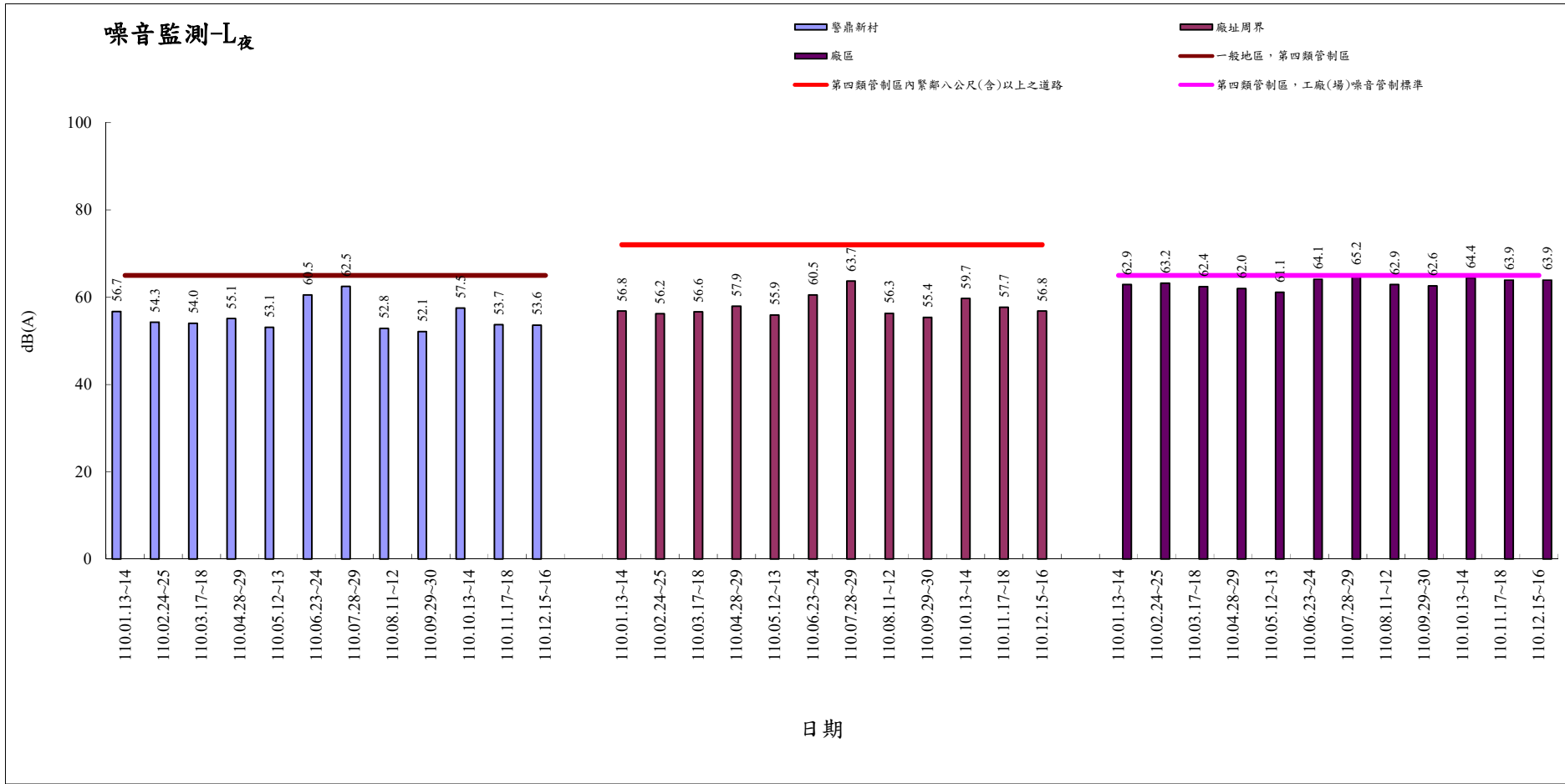
110年1月-110年12月噪音監測(L 夜 )
