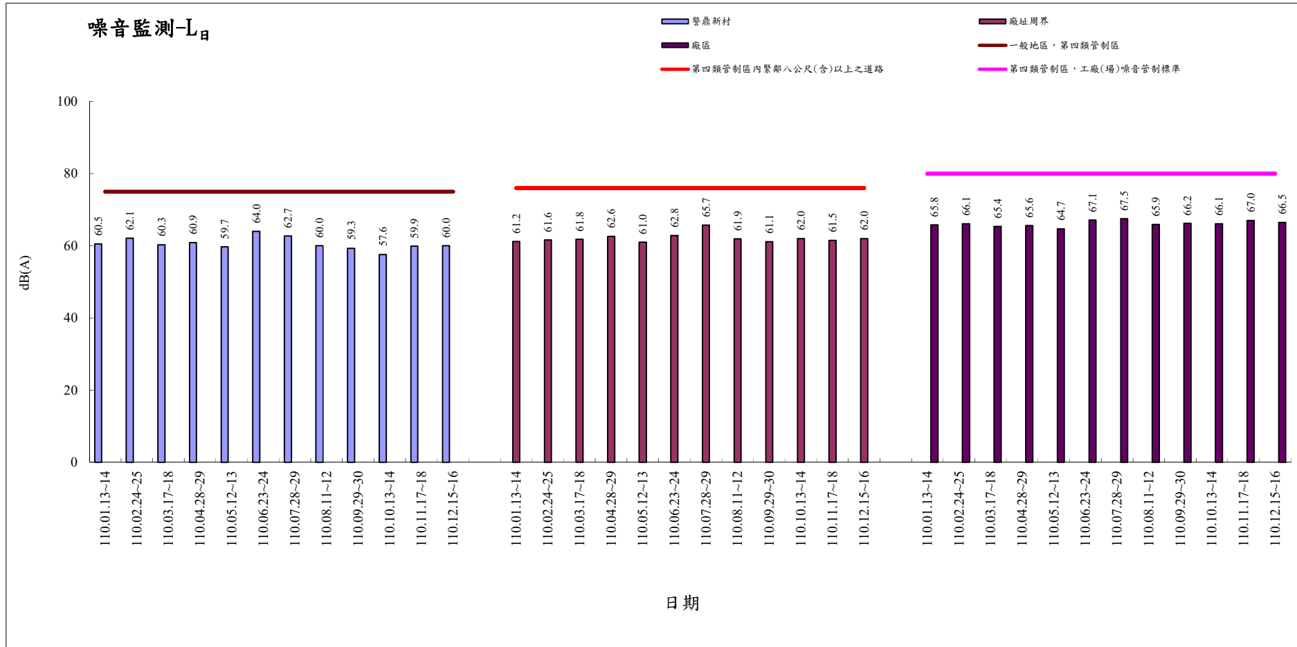
110年1月-110年12月噪音監測(L 日 )
