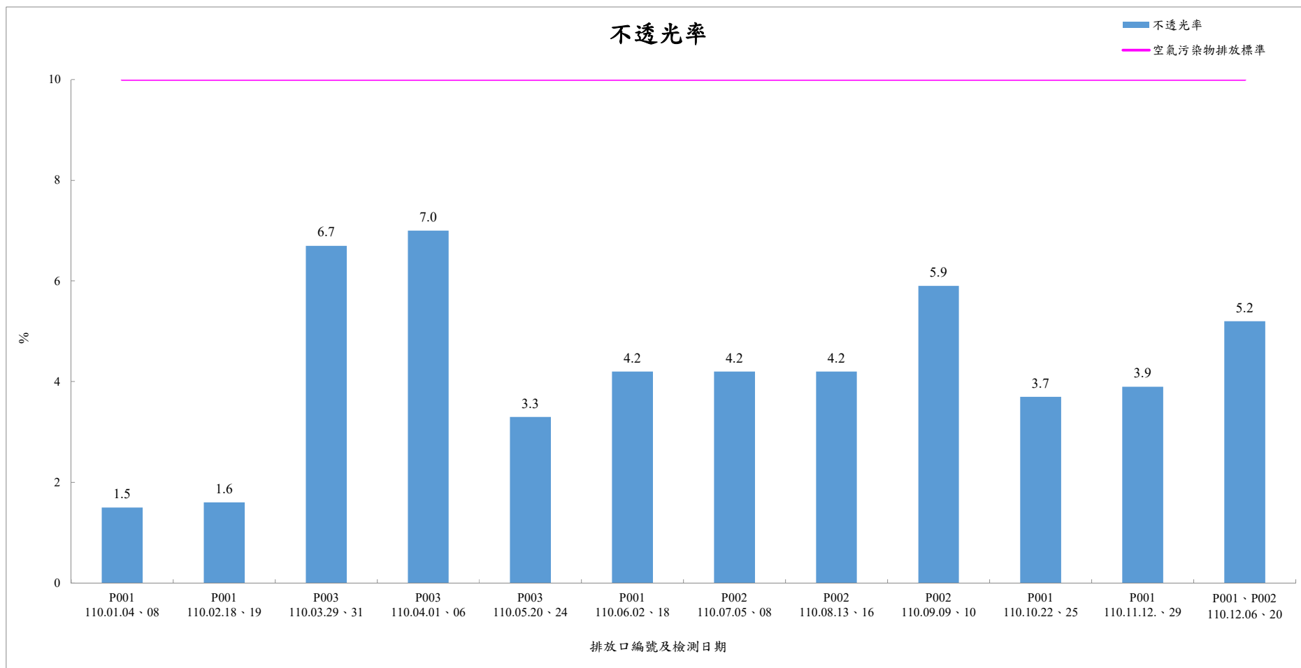
110年1月-110年12月煙道廢氣檢測結果-不透光率
