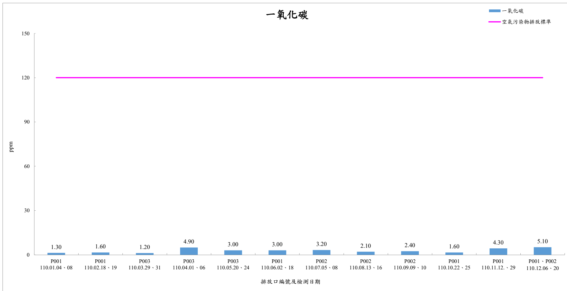
110年1月-110年12月煙道廢氣檢測結果-一氧化碳
