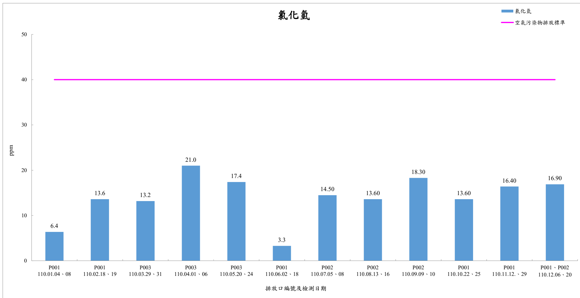
110年1月-110年12月煙道廢氣檢測結果-氯化氫
