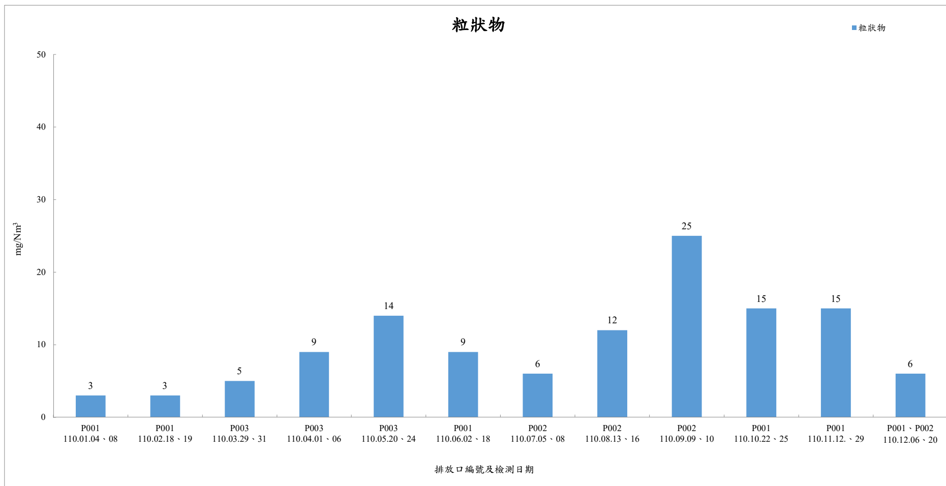
110年1月-110年12月煙道廢氣檢測結果-粒狀物
