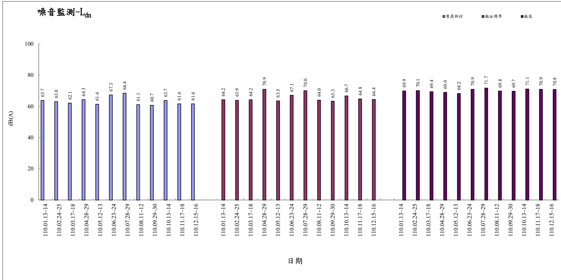
110年1月-110年12月噪音監測(L dn )
