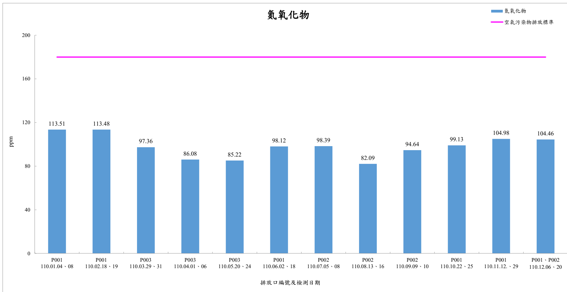
110年1月-110年12月煙道廢氣檢測結果-氮氧化物
