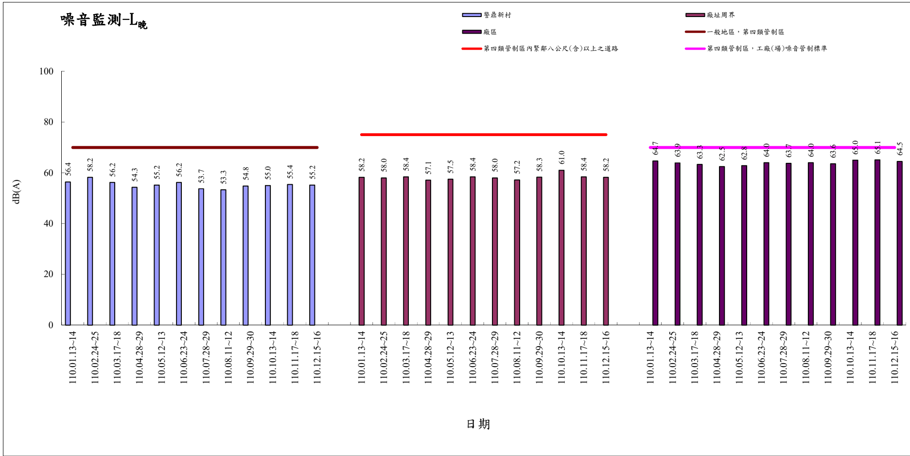
110年1月-110年12月噪音監測(L 晚 )
