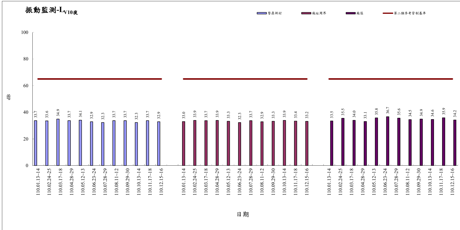
110年1月-110年12月振動監測(L V10 夜)
