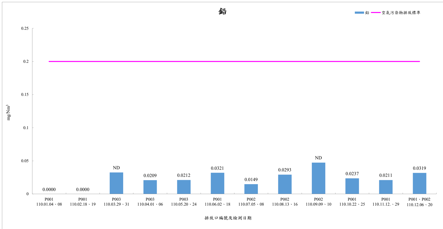
110年1月-110年12月煙道廢氣檢測結果-鉛
