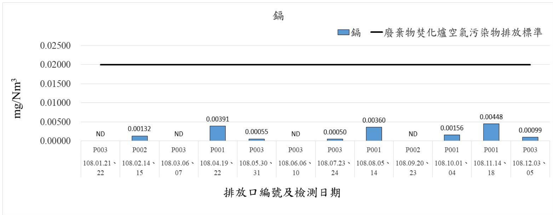
108年1月-108年12月煙道廢氣檢測結果-鎘
