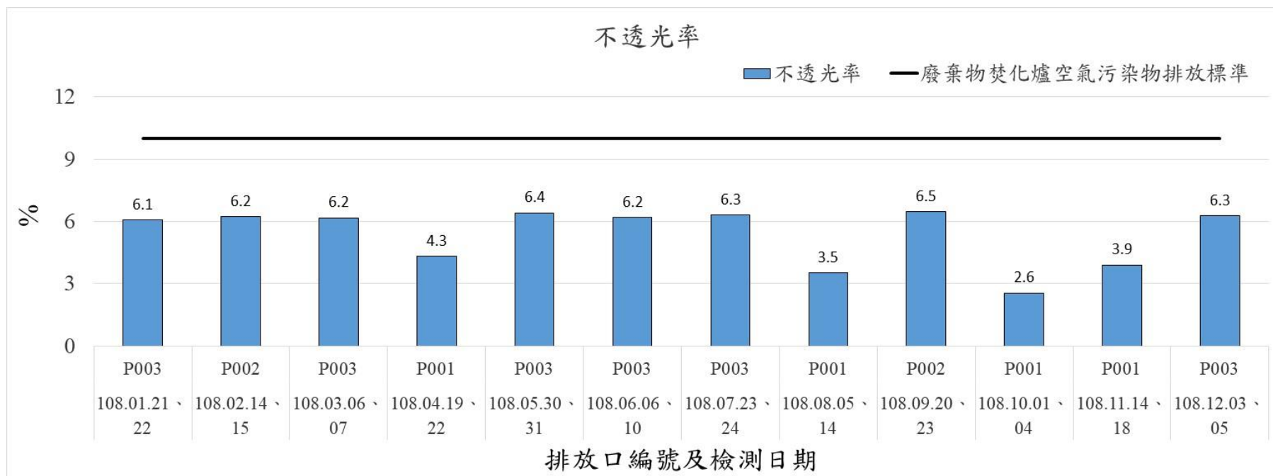
108年1月-108年12月煙道廢氣檢測結果-不透光率
