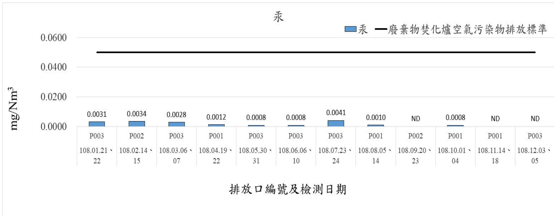
108年1月-108年12月煙道廢氣檢測結果-汞
