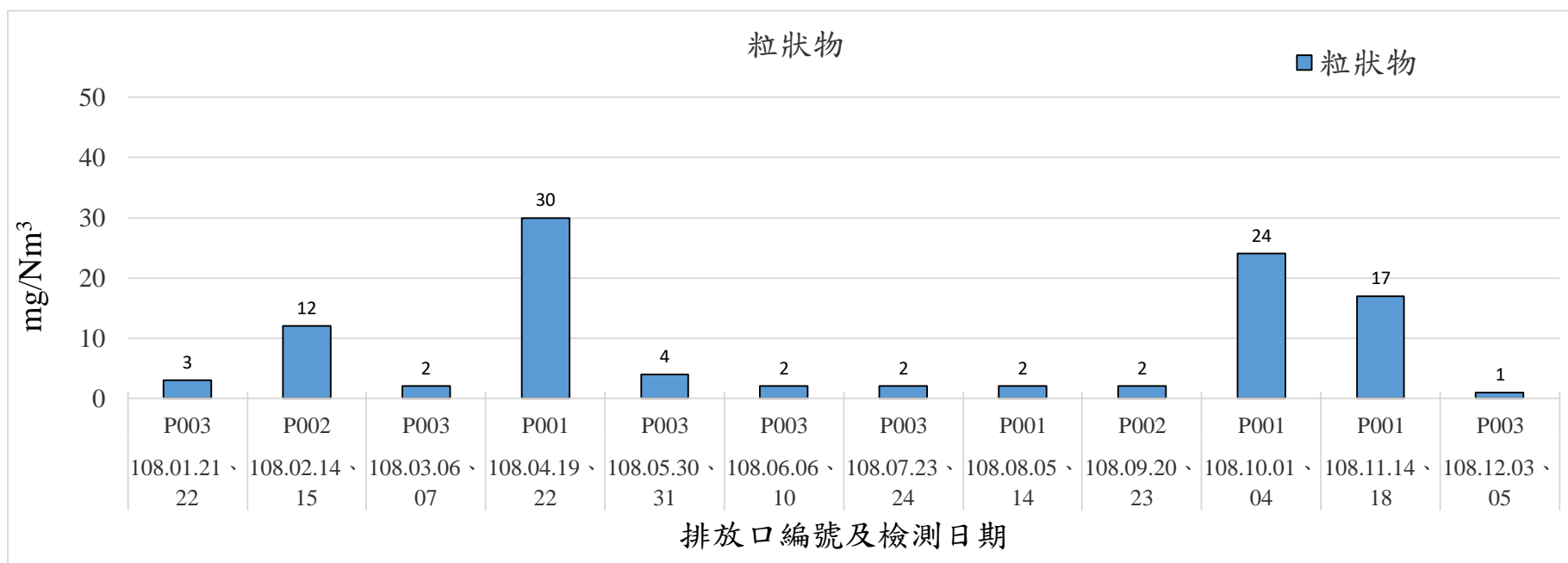
108年1月-108年12月煙道廢氣檢測結果-粒狀物
