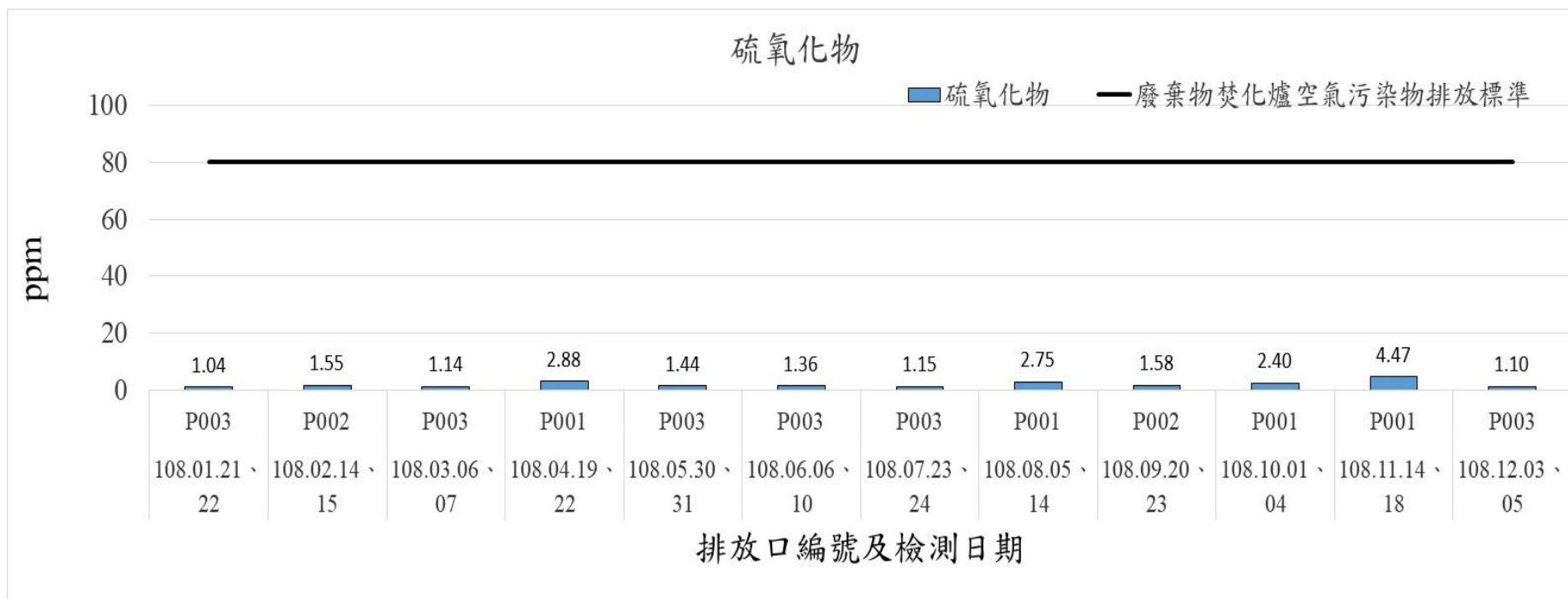
108年1月-108年12月煙道廢氣檢測結果-硫氧化物
