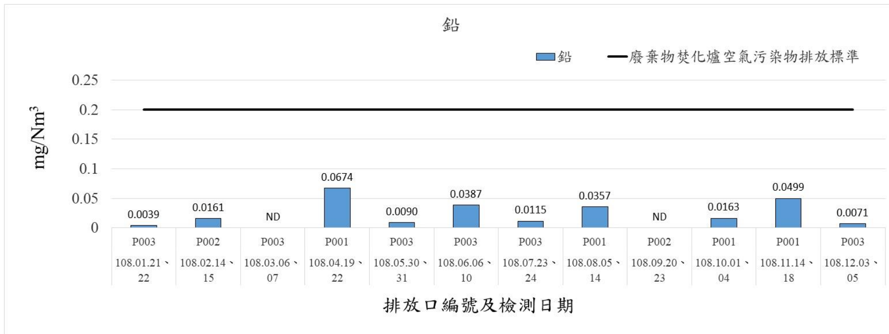
108年1月-108年12月煙道廢氣檢測結果-鉛
