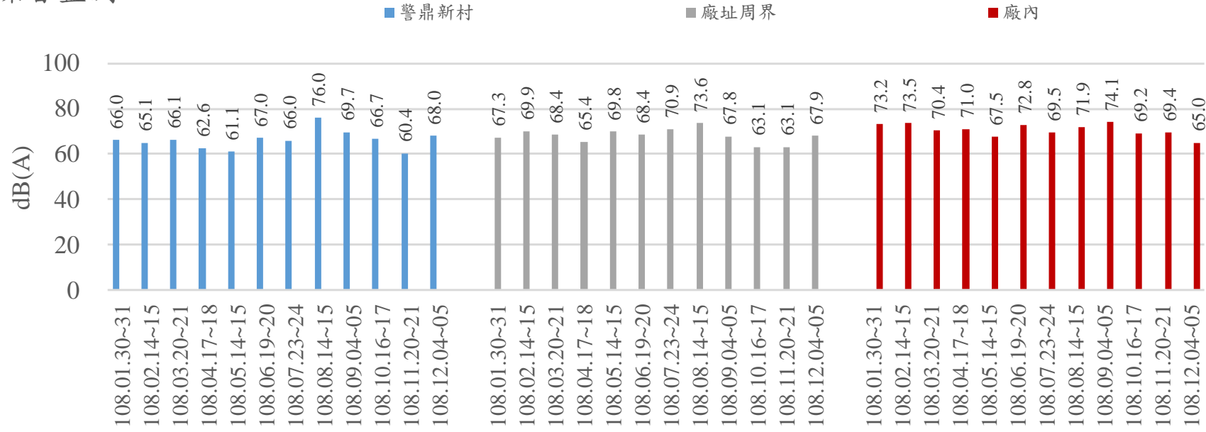
108年1月-108年12月噪音監測(Ldn)
