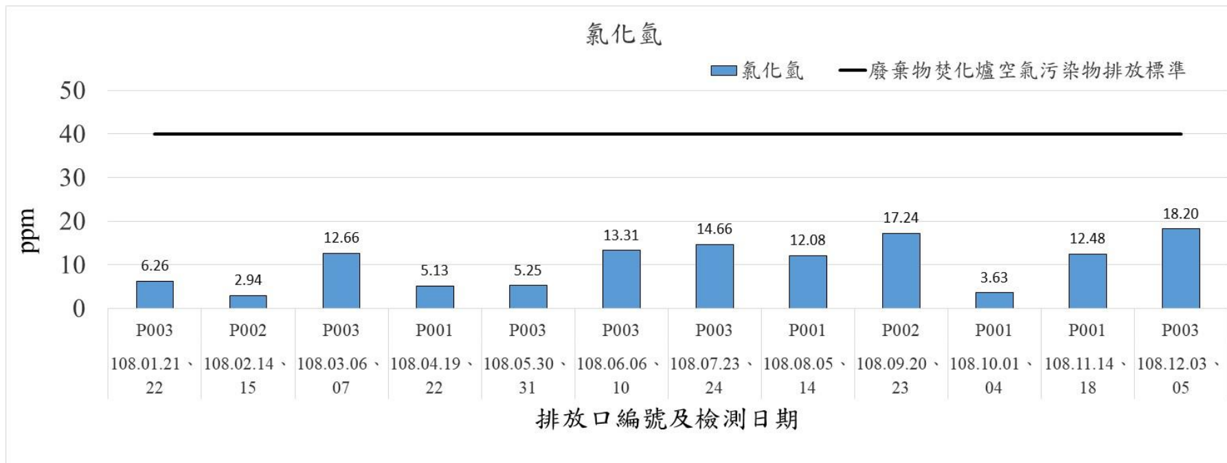
108年1月-108年12月煙道廢氣檢測結果-氯化氫
