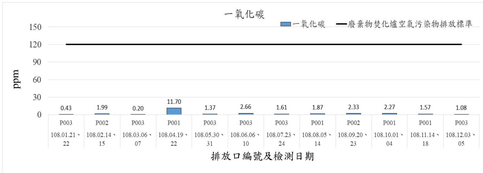
108年1月-108年12月煙道廢氣檢測結果-一氧化碳
