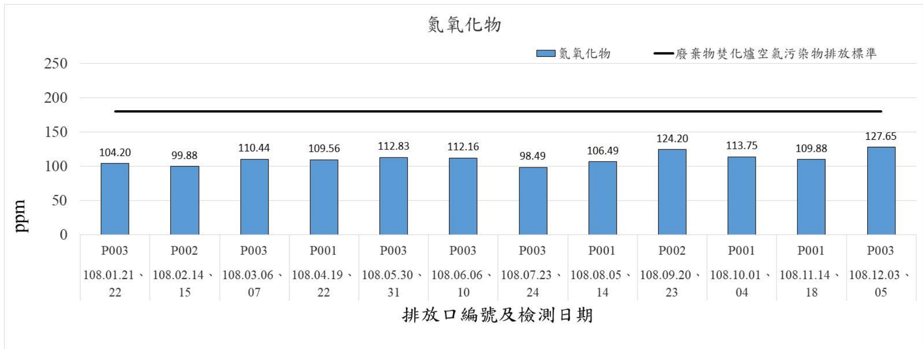
108年1月-108年12月煙道廢氣檢測結果-氮氧化物
