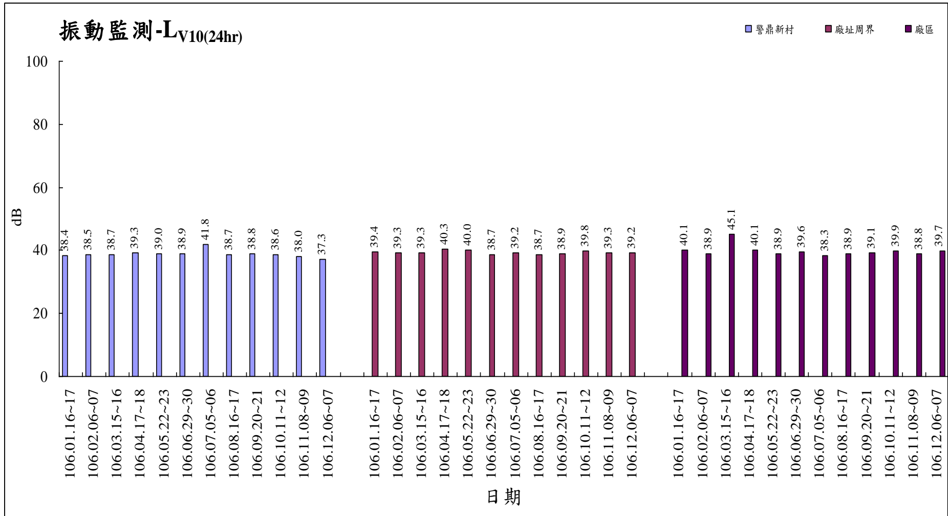
106年1月-106年12月振動監測(L V10 (24hr))
