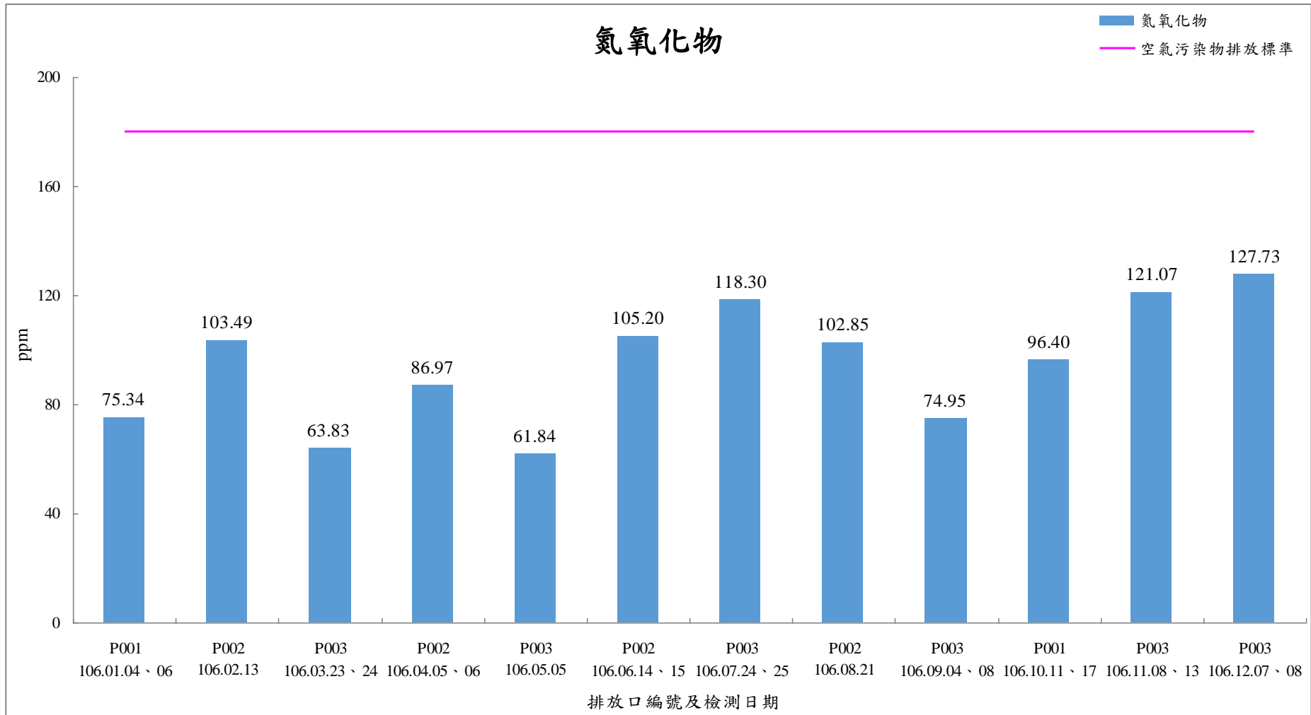
106年1月-106年12月煙道廢氣檢測結果-氮氧化物
