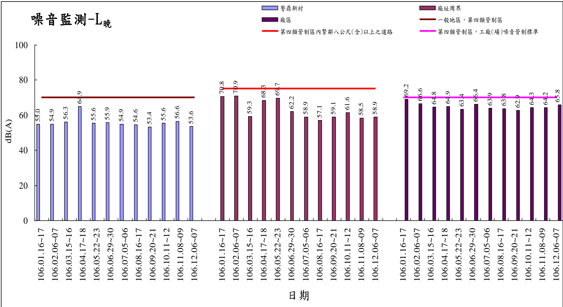
106年1月-106年12月噪音監測(L 晚 )
