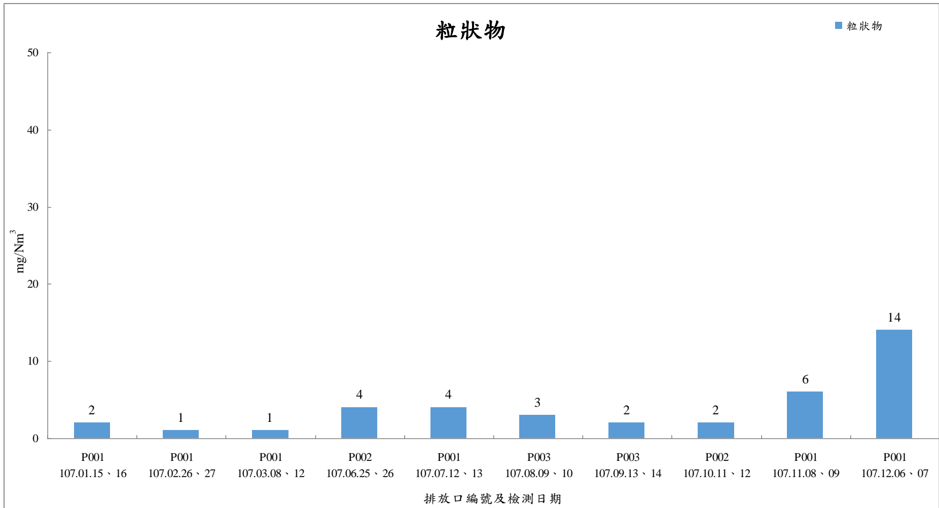
107年1月-107年12月煙道廢氣檢測結果-粒狀物
