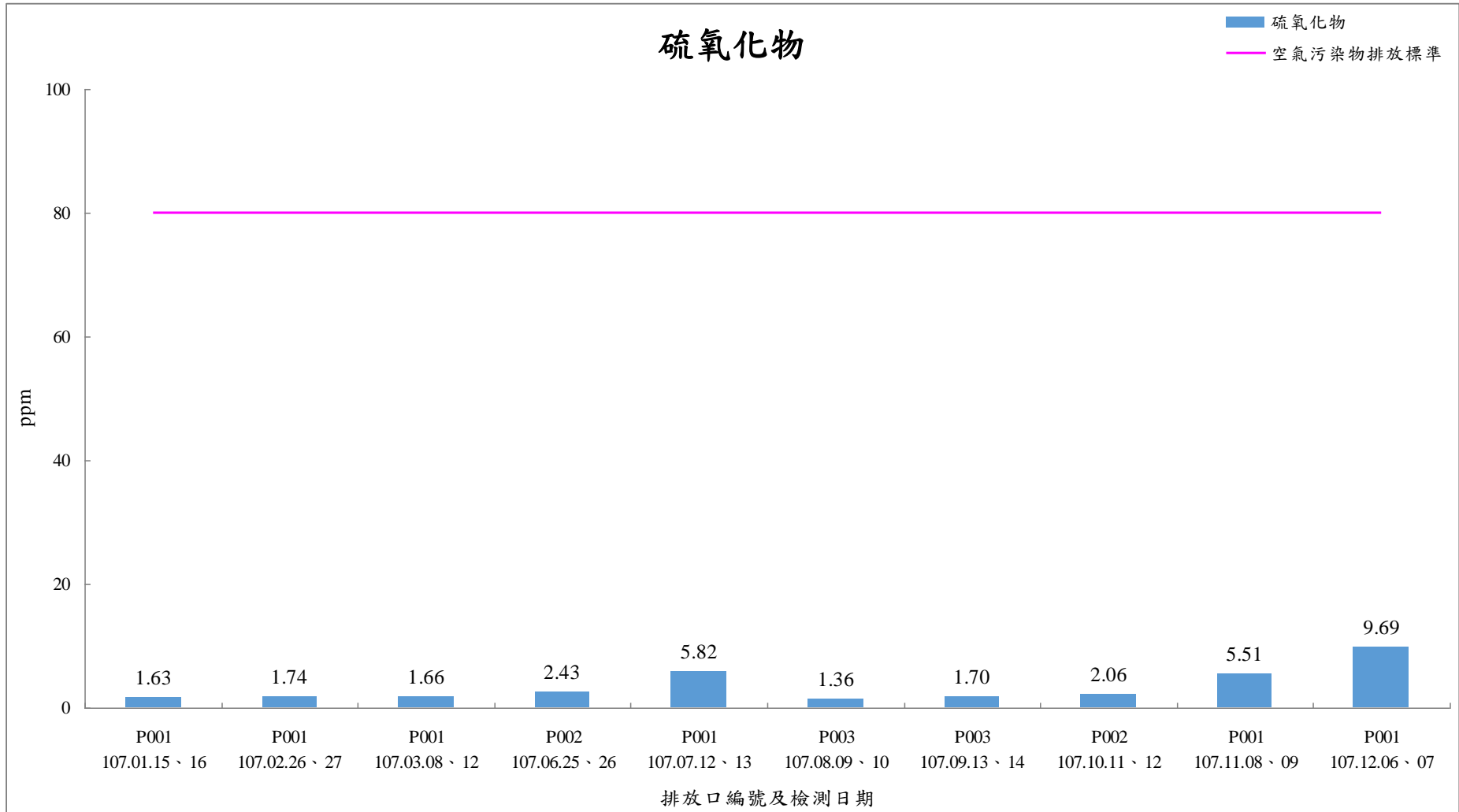
107年1月-107年12月煙道廢氣檢測結果-硫氧化物
