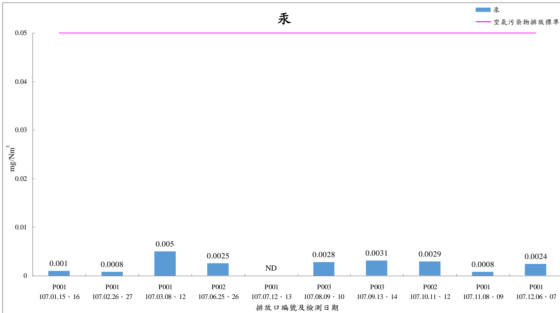
107年1月-107年12月煙道廢氣檢測結果-汞
