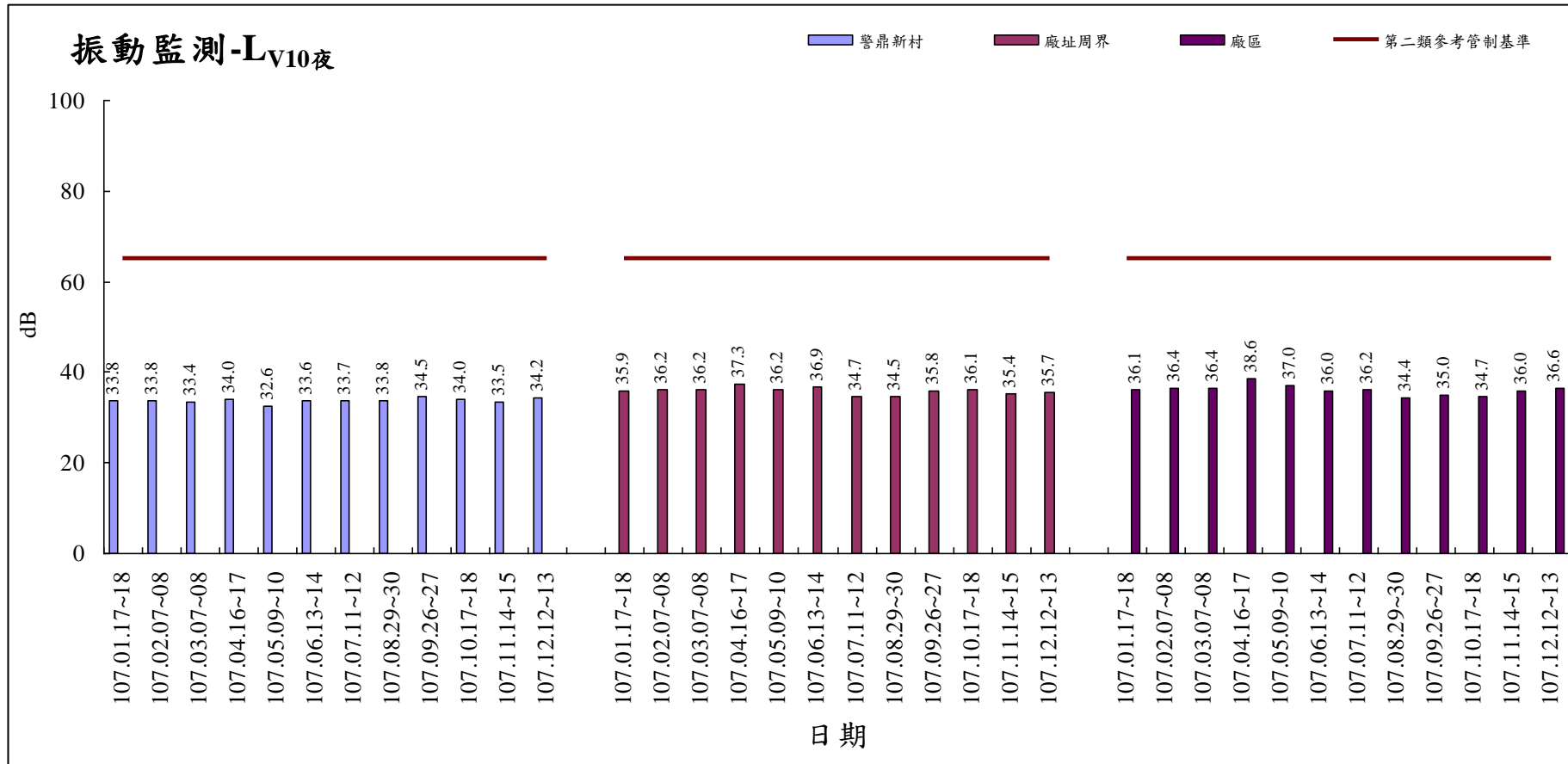
107年1月-107年12月振動監測(L V10 夜)
