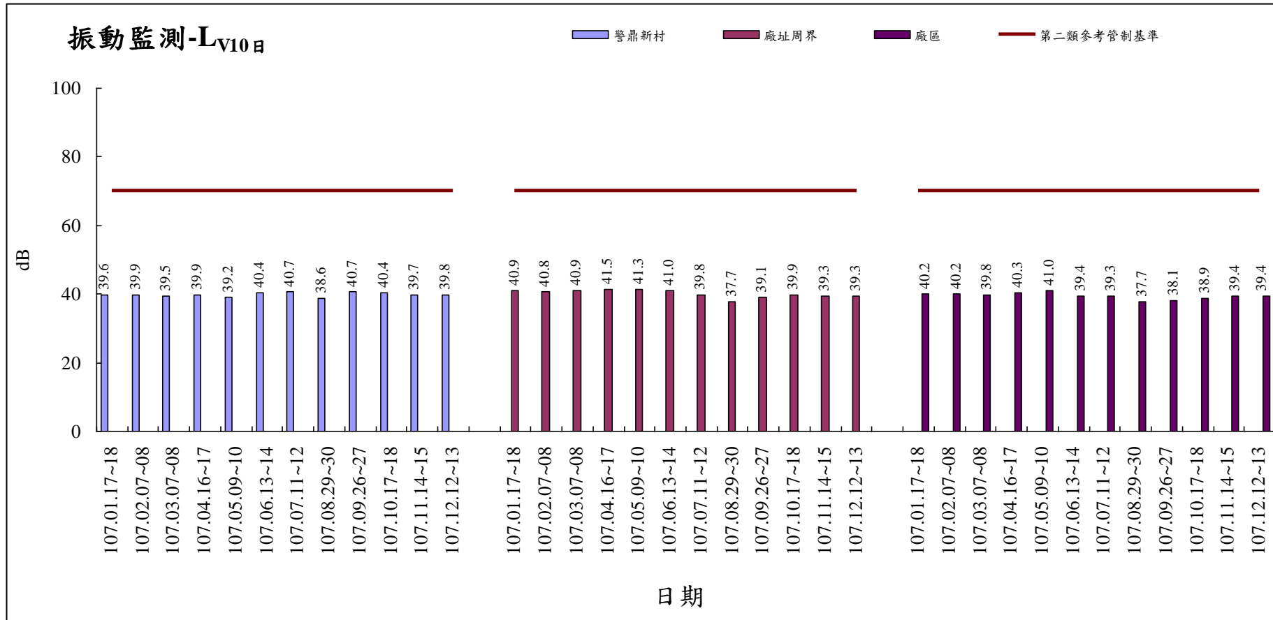
107年1月-107年12月振動監測(L V10日 )
