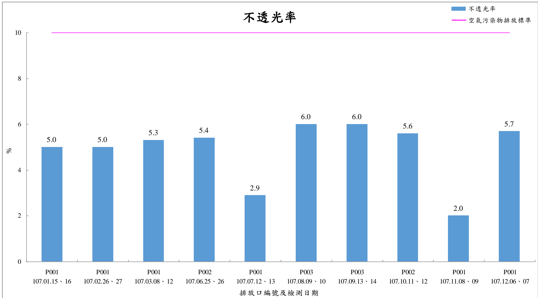
107年1月-107年12月煙道廢氣檢測結果-不透光率
