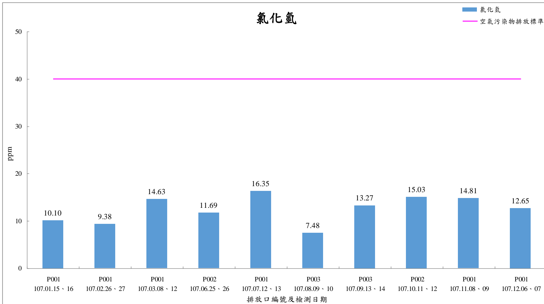
107年1月-107年12月煙道廢氣檢測結果-氯化氫
