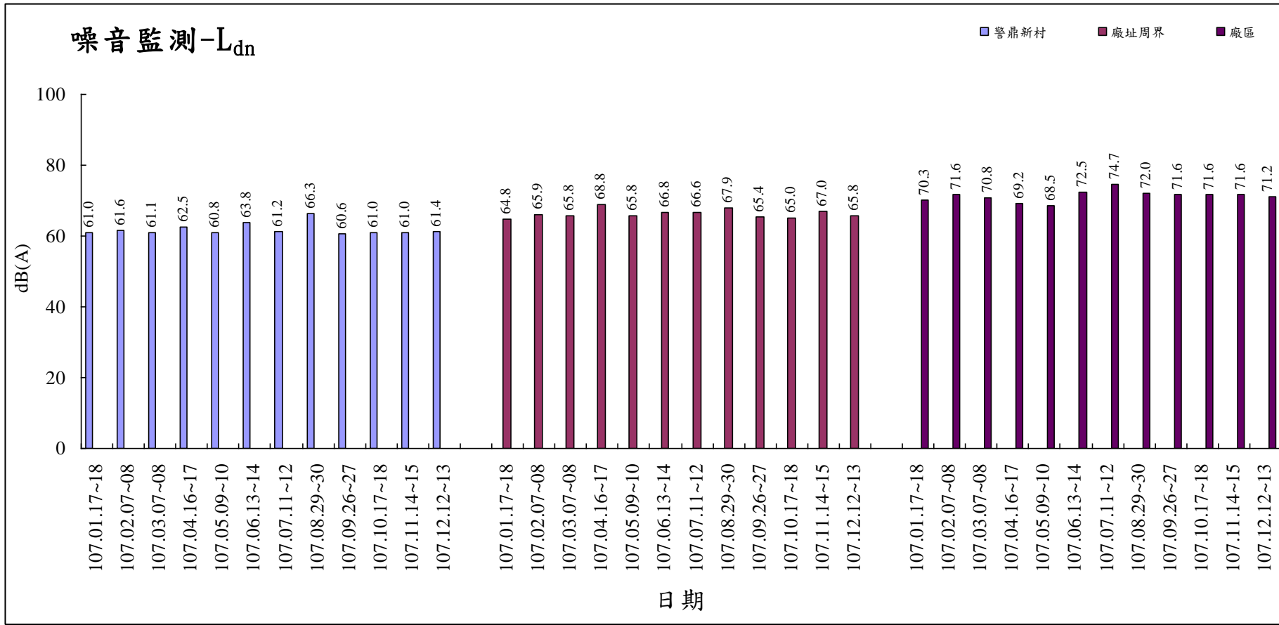
107年1月-107年12月噪音監測(L dn )
