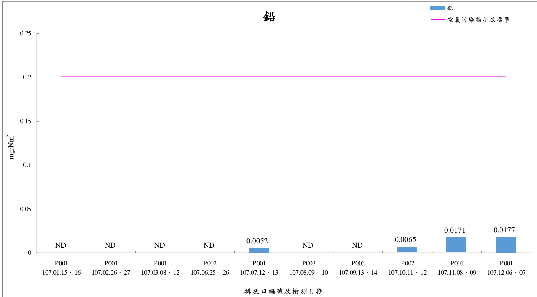
107年1月-107年12月煙道廢氣檢測結果-鉛
