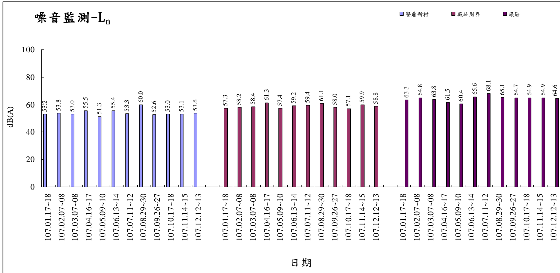
107年1月-107年12月噪音監測(L n )
