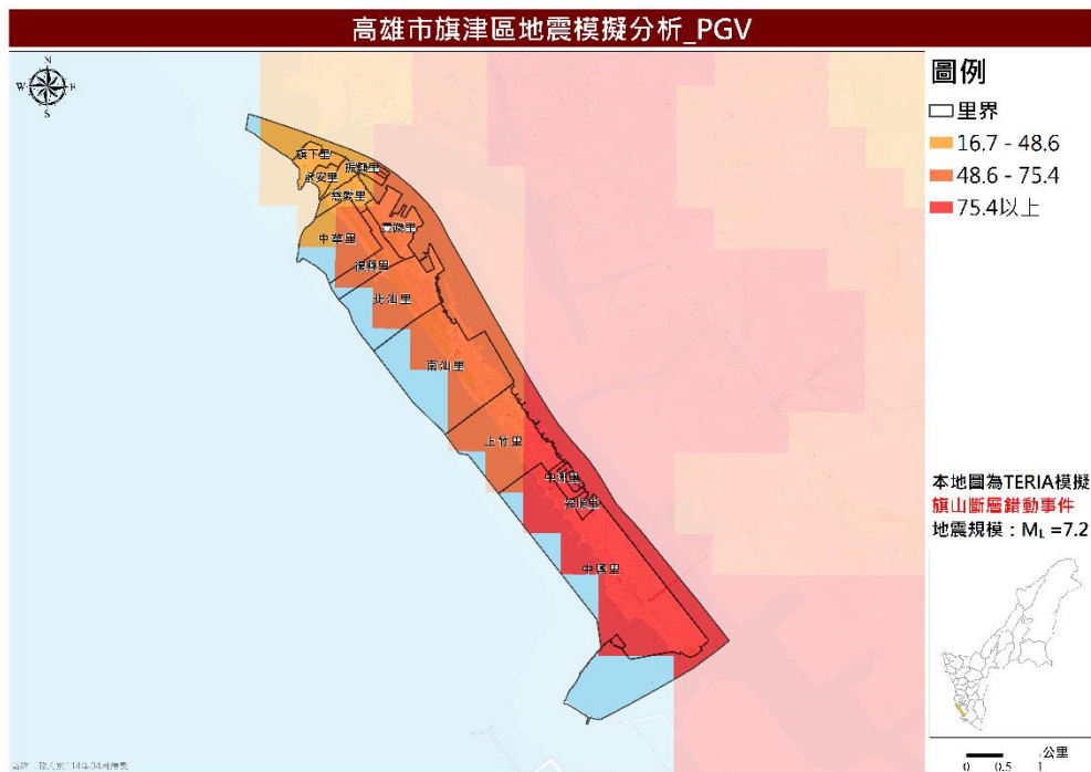
圖 10 旗山斷層錯動事件最大地表速度值 (PGV) 分布圖
