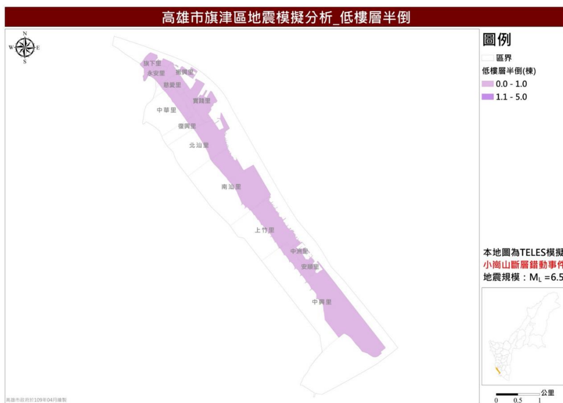
圖 20 小崗山斷層錯動事件低樓層半倒棟數推估圖
