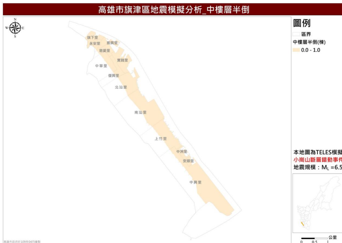
圖 21 小崗山斷層錯動事件中樓層半倒棟數推估圖
