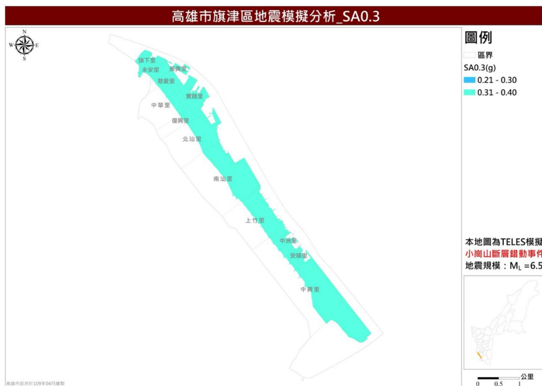
圖 14 小崗山斷層錯動事件短周期譜加速度（SA0.3）分布圖
