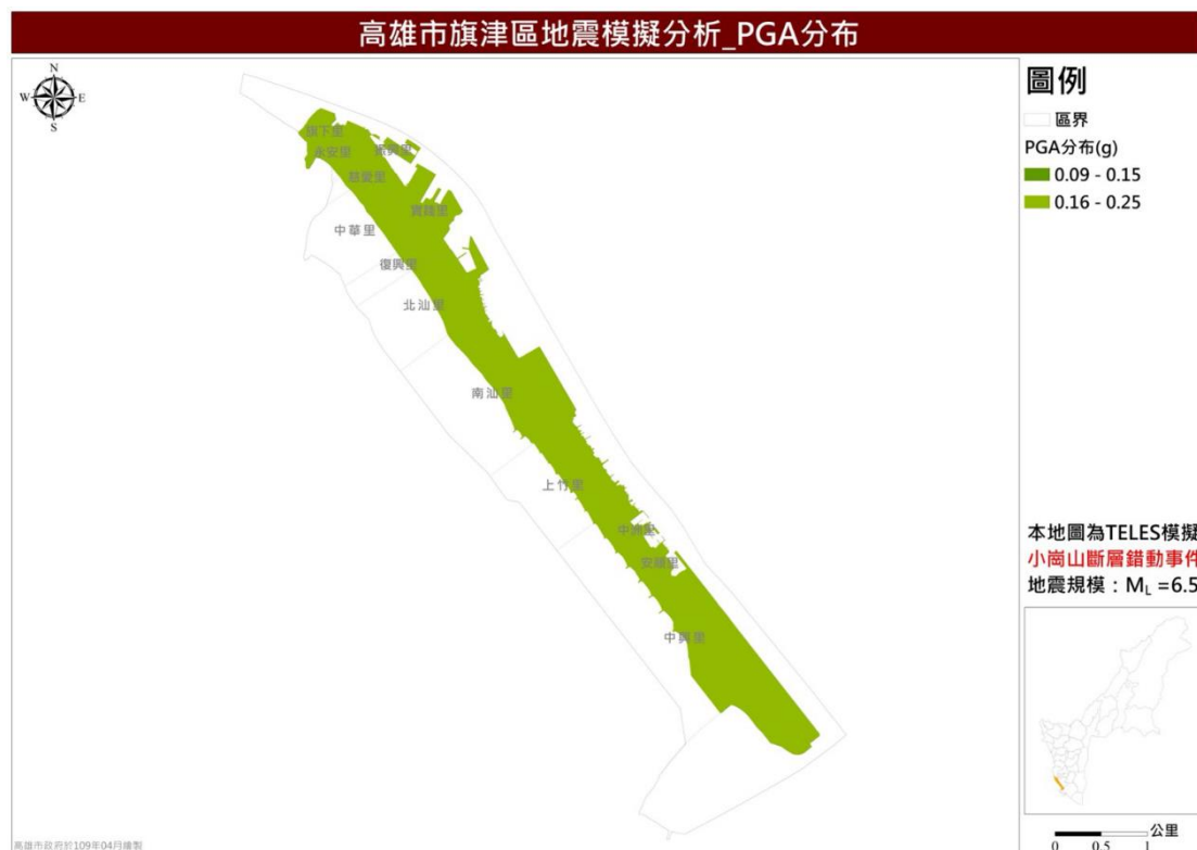
圖 13 小崗山斷層錯動事件最大地表加速度（PGA）分布圖
