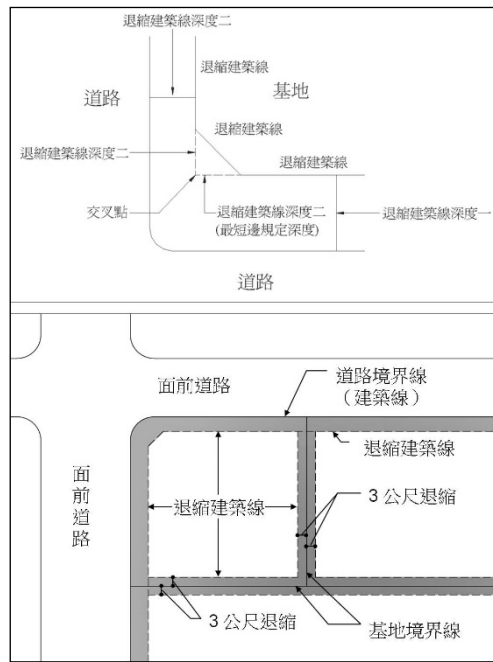
建築基地退縮示意圖
