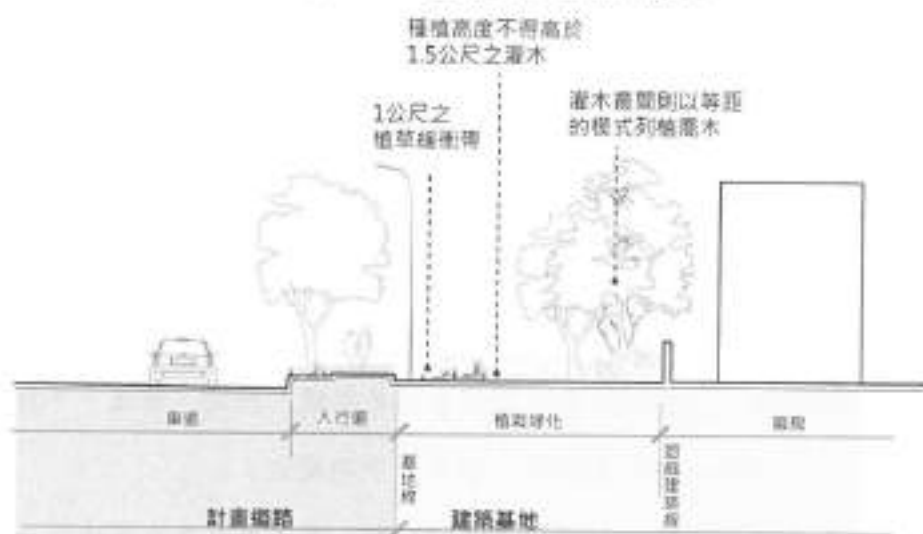
圖 5-6 臨計畫道路之建築基地退縮示意圖
