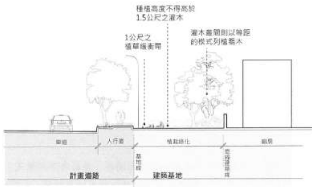
臨計畫道路之建築基地退縮示意
