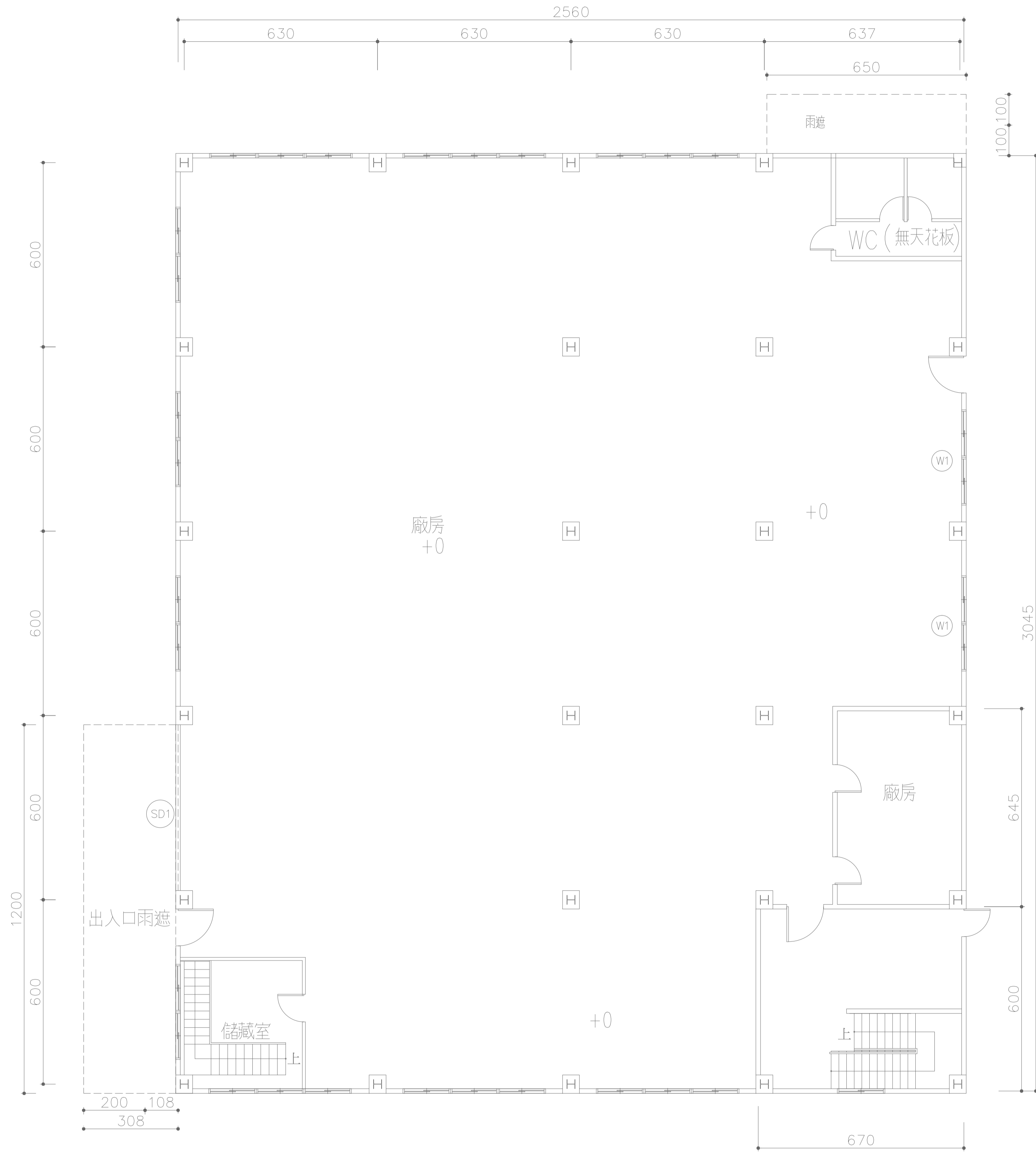
一層平面圖
