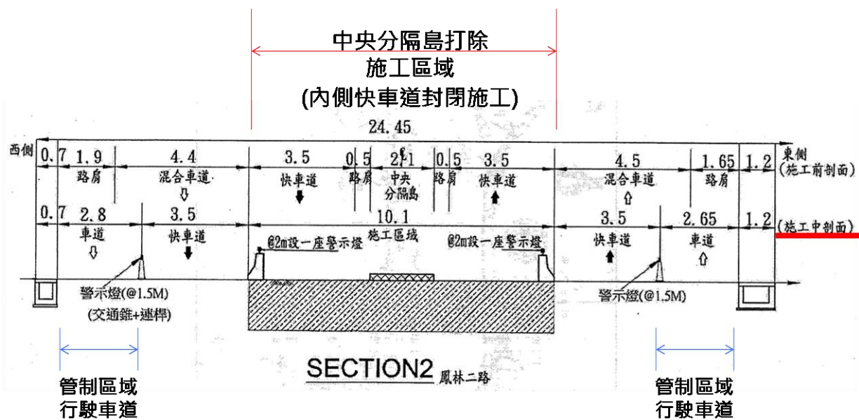
圖 3 改道及道路封閉示意圖
