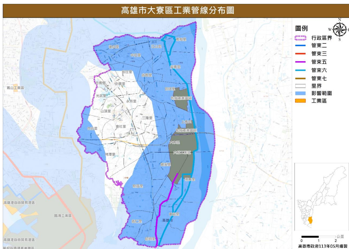
圖 29 大寮區工業管線分布圖
