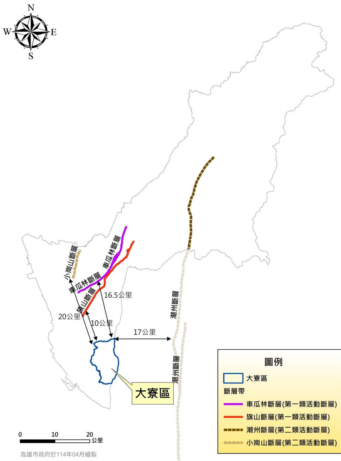
圖 12 大寮區與高雄市斷層分布相對位置圖
