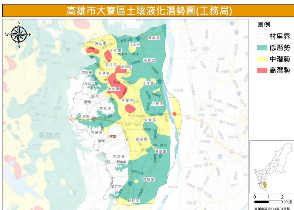
圖 25 大寮區土壤液化潛勢圖
