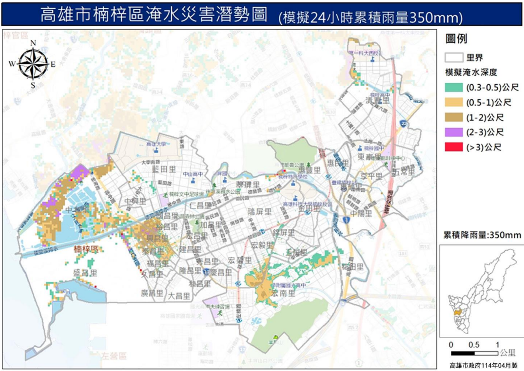
圖 8 楠梓區淹水災害潛勢圖（模擬 24 小時累積降雨量 350mm）
