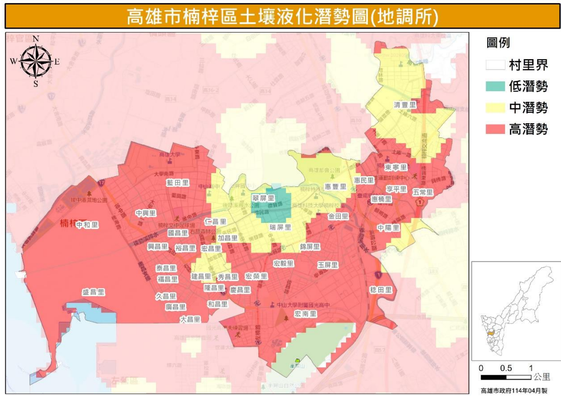
圖 26 楠梓區土壤液化潛勢圖（資料來源：地質調查及礦業管理中心）
