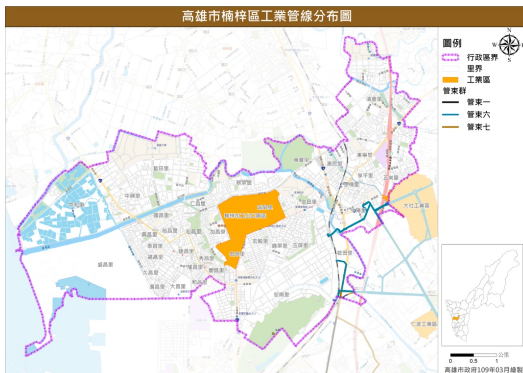
圖 33 楠梓區工業管線分布圖
