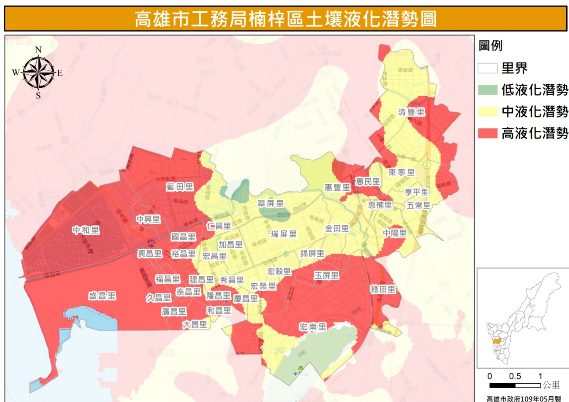
圖 28 楠梓區土壤液化潛勢圖（資料來源：高雄市政府工務局）
