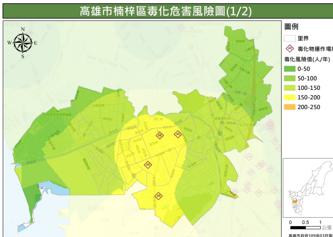
圖 30 楠梓區毒性化學物質災害危害風險潛勢圖（低機率）
