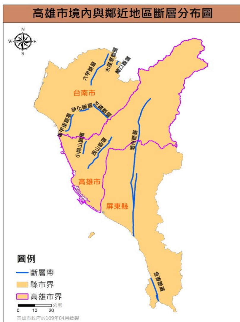
圖 12 高雄市境內與鄰近地區斷層分布圖
