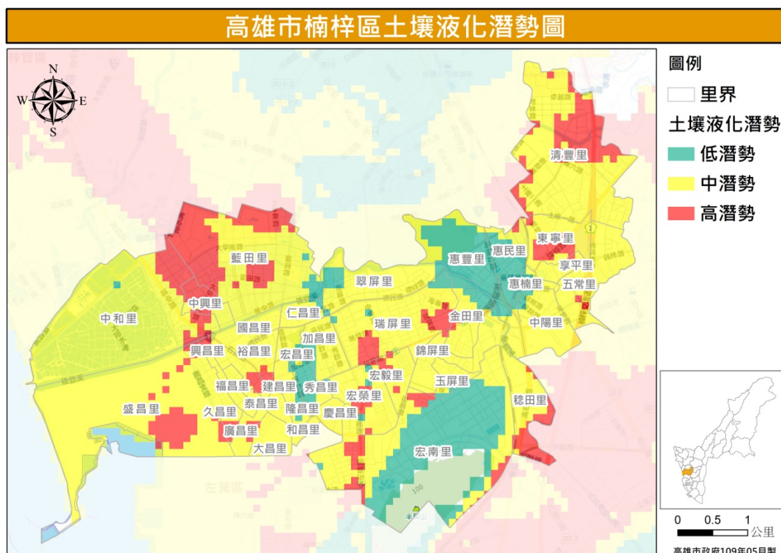
圖 27 楠梓區土壤液化潛勢圖（資料來源：經濟部中央地質調查所）
