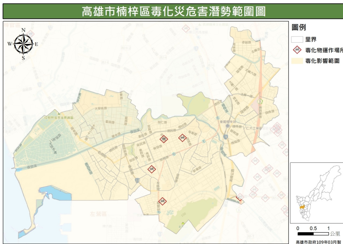
圖 29 楠梓區毒性化學物質災害危害潛勢範圍圖
