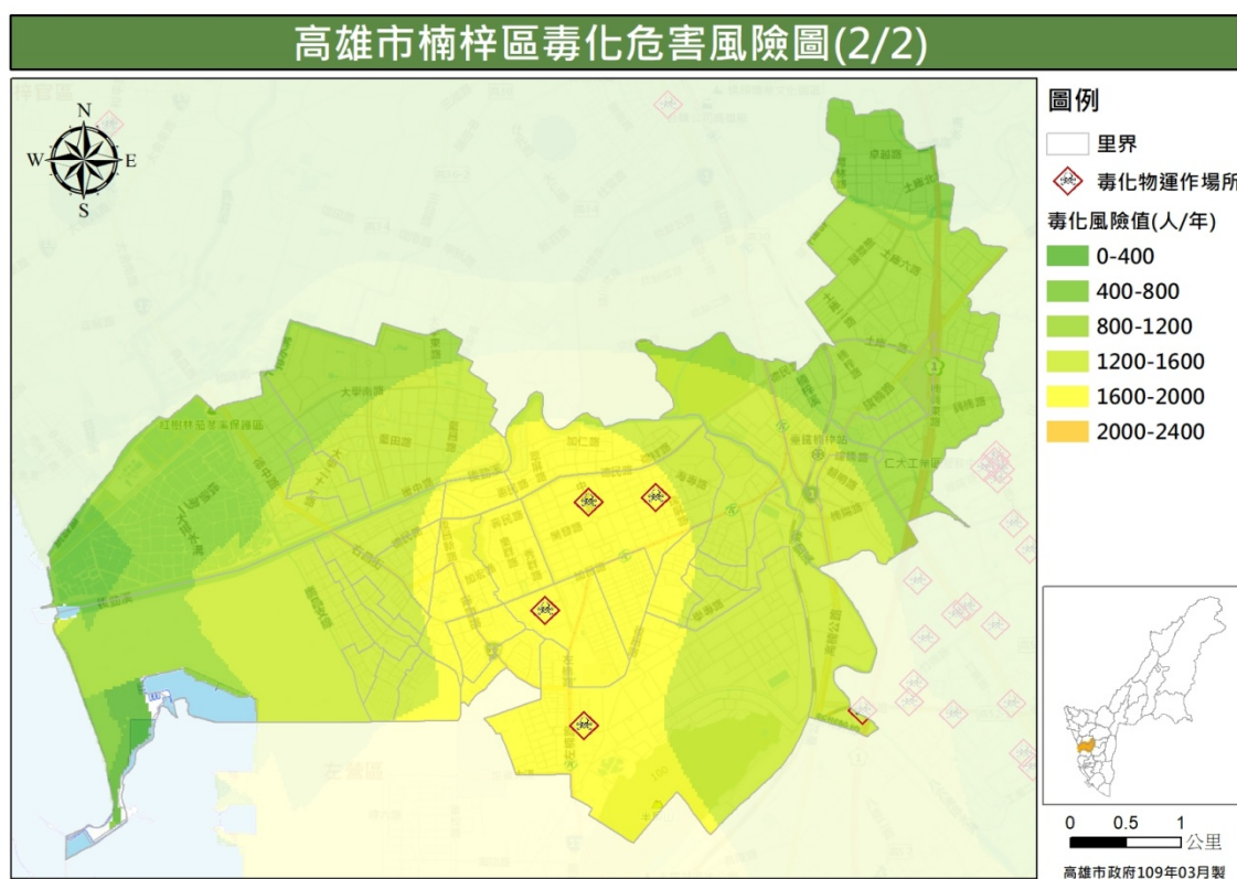
圖 31 楠梓區毒性化學物質災害危害風險潛勢圖（高機率）
