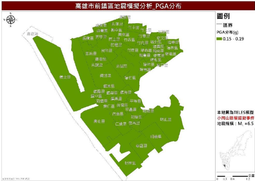
圖 15 小崗山斷層錯動事件最大地表加速度 (PGA) 分布圖
