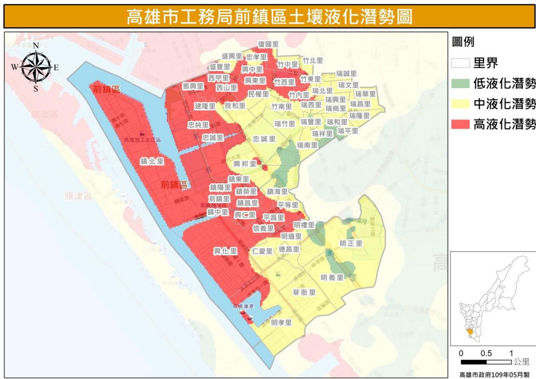
圖 29 高雄市工務局前鎮區土壤液化潛勢圖 (資料來源：高雄市政府工務局)
