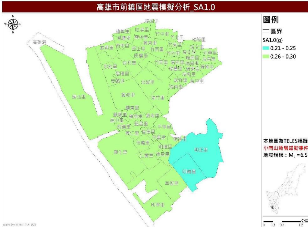
圖 17 小崗山斷層錯動事件長周期譜加速度 (SA1.0) 分布圖
