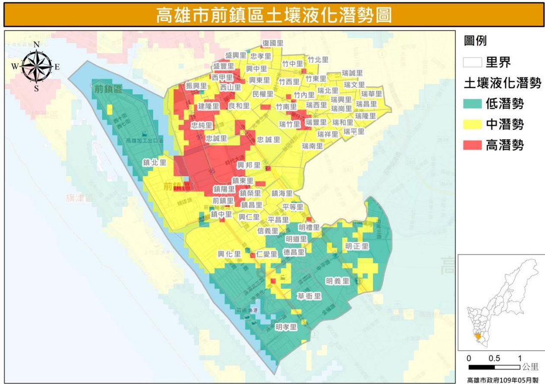
圖 28 高雄市前鎮區土壤液化潛勢圖 (資料來源：經濟部中央地質調查所)
