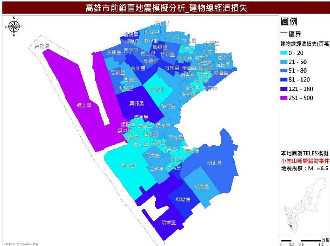
圖 18 小崗山斷層錯動事件建物總經濟損失分布圖
