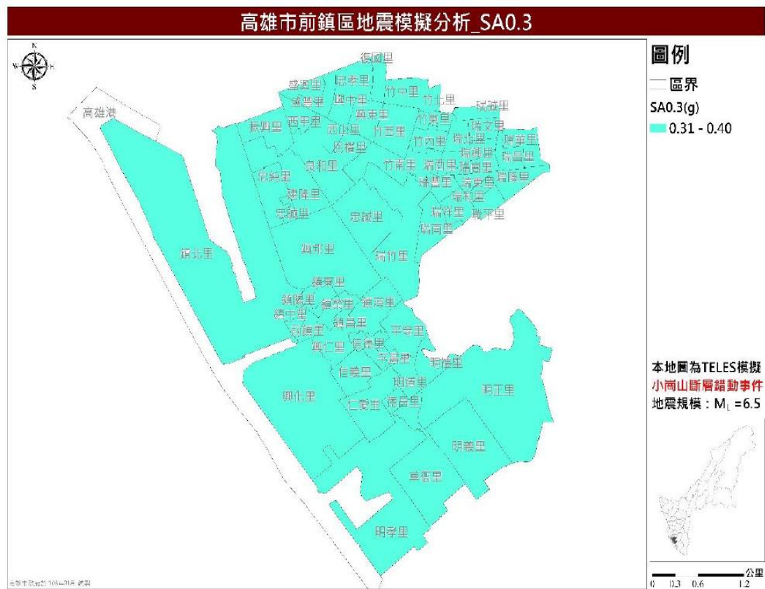
圖 16 小崗山斷層錯動事件短周期譜加速度 (SA0.3) 分布圖
