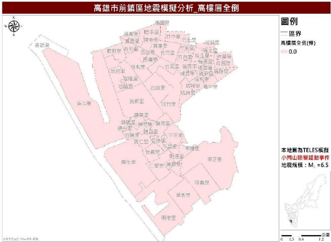
圖 21 小崗山斷層錯動事件高樓層全倒棟數推估圖
