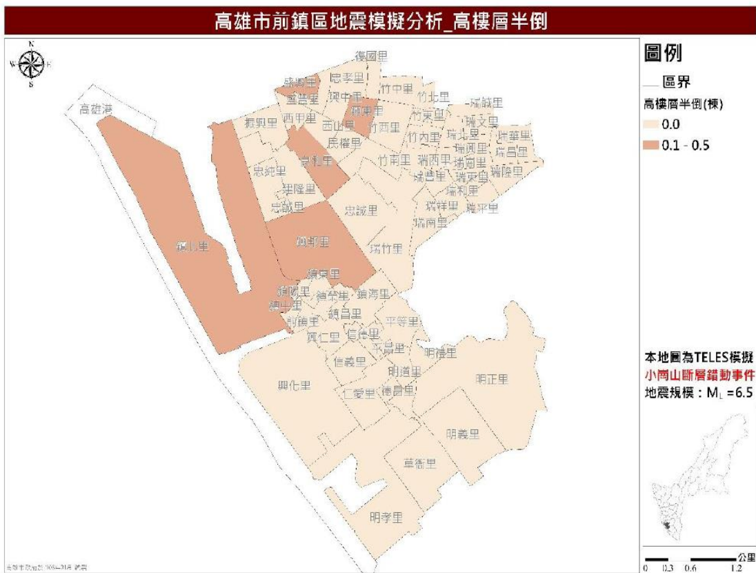
圖 24 小崗山斷層錯動事件高樓層半倒棟數推估圖
