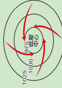
北半球氣旋
