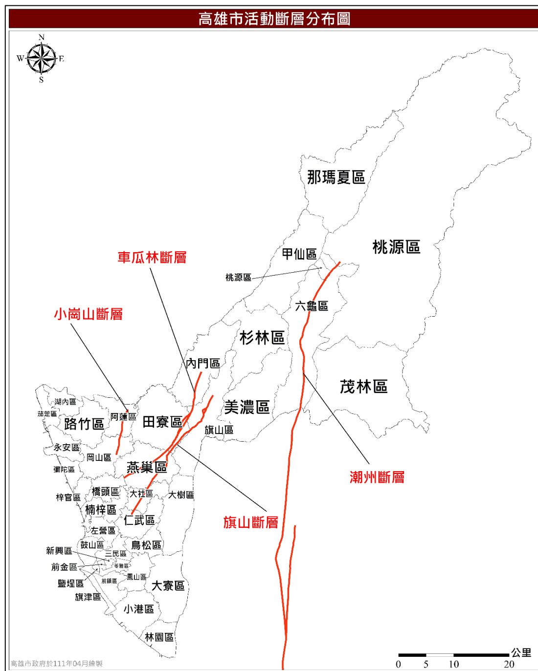
圖 12 高雄市境內與鄰近地區斷層分布圖
