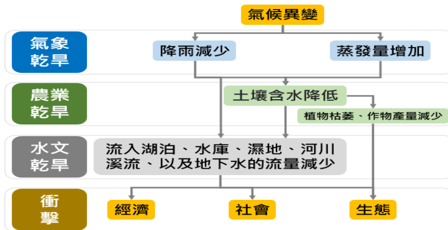
圖 34 不同乾旱類型之相互關係及衝擊
