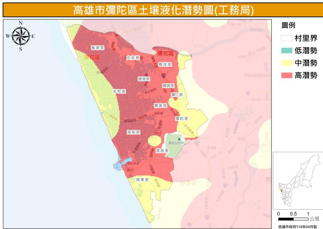
彌陀區土壤液化潛勢圖(工務局)
