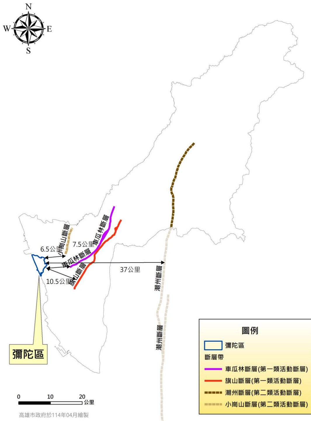
彌陀區斷層距離圖
