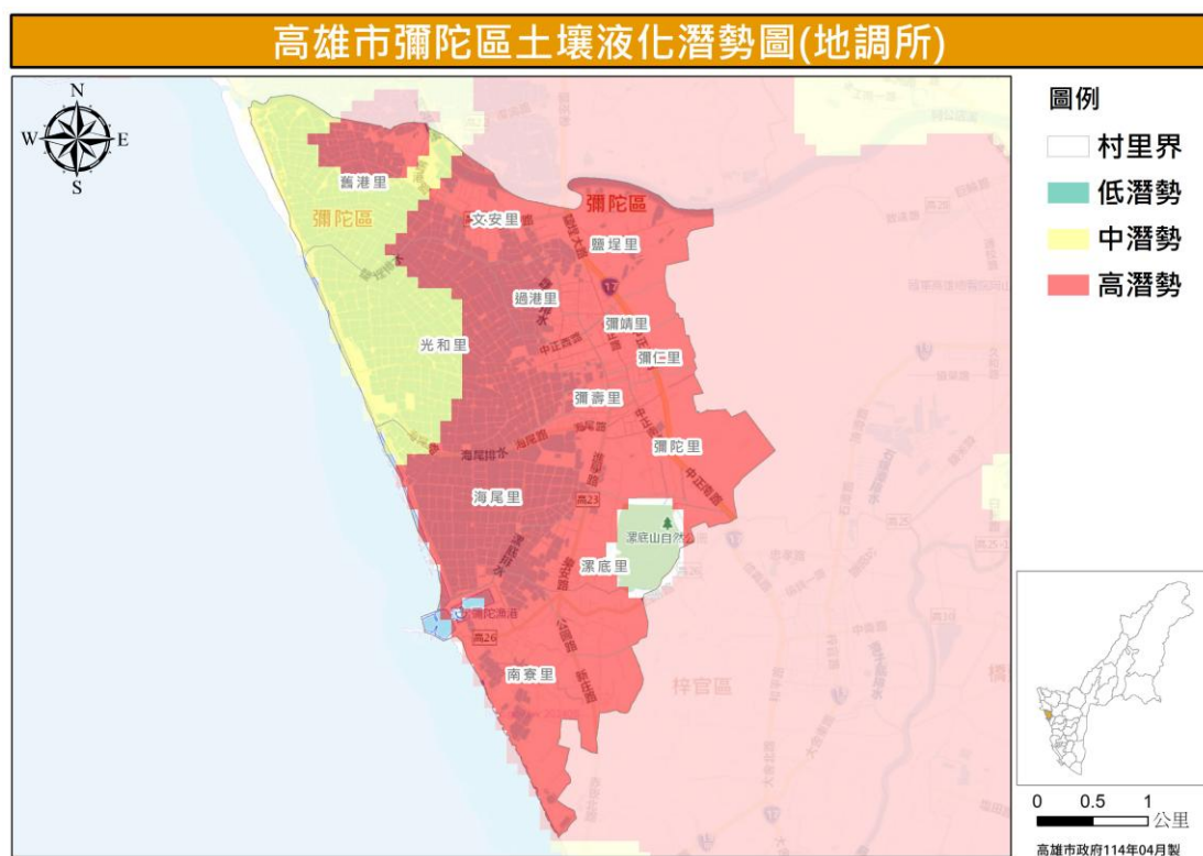
彌陀區土壤液化潛勢圖(地調所)
