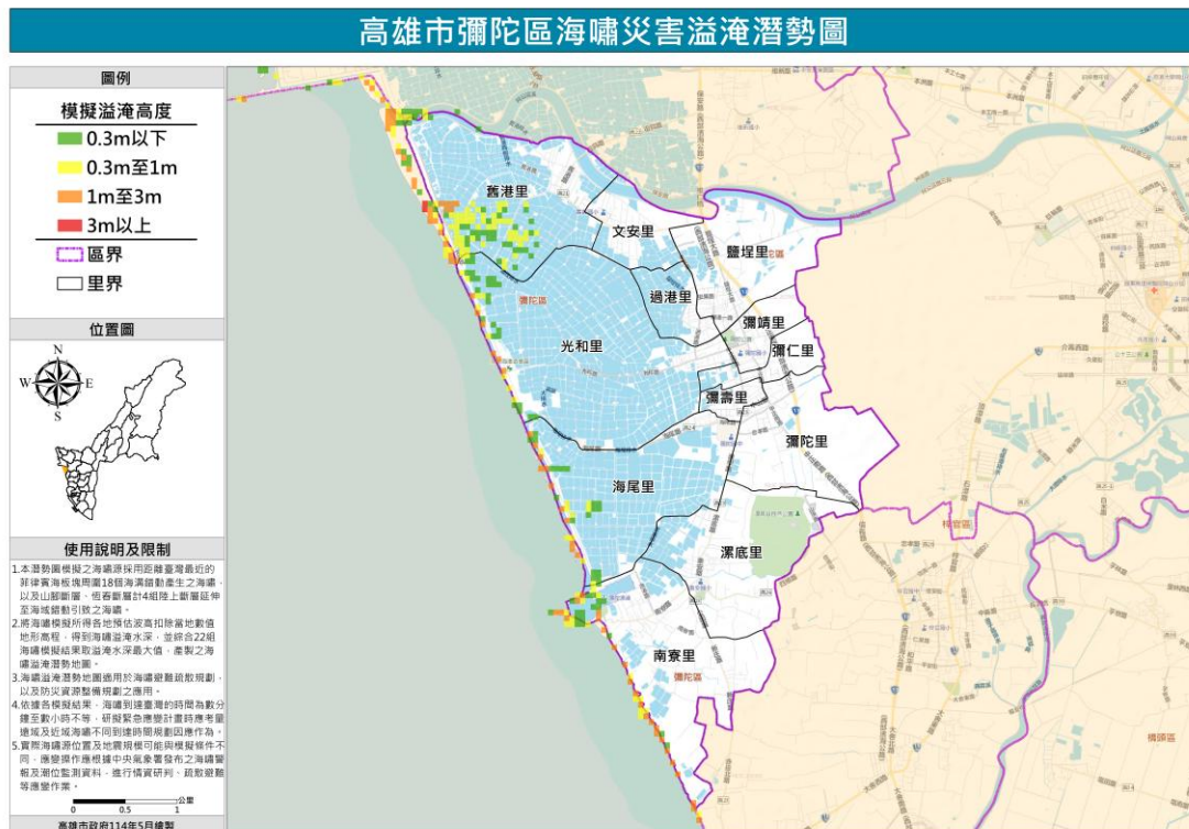
彌陀區海嘯災害溢淹潛勢圖
