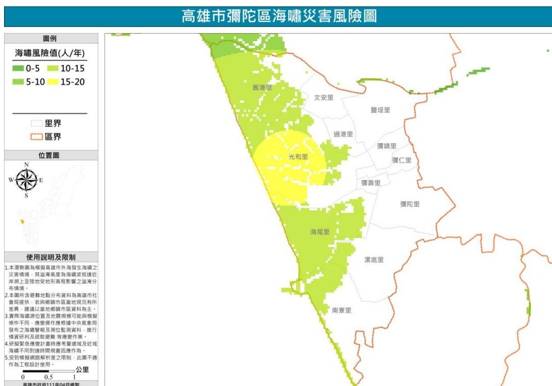
圖 27 彌陀區海嘯災害風險圖
