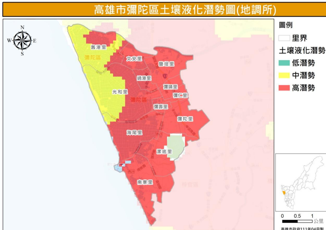
圖 24 彌陀區土壤液化潛勢圖（資料來源：經濟部中央地質調查所）
