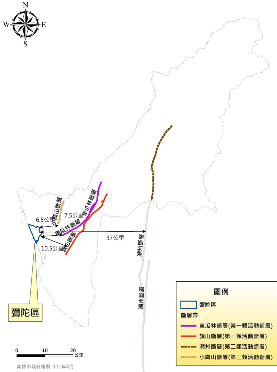
圖 11 彌陀區與高雄市斷層分布相對位置圖
