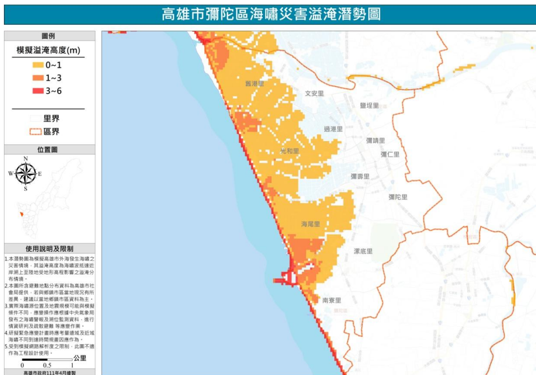
圖 26 彌陀區海嘯災害溢淹潛勢圖
