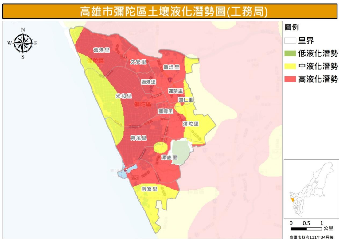
圖 25 彌陀區土壤液化潛勢圖（資料來源：高雄市政府工務局）
