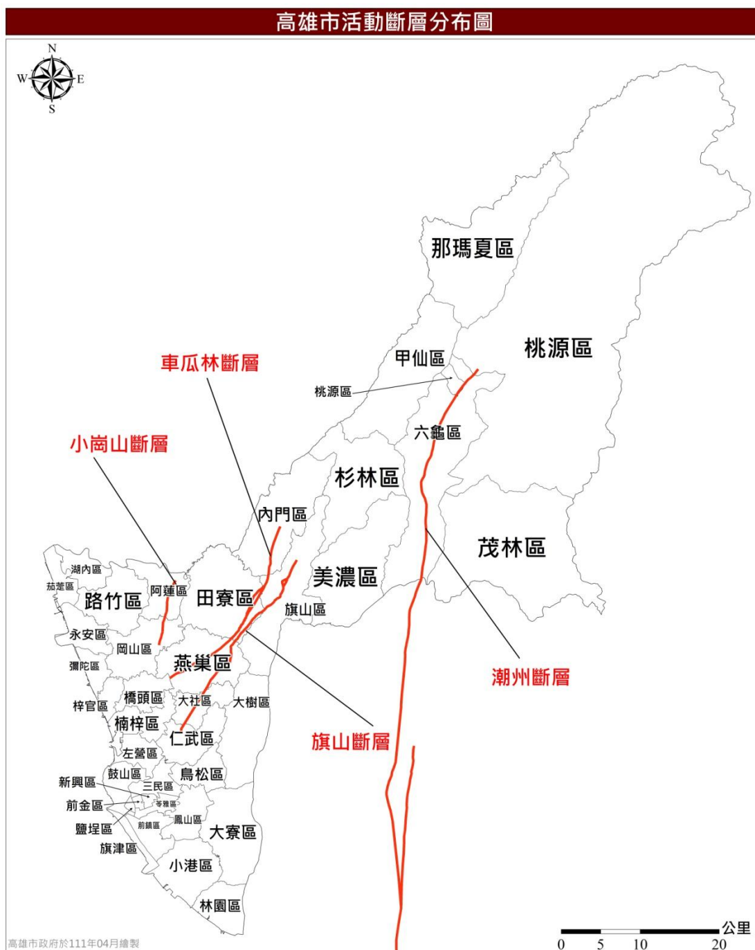
圖 10 高雄市境內與鄰近地區斷層分布圖
