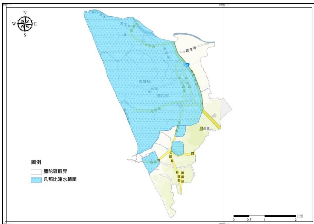
圖 9 彌陀區凡那比颱風淹水範圍分布圖
