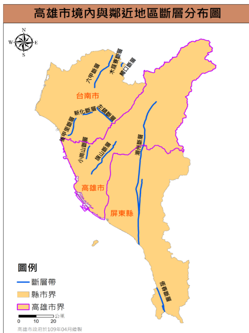
圖 10 高雄市境內與鄰近地區斷層分布圖
