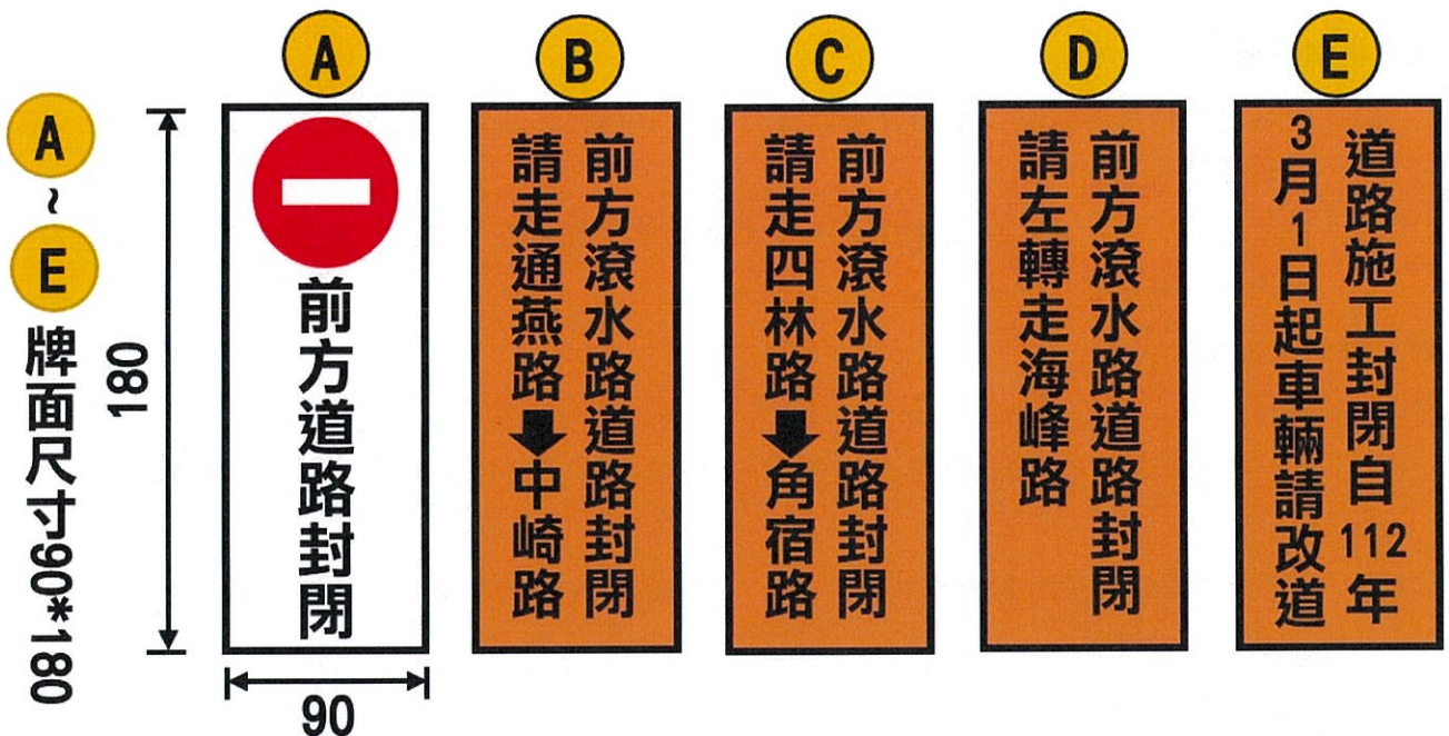
圖 2 改道牌面(尺寸皆為 90*180CM)
