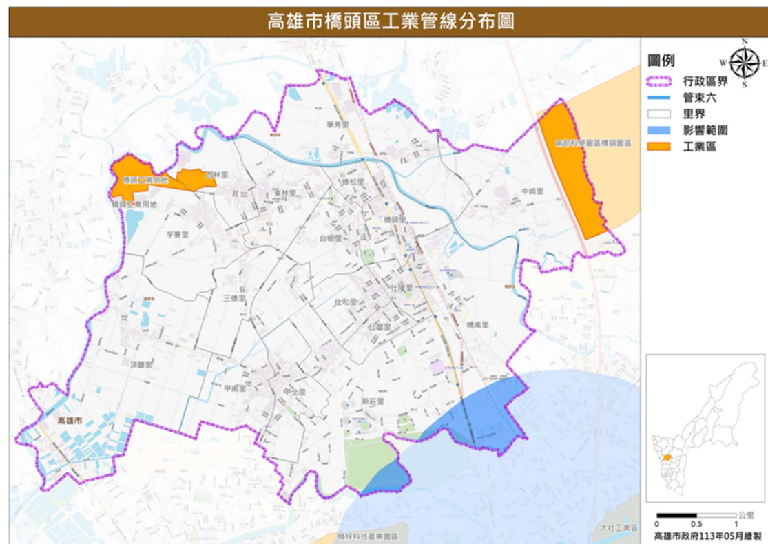
圖 36 橋頭區工業管線分布圖
