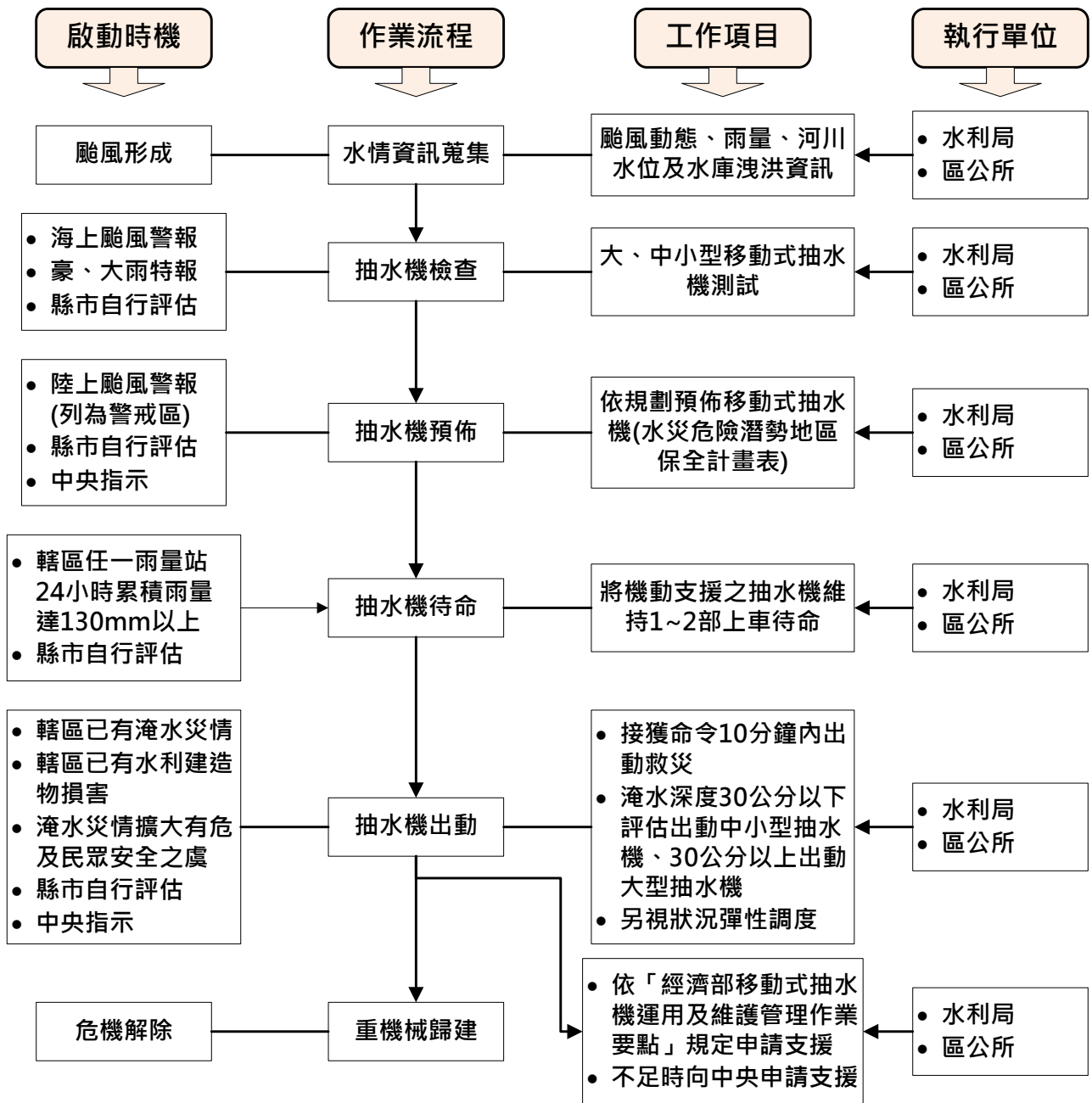
附圖八、移動式抽水機運用作業流程
