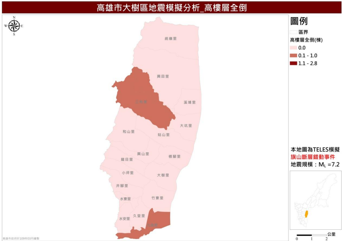
圖 18 小崗山斷層錯動事件高樓層全倒棟數推估圖
