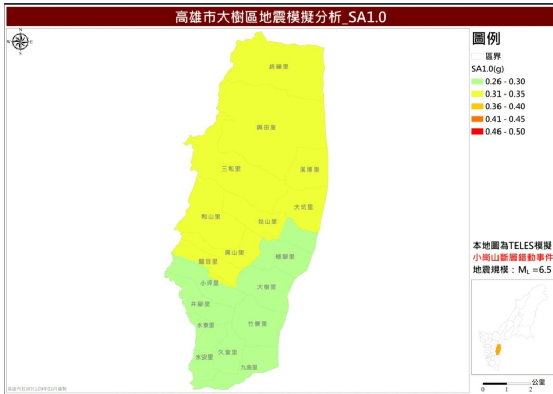
圖 14 小崗山斷層錯動事件長周期譜加速度 (SA1.0) 分布圖
