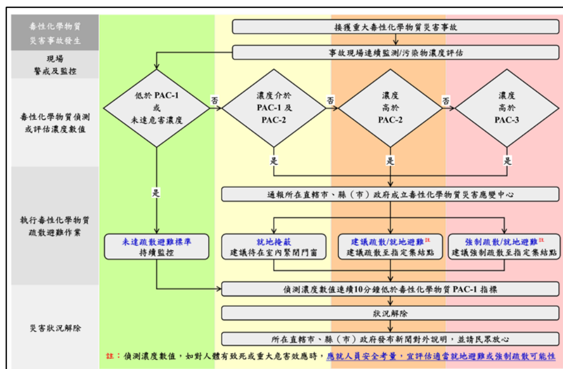
圖 22 毒性化學物質災害疏散避難計畫作業流程圖
