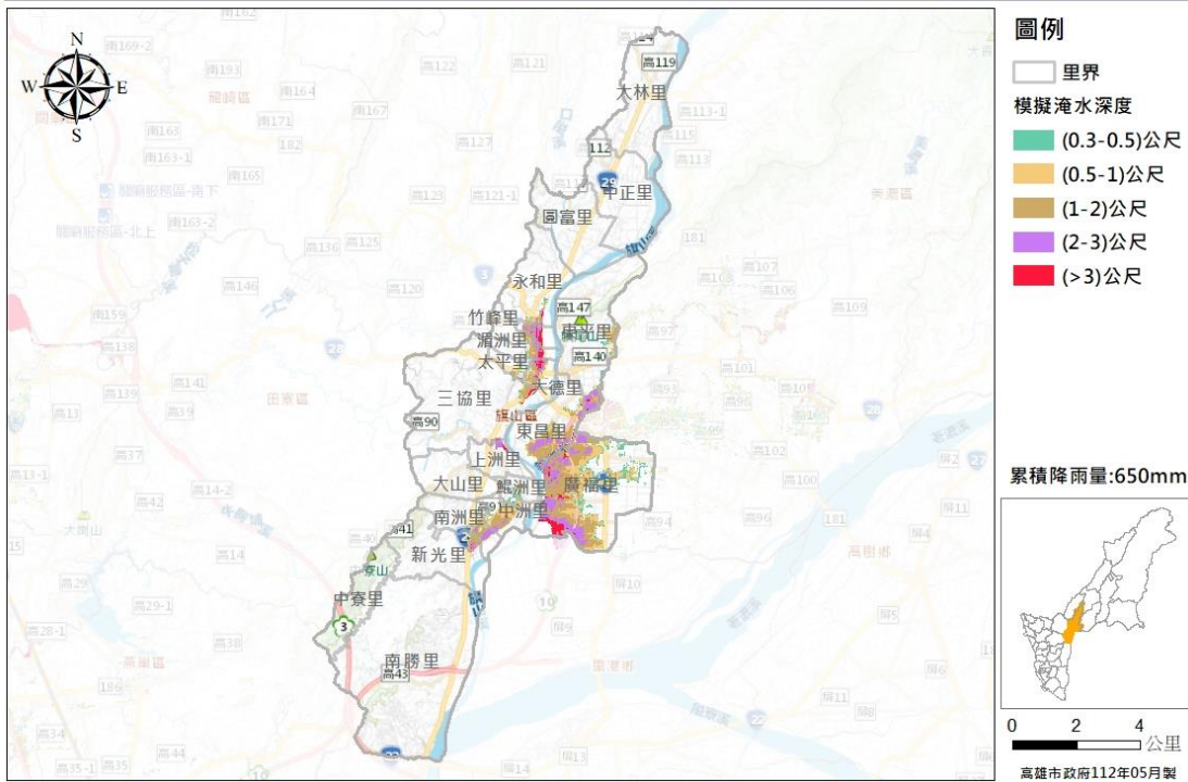
圖 5 旗山區淹水災害潛勢圖 (模擬 24 小時累積降雨量 650mm)
