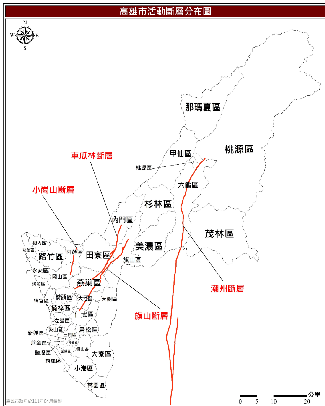
圖 13 高雄市境內與鄰近地區斷層分布圖
