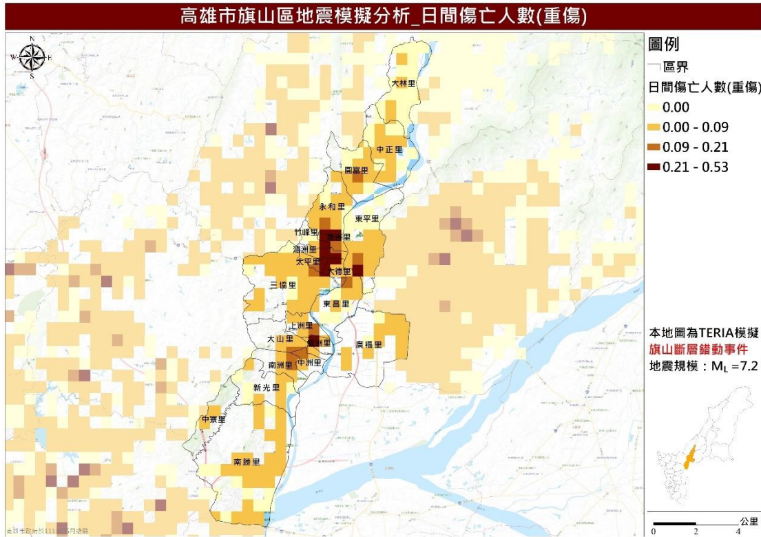
圖 26 旗山斷層錯動事件日間重傷人數推估圖
