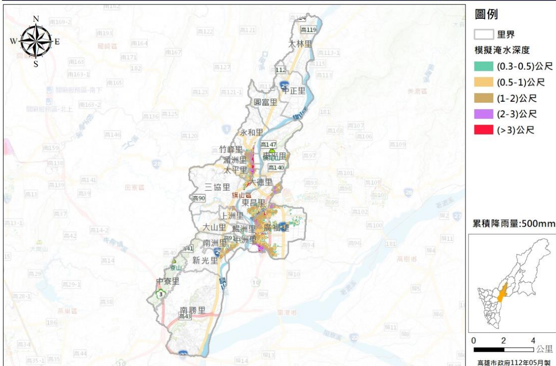
圖 6 旗山區淹水災害潛勢圖 (模擬 24 小時累積降雨量 500mm)
