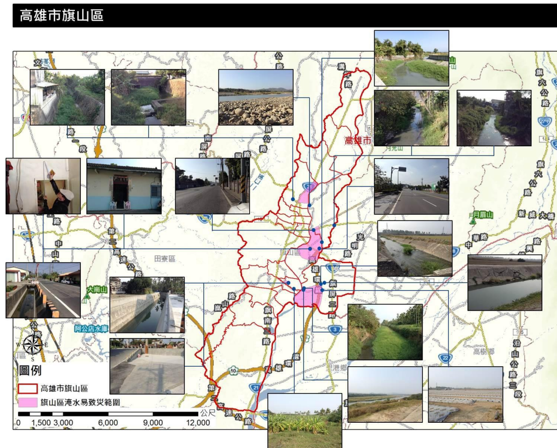
圖 8 旗山區淹水易致災區域分布圖
