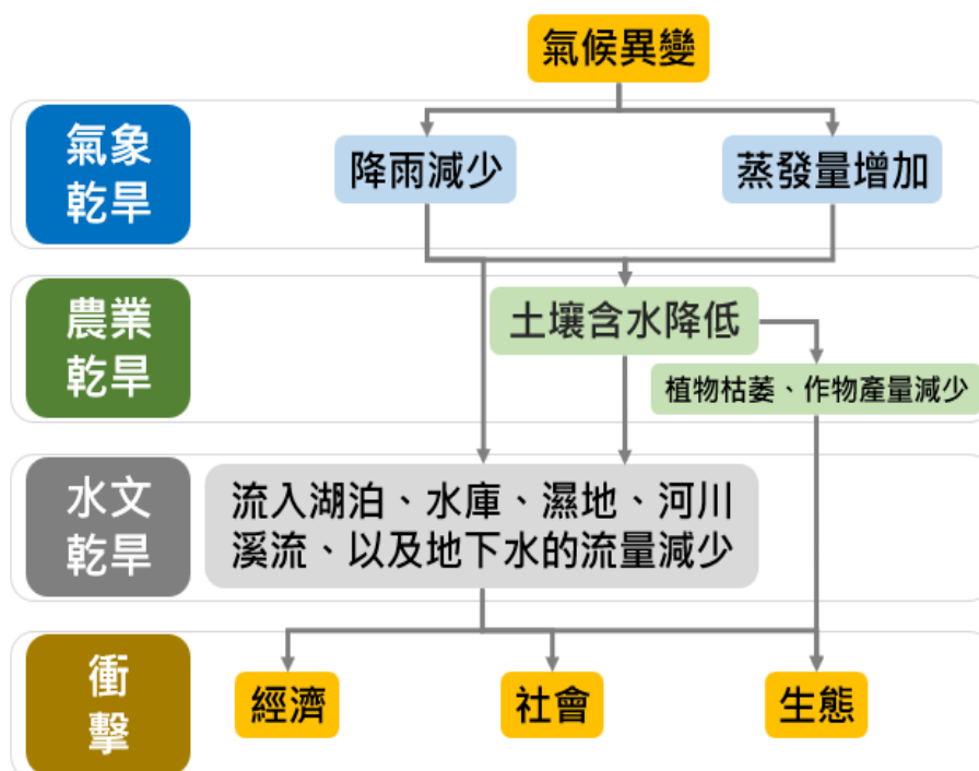
圖 25 不同乾旱類型之相互關係及衝擊
