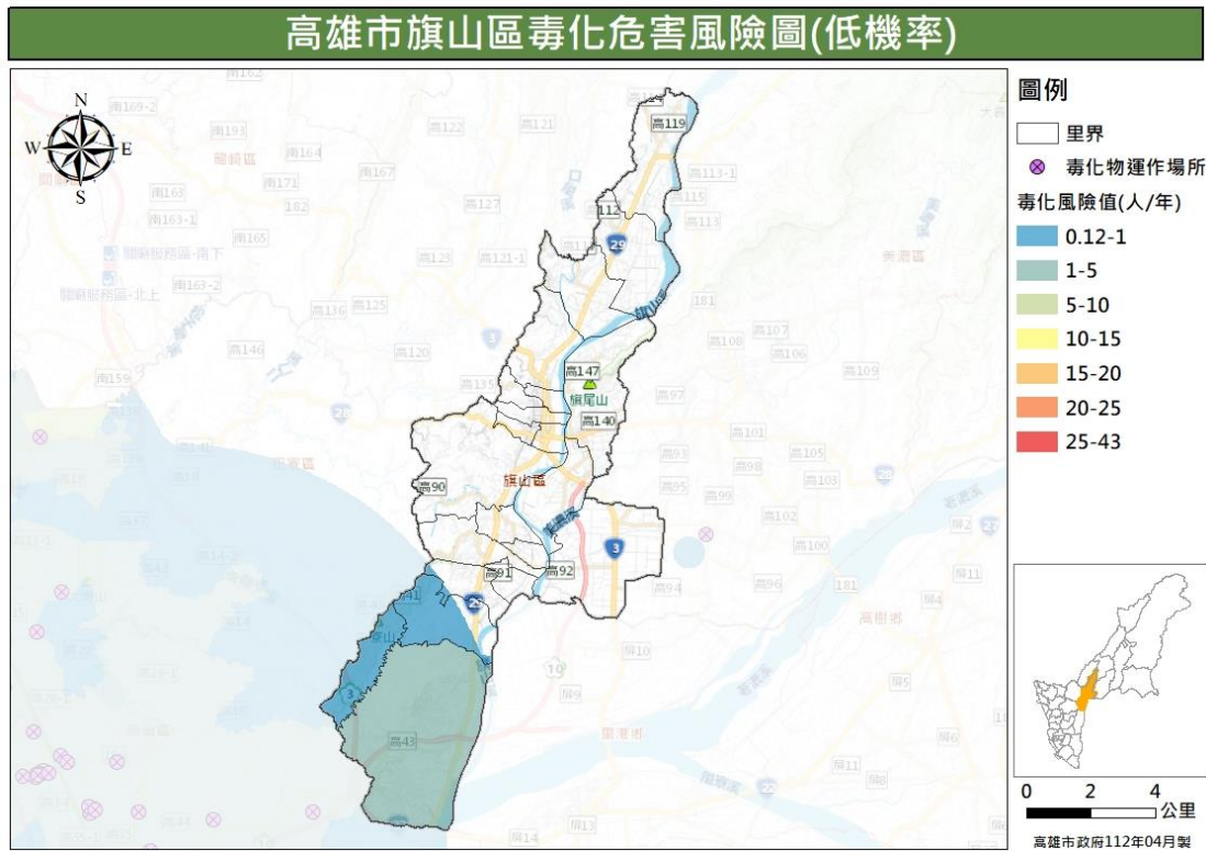
圖 30 旗山區毒性化學物質災害危害風險潛勢圖（低機率）
