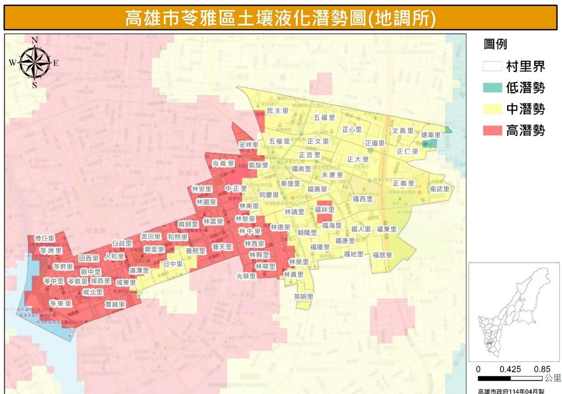
圖 24 苓雅區土壤液化潛勢圖 (資料來源：地質調查及礦業管理中心)
