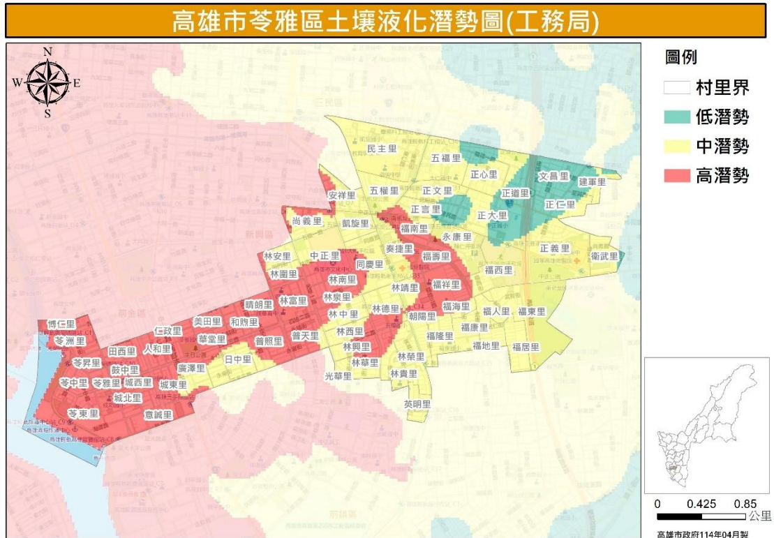
圖 25 苓雅區土壤液化潛勢圖 (資料來源：高雄市政府工務局)
