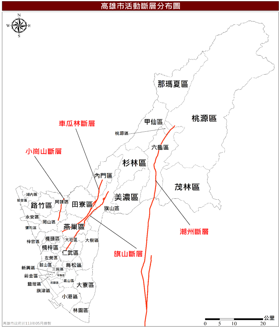
圖 9 高雄市境內與鄰近地區斷層分布圖
