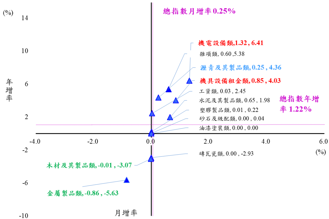
圖3、114年1月高雄市營造工程物價指數月增率及年增率
